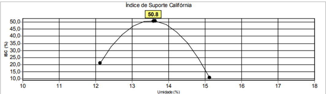
Gráfico 17 – Curva de ISC da mistura 4.
