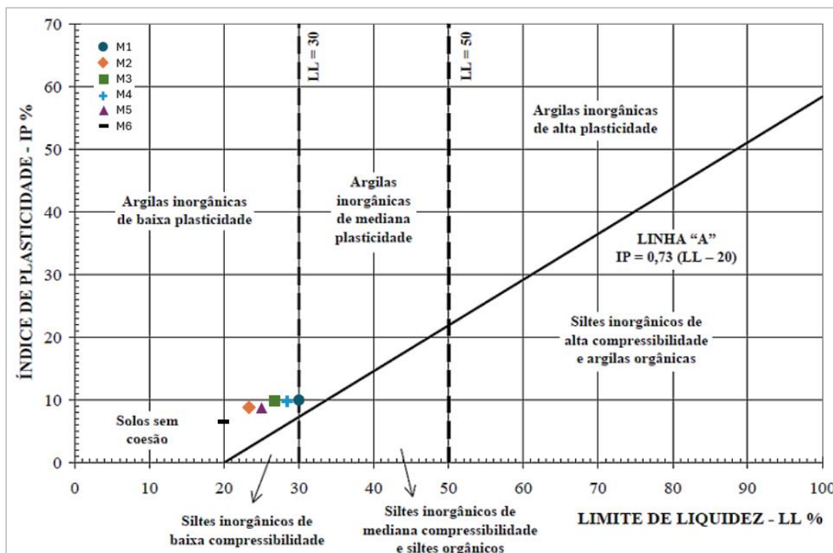
Figura 38 – Gráfico índice de plasticidade x limite de liquidez das misturas e solo coletado.
