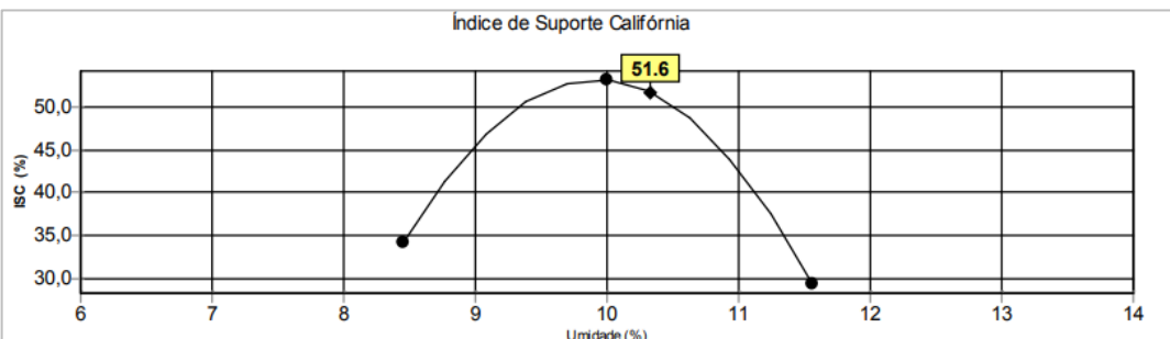
Gráfico 19 – Curva de ISC da mistura 6.
