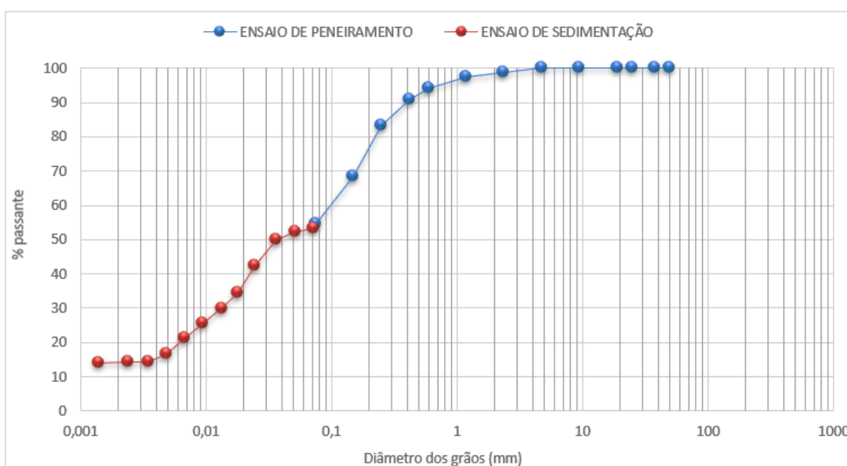
Gráfico 2 –Curva granulométrica obtida do solo coletado
