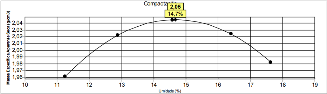
Gráfico 9 – Curva de compactação da mistura 2.
