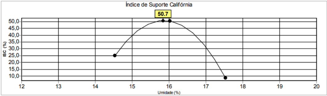
Gráfico 14 – Curva de ISC da mistura 1.
