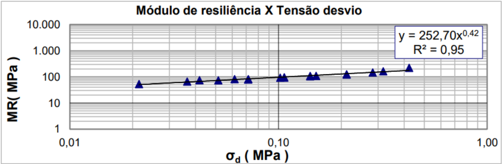
Gráfico 28 – Módulo de resiliência x Tensão desvio da mistura 3.
