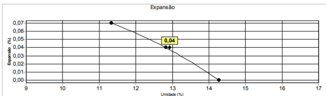
Gráfico 24 – Expansão da mistura 5.
