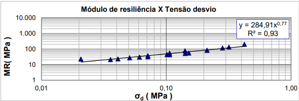
Gráfico 26 – Módulo de resiliência x Tensão desvio da mistura 1.
