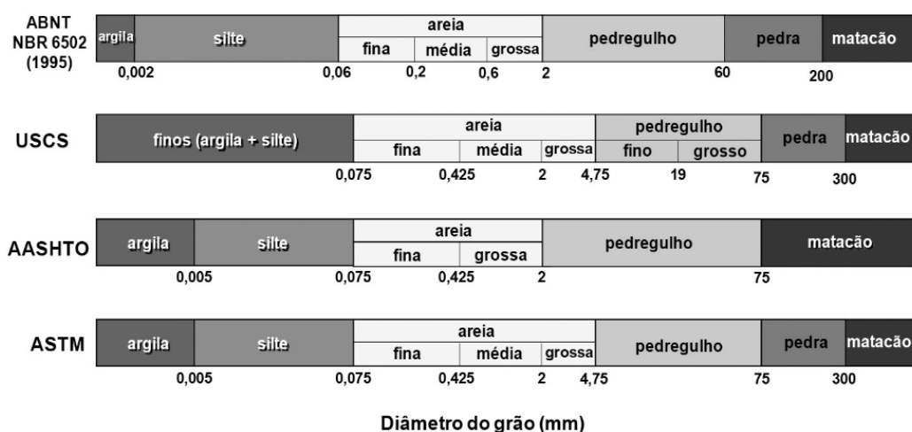
Figura 5 – Escala granulométrica de solos conforme normas técnicas aplicáveis
