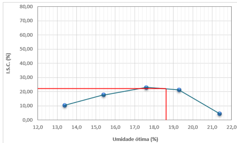
Gráfico 6 – Resultado Índice de Suporte Califórnia do solo coletado.
