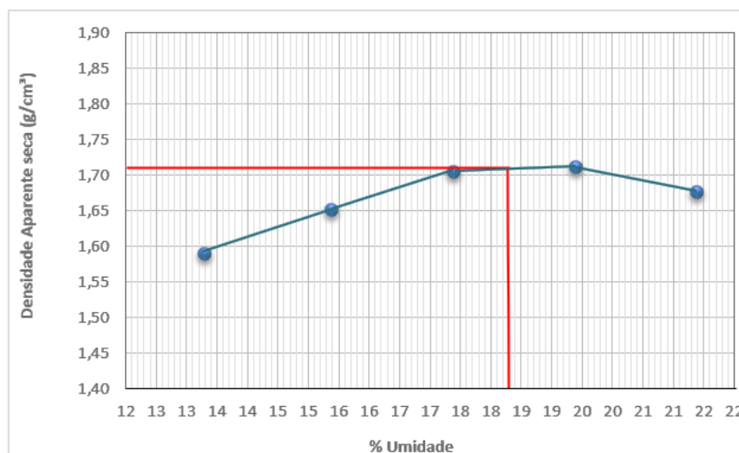
Gráfico 3 – Curva de compactação - massa específica do solo
