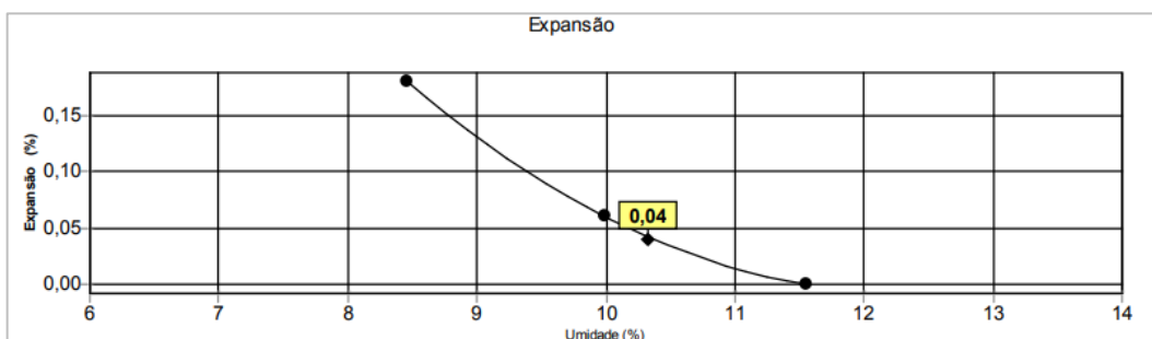
Gráfico 25 – Expansão da mistura 6.
