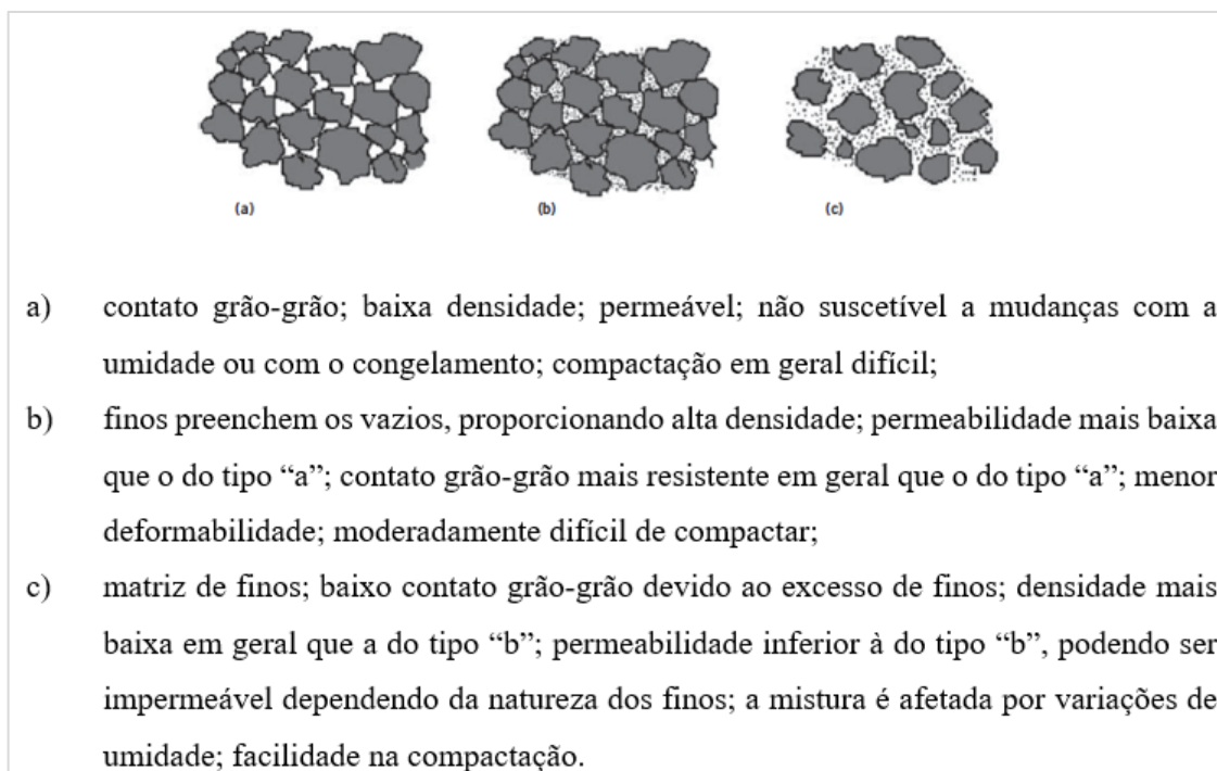
Figura 12 – Subdivisão dos solos-agregados em relação a finura e interação dos grãos
