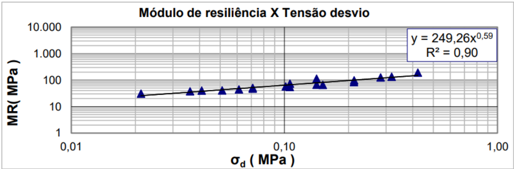
Gráfico 27 – Módulo de resiliência x Tensão desvio da mistura 2.
