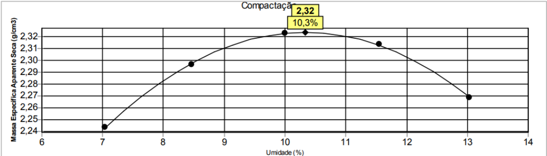
Gráfico 13 – Curva de compactação da mistura 6.
