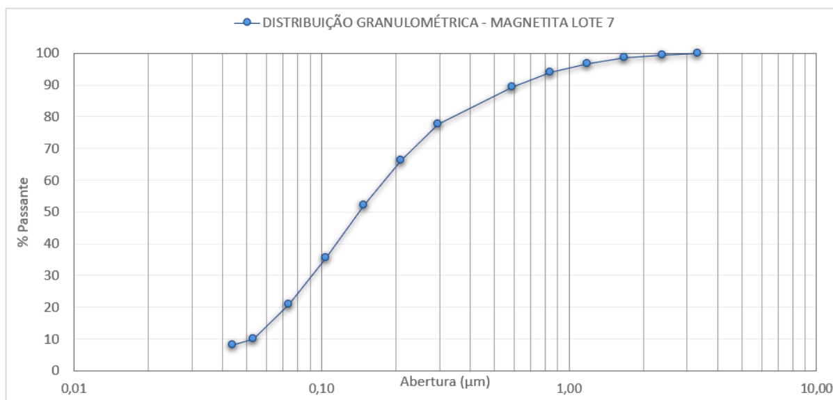
Gráfico 1 – Distribuição granulométrica do rejeito magnetita
