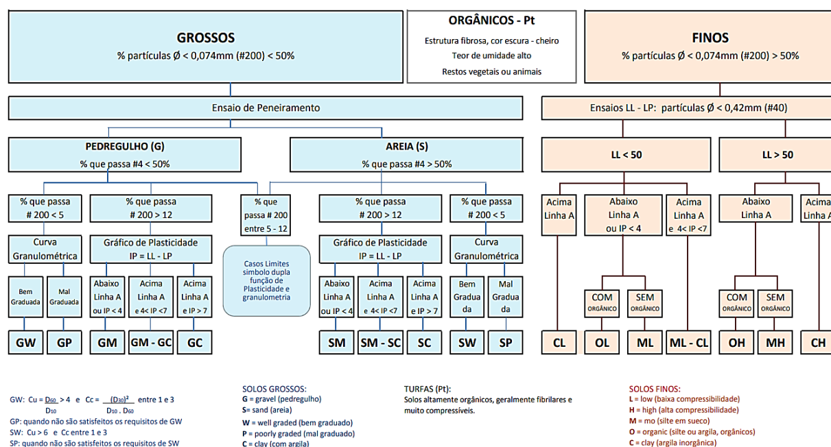
Figura 7 – SUCS – Sistema Unificado de Classificação de Solos
