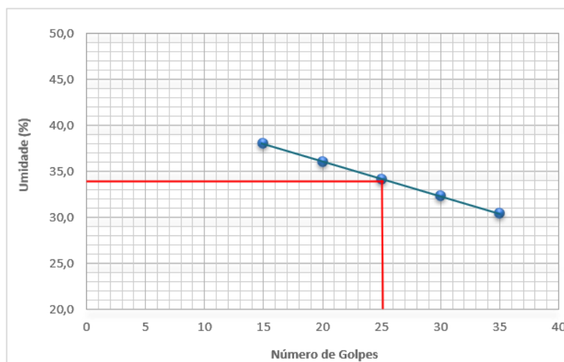
Gráfico 4 – Limite de liquidez do solo
