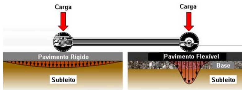
Figura 4 – Representação da distribuição das cargas nos pavimentos
