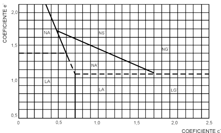
Figura 8 – Ábaco de classificação MCT
