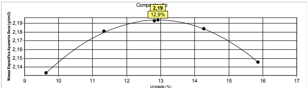
Gráfico 12 – Curva de compactação da mistura 5.
