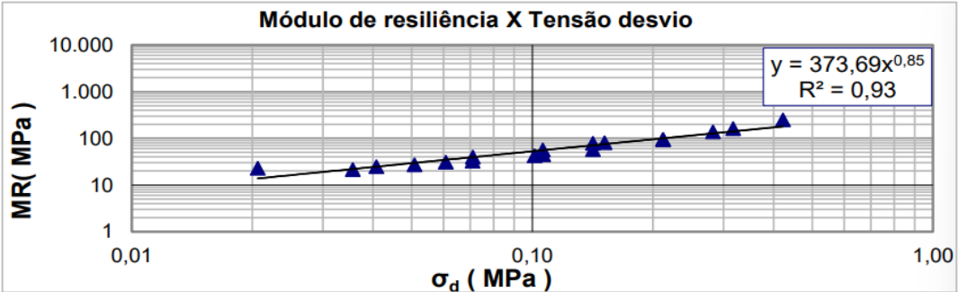
Gráfico 29 – Módulo de resiliência x Tensão desvio da mistura 4.
