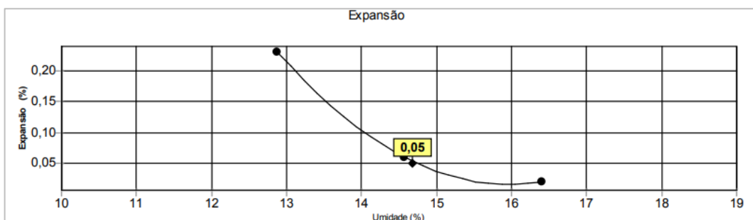
Gráfico 21 – Expansão da mistura 2.
