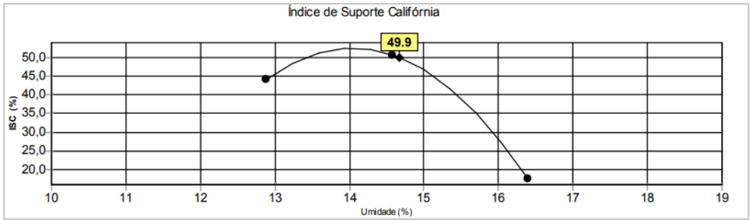
Gráfico 15 – Curva de ISC da mistura 2.
