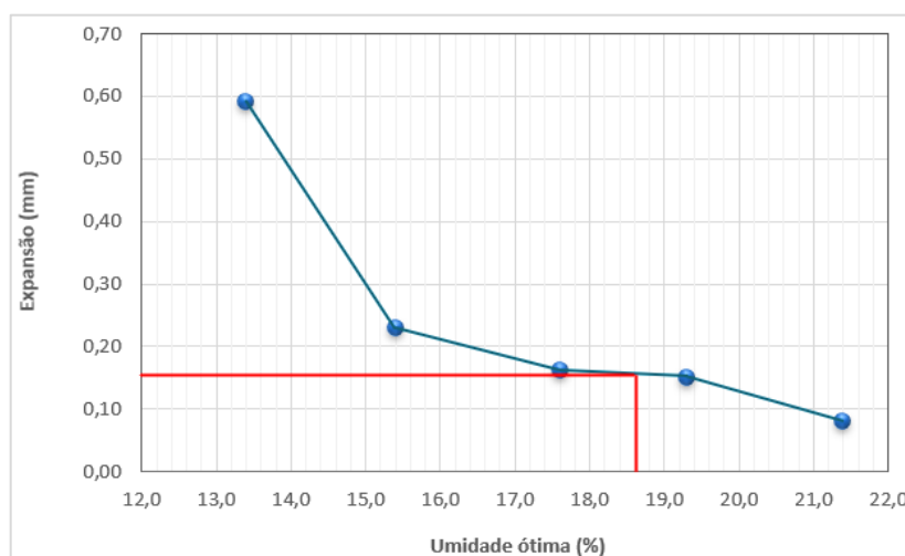
Gráfico 5 – Resultado percentual de Expansão do solo coletado
