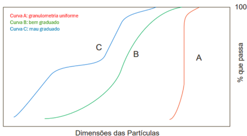
Figura 31 – Tipos de faixas granulométricas conforme graduação das partículas.
