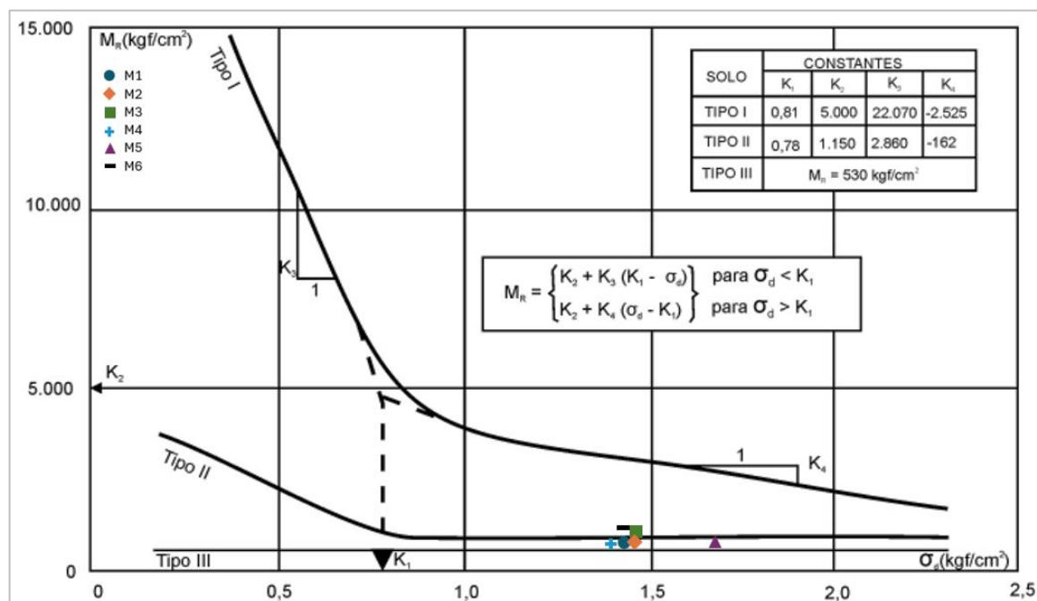
Figura 39 – Classificação resiliente de solos finos
