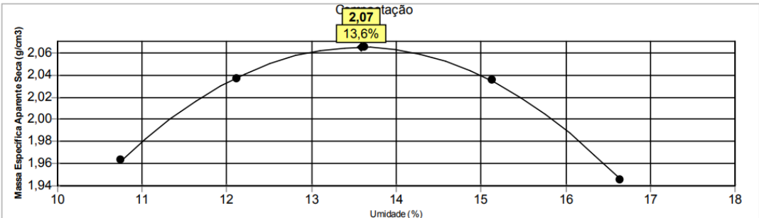
Gráfico 11 – Curva de compactação da mistura 4.
