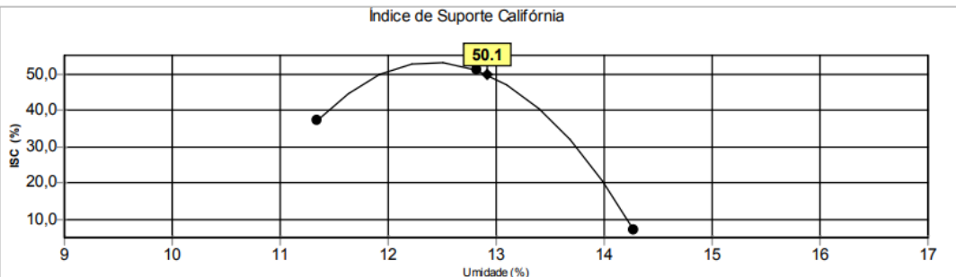
Gráfico 18 – Curva de ISC da mistura 5.
