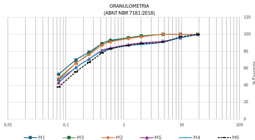
Gráfico 7 – Curva granulométrica das misturas
