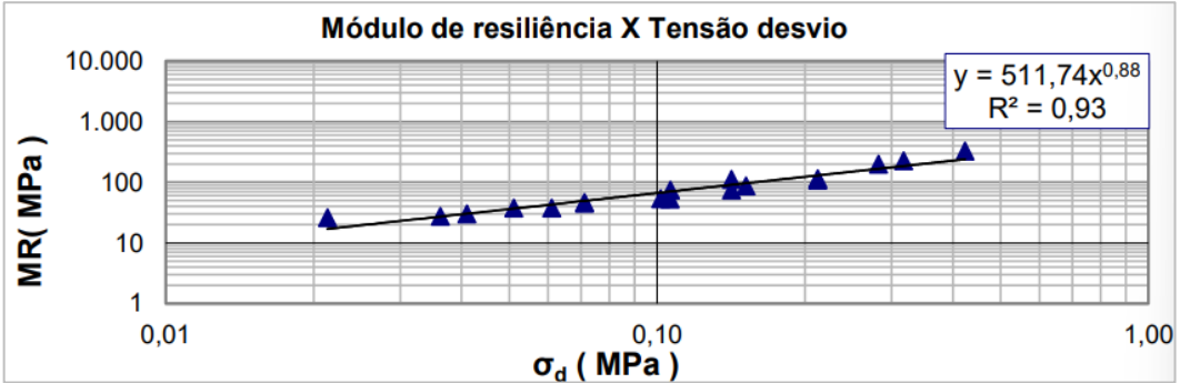
Gráfico 31 – Módulo de resiliência x Tensão desvio da mistura 6.
