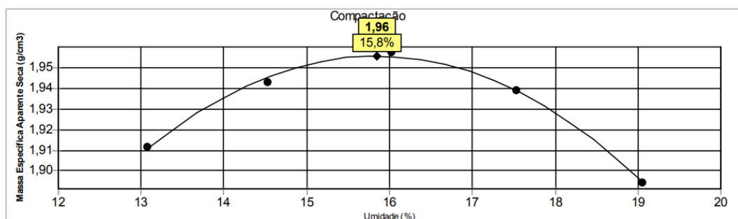
Gráfico 8 – Curva de compactação da mistura 1.
