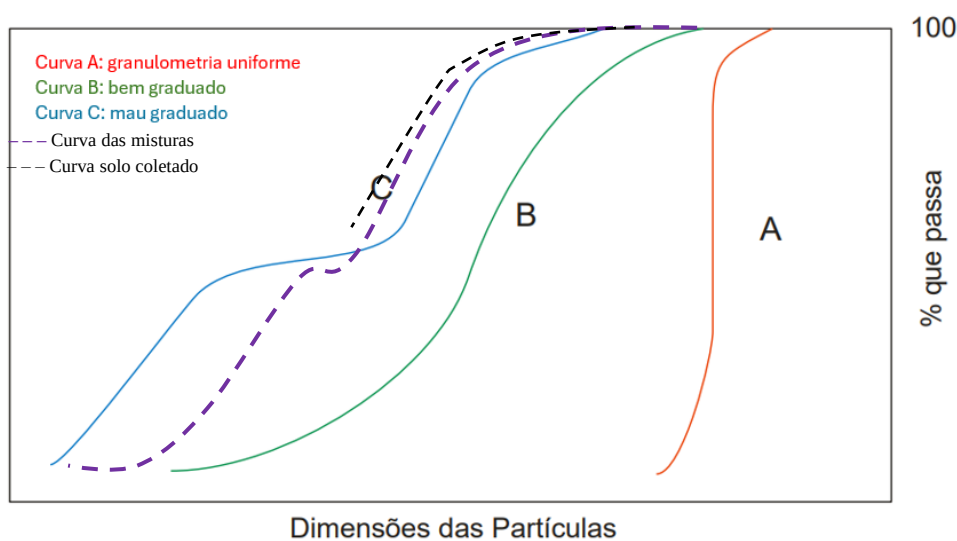
Figura 37 – Classificação do solo em função da curva granulométrica
