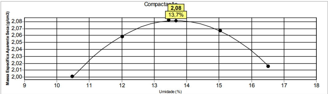
Gráfico 10 – Curva de compactação da mistura 3.
