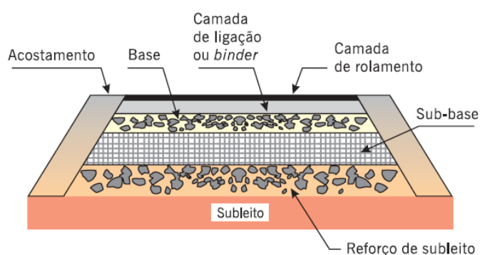
Figura 3 – Esquema da seção transversal do pavimento
