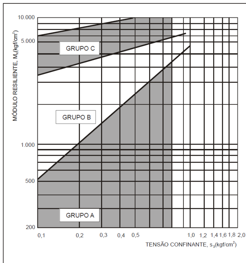
Figura 10 – Classificação resiliente de solos granulares
