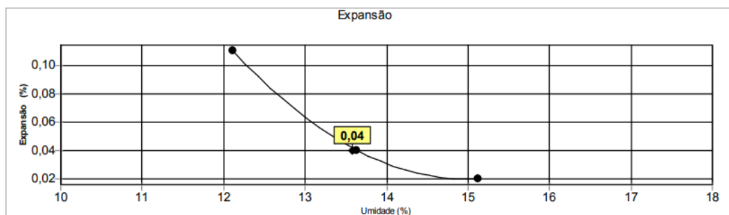
Gráfico 23 – Expansão da mistura 4.
