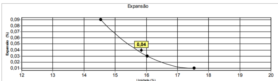
Gráfico 20 – Expansão da mistura 1.
