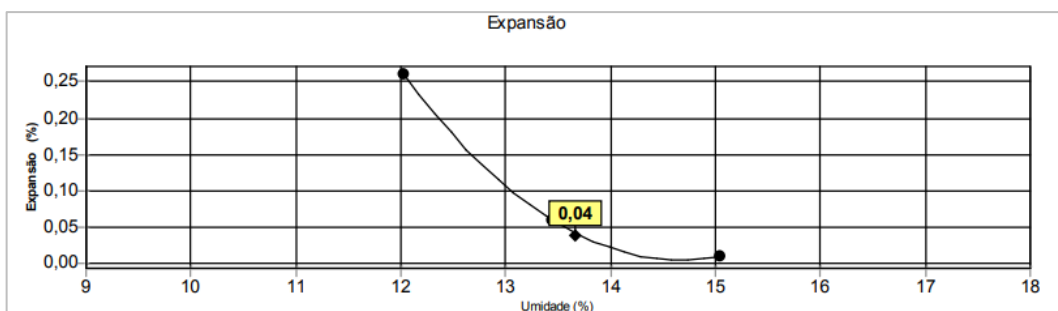
Gráfico 22 – Expansão da mistura 3.
