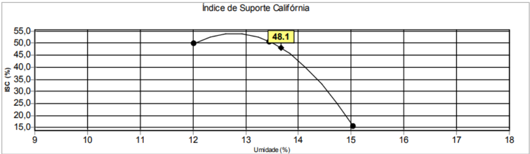
Gráfico 16 – Curva de ISC da mistura 3.
