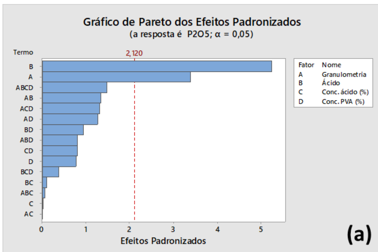
Figura 48 - Teor de P_2O_5 Planejamento Fatorial 2^4 (a) Gráfico de Pareto; (b) Gráfico Normal; (c) Gráfico de Efeitos Principais
