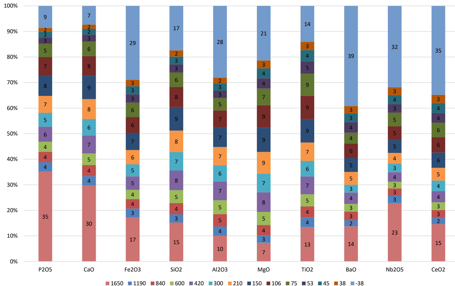
Figura 20 - Distribuição de teores da amostra britada de minério fosfático por faixa granulométrica em micrometros
