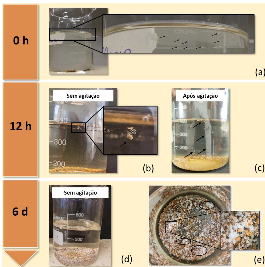
Figura 27 - Evolução da flotação reativa para a faixa -10# +20# (a) Após 0 hora; (b) Após 12 horas sem agitação; (c) Após 12 horas com agitação; (d) Após 6 dias sem agitação; (e) Dissolução dos carbonatos após 6 dias
