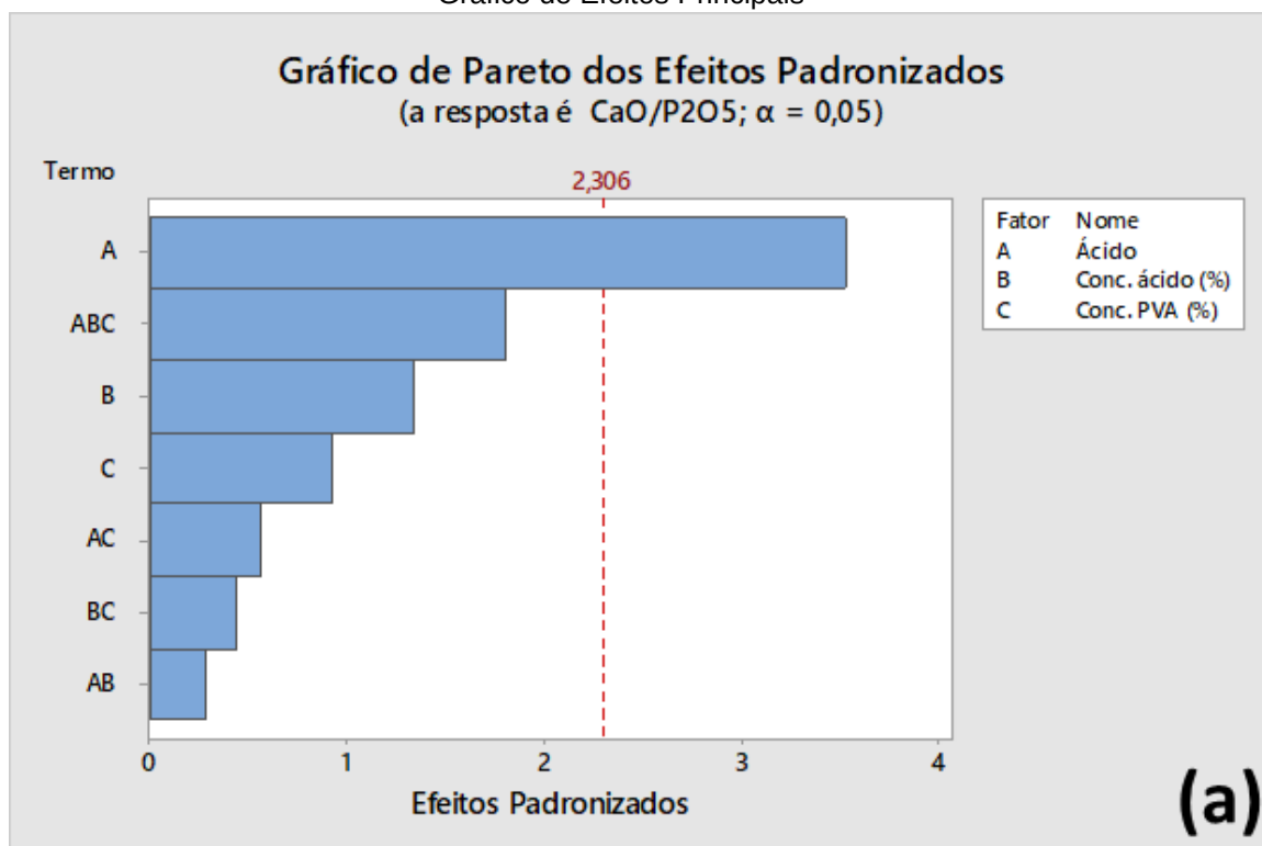
Figura 57 - Relação CaO/ P 2 O 5 Planejamento Fatorial 2 3 (a) Gráfico de Pareto;(b) Gráfico Normal; (c) Gráfico de Efeitos Principais
