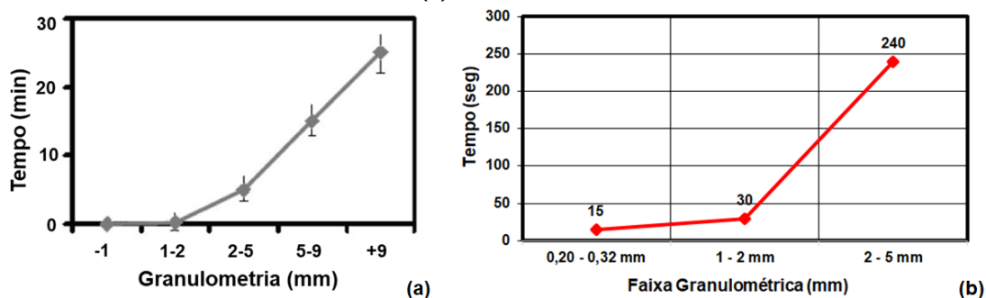
Figura 6 - Tempo necessário para flotar partículas de diferentes frações granulométricas (a) Faixa de -1 a +9 mm; (b) Faixa de 0,20 – 0,32 mm a 2-5 mm
