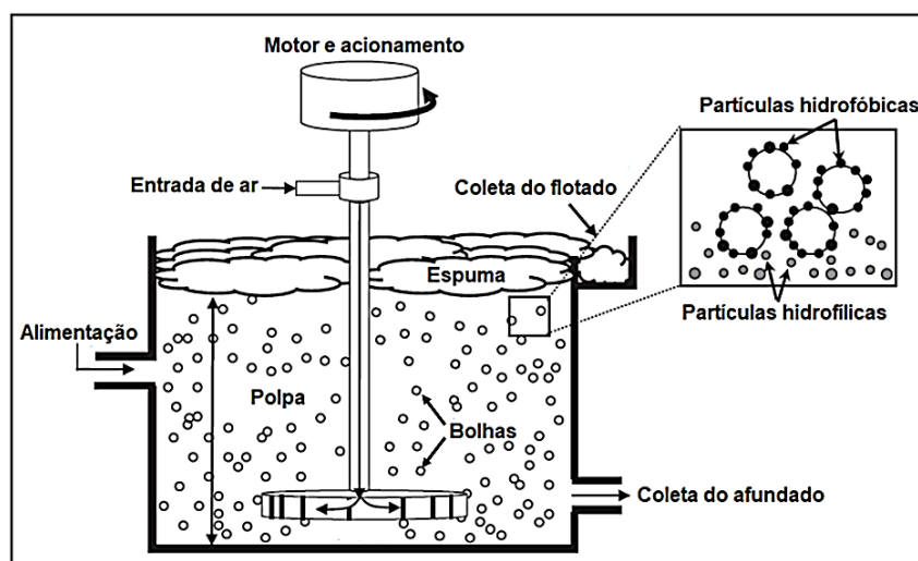
Figura 2 - Sistema de flotação
