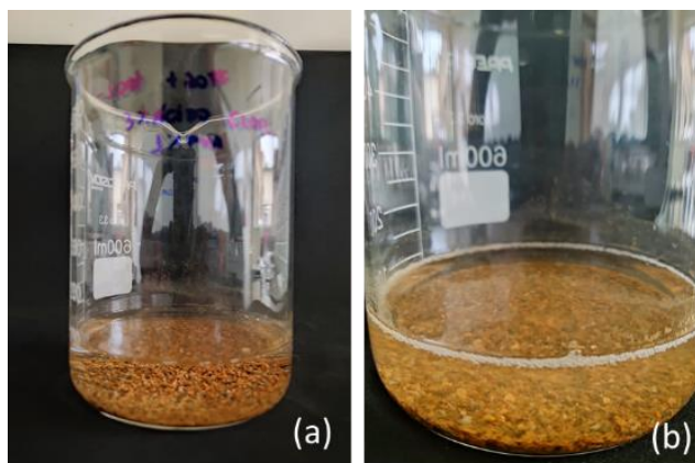
Figura 40 - Evolução da flotação com ácido cloroacético (a) -10# +20# após 72 horas sem agitação; (b) -10# +20# após 72 horas com agitação
