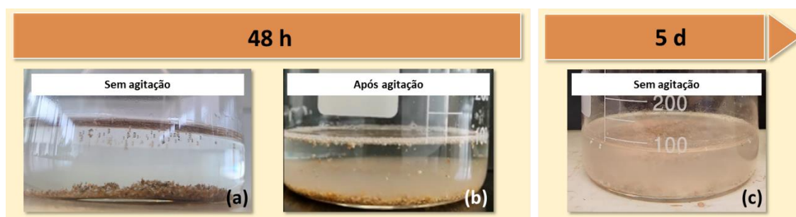
Figura 34 - Evolução da flotação reativa para a faixa -20# +65# para 100 ml de \text{H}_2\text{SO}_4 3% (v/v) e PVA 3% (m/v) (a) Após 48 h sem agitação; (b) Após 48 horas com agitação; (c) Após 5 dias
