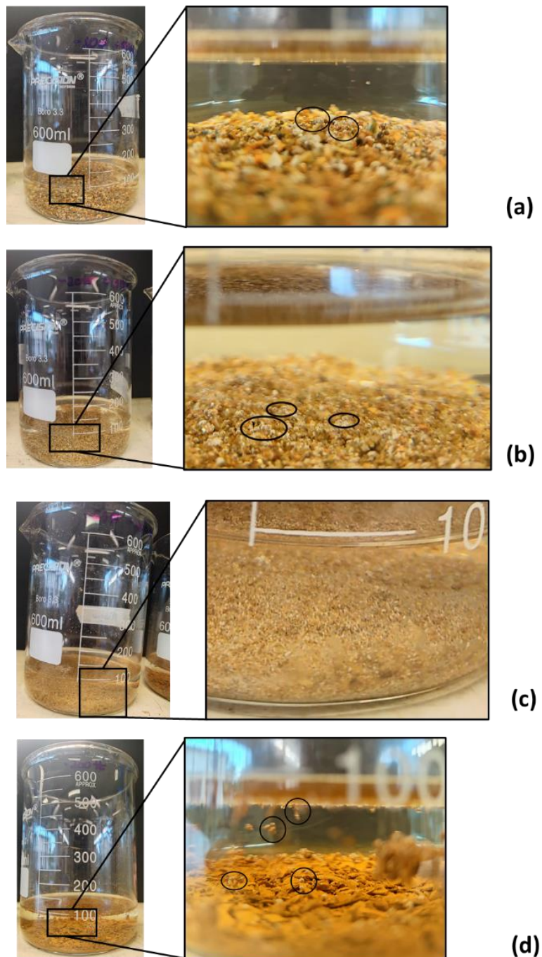
Figura 37 - Flotação reativa após 24 horas com prévia secagem do PVA (a) -10# +20#; (b) -20# +65#; (c) -65# +200#; (d) -200#
