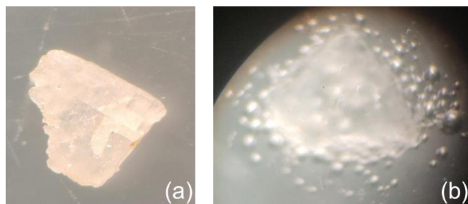
Figura 26 - Calcita presente na faixa -1,70 mm +0,84 mm (a) Calcita antes da reação com ácido clorídrico; (b) Reação entre calcita e ácido clorídrico
