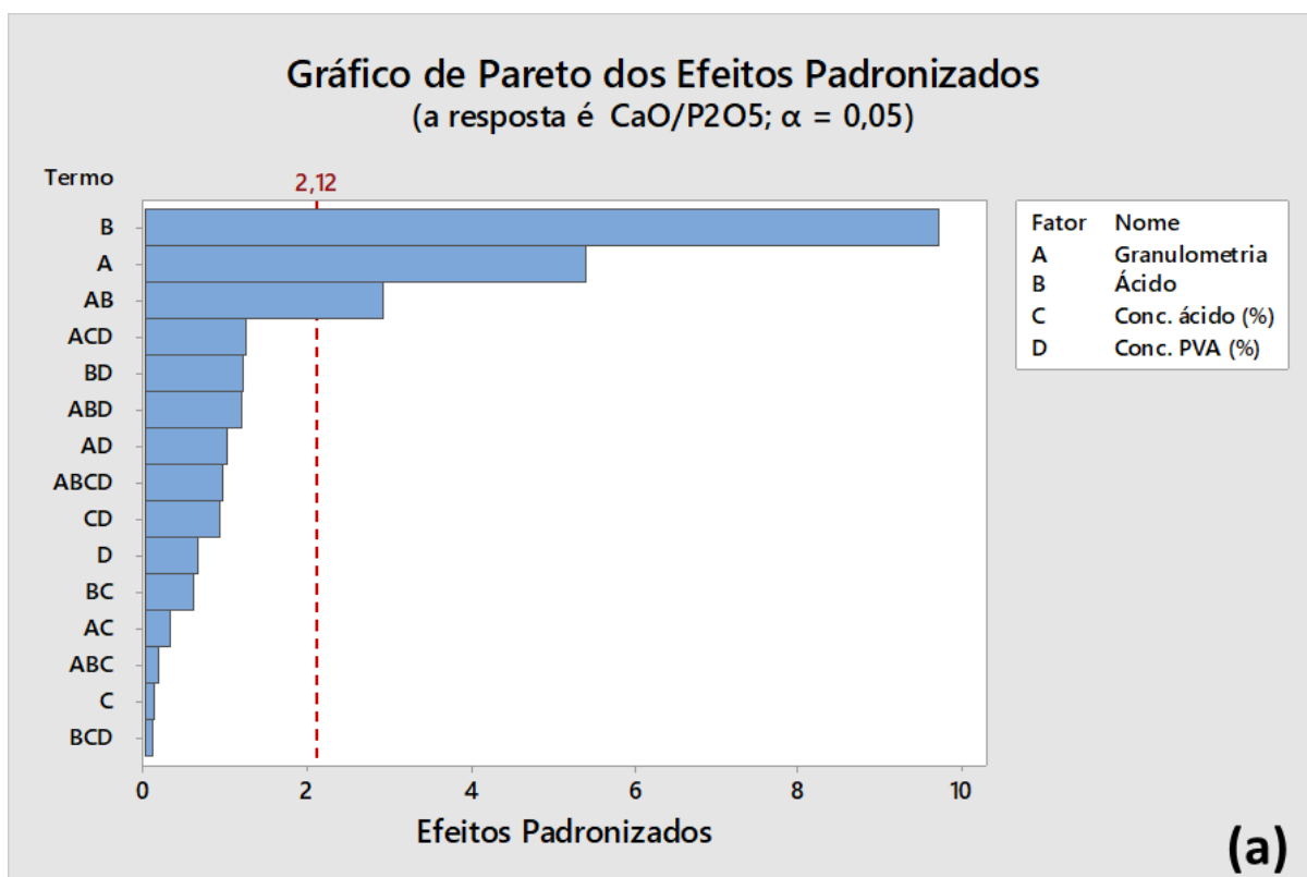
Figura 51 - Teor de CaO/ P 2 O 5 Planejamento Fatorial 2 4 (a) Gráfico de Pareto;(b) Gráfico Normal
