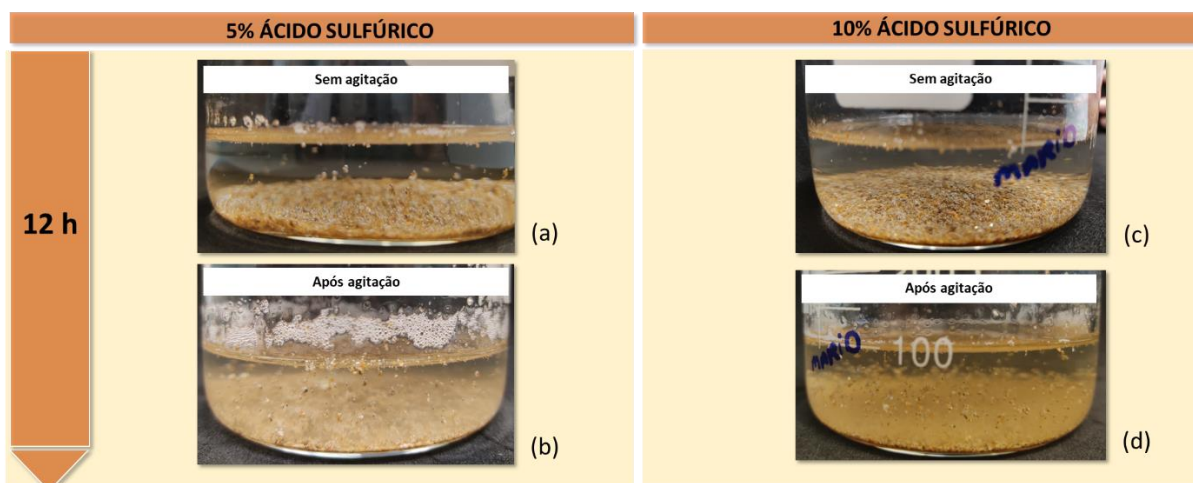
Figura 43 - Avaliação das concentrações de 5 e 10% (v/v) de ácido sulfúrico para a faixa -20# +65# (a) 5% (v/v) \text{H}_2\text{SO}_4 após 12 h sem agitação; (b) 5% (v/v) \text{H}_2\text{SO}_4 após 12 h com agitação; (c) 10% (v/v) \text{H}_2\text{SO}_4 após 12 h sem agitação; (d) 10% (v/v) \text{H}_2\text{SO}_4 após 12 h com agitação.
