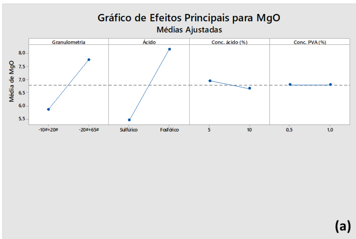
Figura 50 - Teor de MgO Planejamento Fatorial 2^4 (a) Gráfico de Efeitos Principais; (b) Gráfico de Interação
