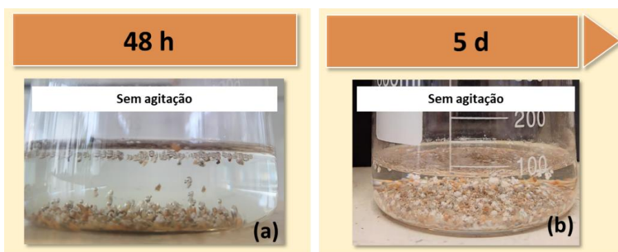
Figura 32 - Evolução da flotação reativa para a faixa -10# +20# para 100 ml de \text{H}_2\text{SO}_4 3% (v/v) e PVA 3% (m/v) (a) Após 48 h; (b) Após 5 dias
