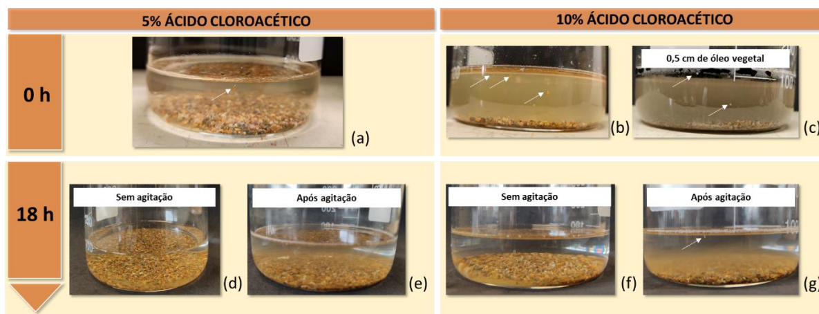
Figura 42 - Avaliação das concentrações de 5 e 10% (m/v) de ácido cloroacético para a faixa -10# +20# (a) 5% (m/v) ácido cloroacético após 0 h; (b) 10% (m/v) ácido cloroacético após 0 h; (c) 10% (m/v) ácido cloroacético após 0 h com 0,5 cm de óleo vegetal; (d) 5% (m/v) ácido cloroacético após 18 h sem agitação; (e) 5% (m/v) ácido cloroacético após 18 h com agitação; (f) 10% (m/v) ácido cloroacético após 18 h sem agitação; (g) 10% (m/v) ácido cloroacético após 18 h com agitação.
