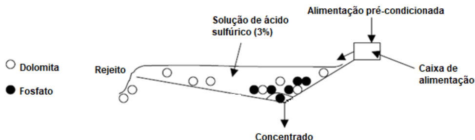
Figura 8 - Representação do processo de flotação reativa empregando calha
