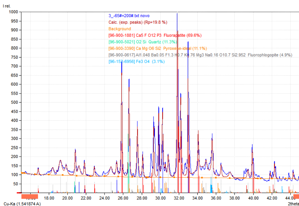
Figura 23 - Difratoograma da fração -65# +200#
