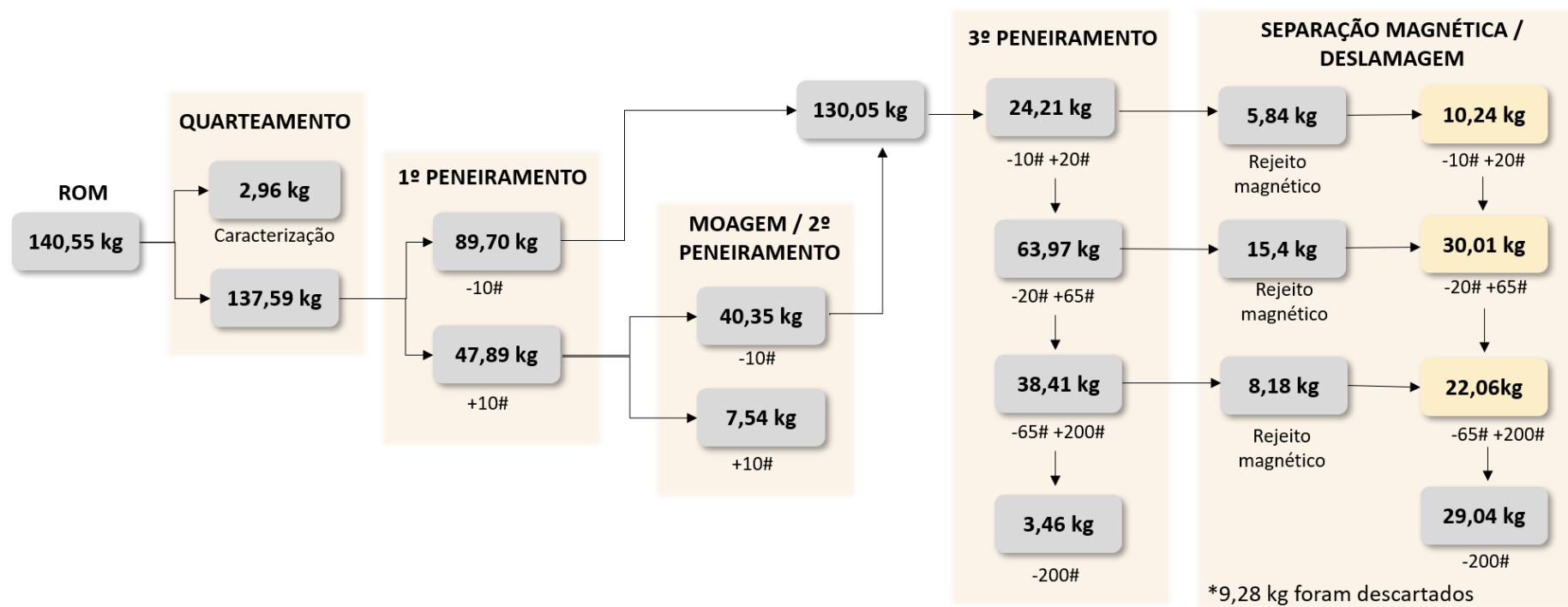
Figura 17 - Balanço de massa
