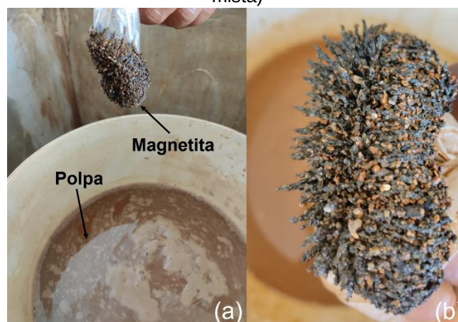
Figura 16 - Separação Magnética (a) Produtos; (b) Rejeito Magnético (Partículas de magnetita mista)
