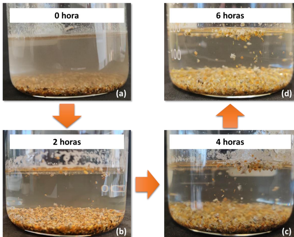
Figura 46 - Flotação ao longo de 6 horas empregando 200 ml de \text{H}_2\text{SO}_4 10% (v/v) e 1% (m/v) de PVA (a) Após 0 h; (b) Após 2 h; (c) Após 4 h; (d) Após 6 h
