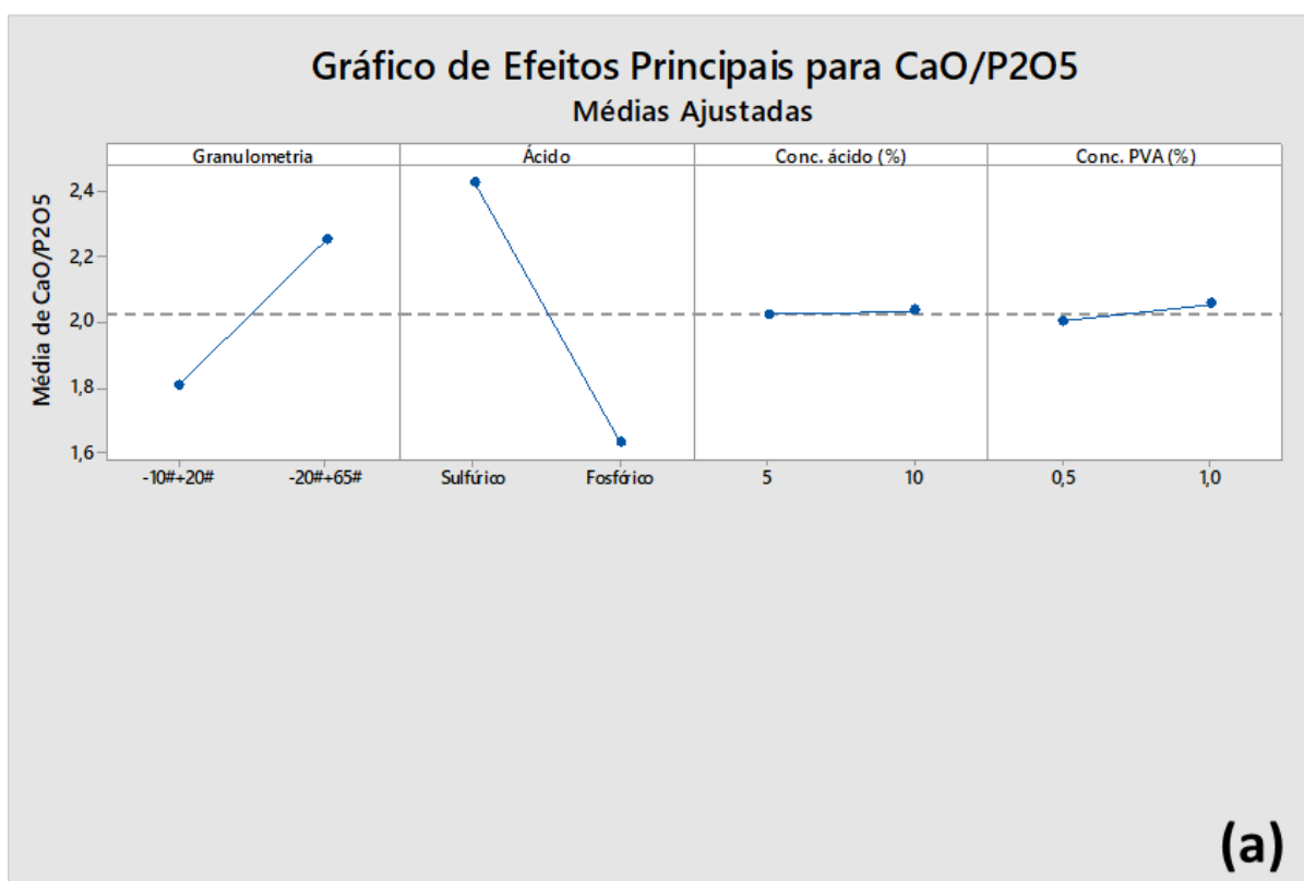
Figura 52 - Teor de \text{MgO} Planejamento Fatorial 2^4 (a) Gráfico de Efeitos Principais; (b) Gráfico de Interação
