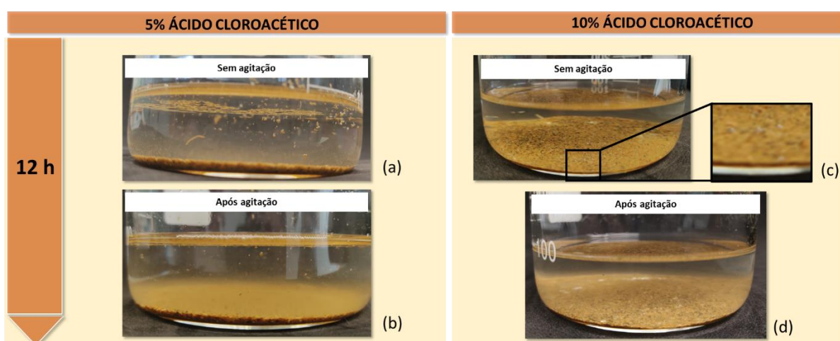
Figura 44 - Avaliação das concentrações de 5 e 10% (m/v) de ácido cloroacético para a faixa -20# +65# (a) 5% (m/v) ácido cloroacético após 12 h sem agitação; (b) 5% (m/v) ácido cloroacético após 12 h com agitação; (c) 10% (m/v) ácido cloroacético após 12 h sem agitação; (d) 10% (m/v) ácido cloroacético após 12 h com agitação.
