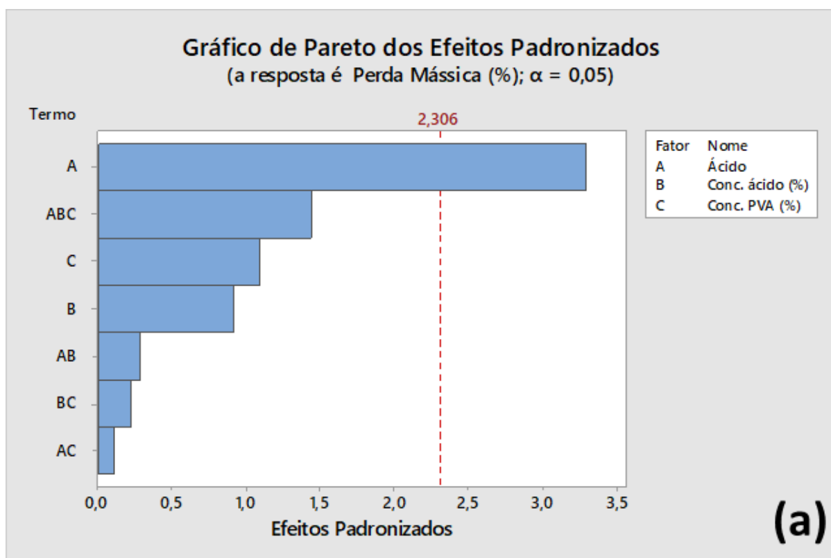
Figura 54 - Perda Mássica Planejamento Fatorial 2^3 (a) Gráfico de Pareto; (b) Gráfico Normal; (c) Gráfico de Efeitos Principais
