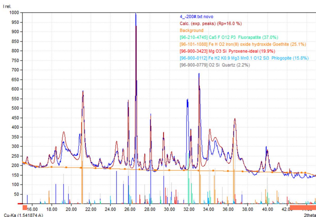
Figura 24 - Difratoograma da fração -200#
