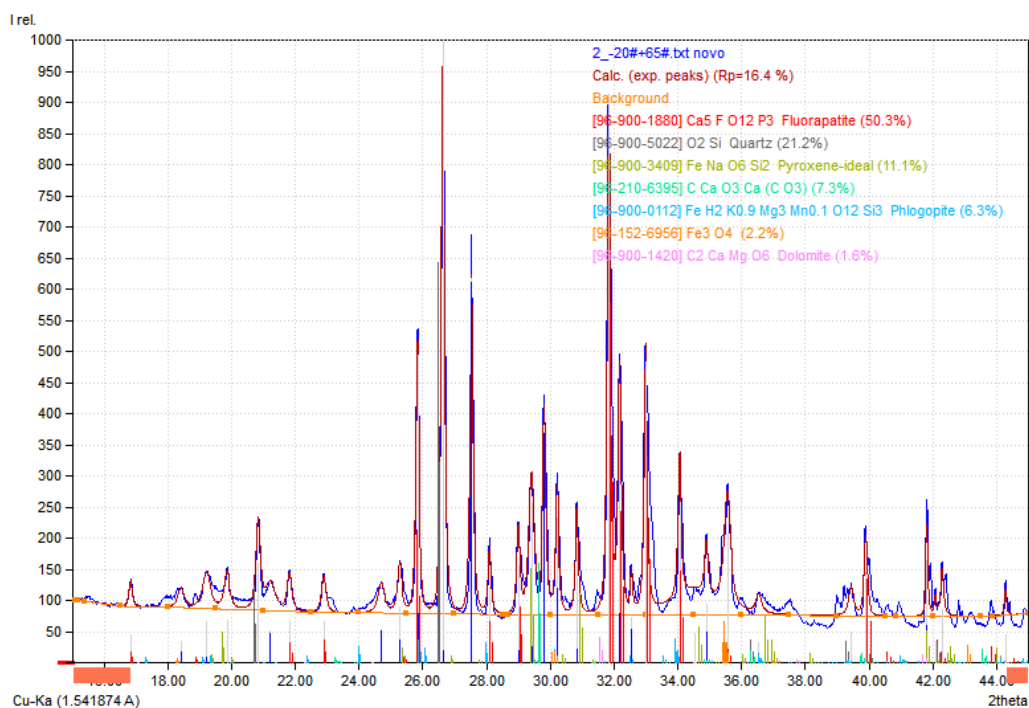
Figura 22 - Difratoograma da fração -20# +65#
