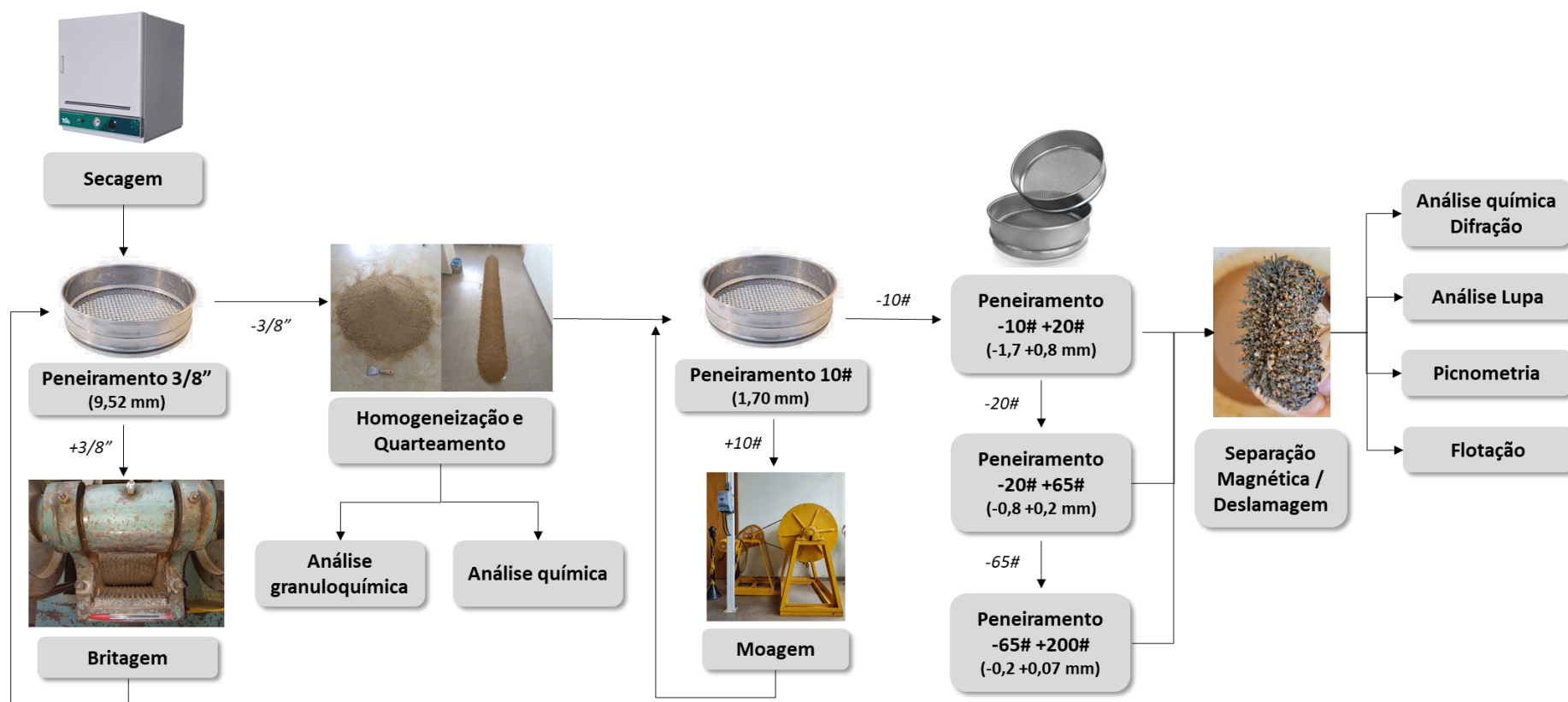
Figura 10 - Fluxograma das etapas de preparação da amostra
