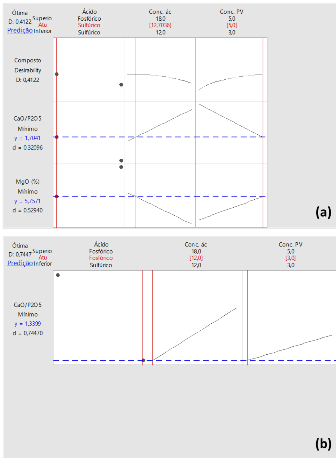
Figura 58 - Otimização de resposta Planejamento Fatorial 2^3 (a) Otimização de CaO/ P_2O_5 e MgO (b) Otimização de CaO/ P_2O_5
