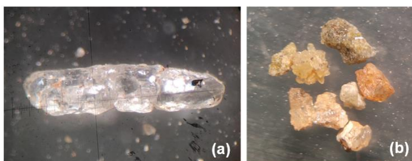
Figura 25 - Apatitas presentes na faixa -1,70 mm +0,84 mm (a) Apatita cristalina; (b) Apatitas recobertas por óxidos e hidróxidos de ferro, e agregado de apatitas
