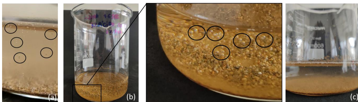
Figura 39 - Evolução da flotação com ácido cloroacético (a) -20# +65# 0 hora; (b) -20# +65# após 72 horas sem agitação; (c) -20# +65# após 72 horas com agitação
