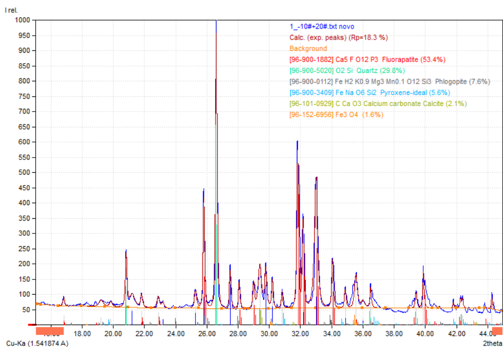
Figura 21 - Difratoograma da fração -10# +20#
