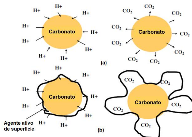
Figura 4 - Interação de carbonatos com o meio ácido (a) sem a recobrimento de um surfactante ou polímero; (b) após recobrimento
