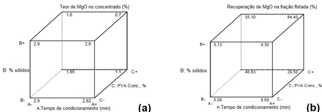
Figura 5 - Gráfico de Cubo (a) Teor de MgO no concentrado; (b) Recuperação de MgO na fração flotada
