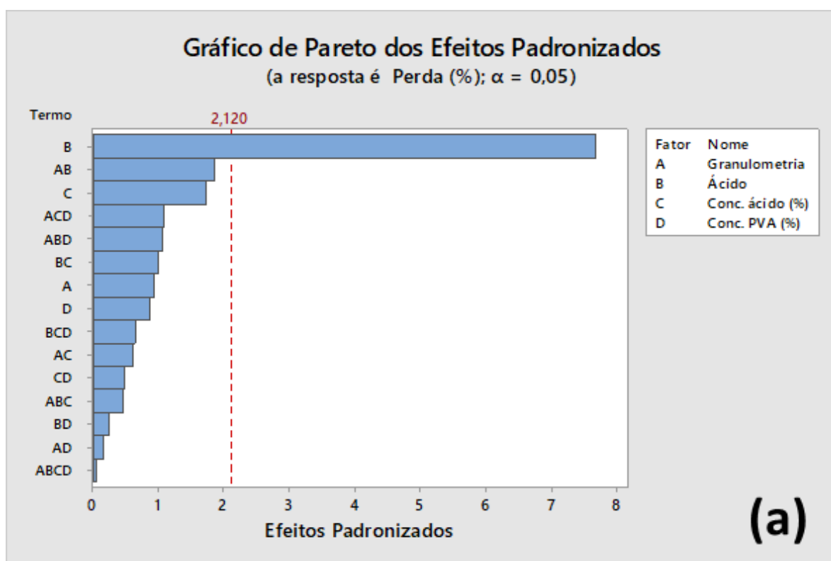
Figura 47 - Perda Mássica Planejamento Fatorial 2 4 (a) Gráfico de Pareto;(b) Gráfico Normal; (c) Gráfico de Efeitos Principais
