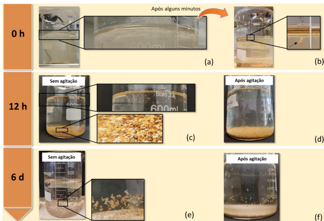
Figura 28 - Evolução da flotação reativa para a faixa -20# +65# (a) Após 0 horas; (b) Após alguns minutos; (c) Após 12 horas sem agitação; (d) Após 12 horas com agitação; (e) Após 6 dias sem agitação; (f) Após 6 dias com agitação
