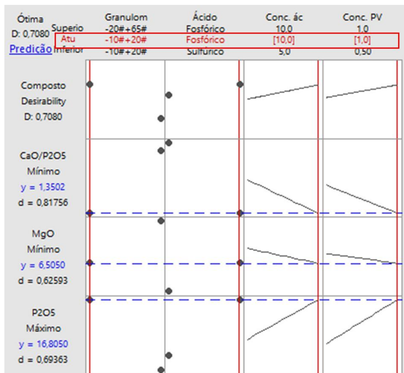
Figura 53 - Gráfico de otimização de resposta para o Planejamento Fatorial 2 4
