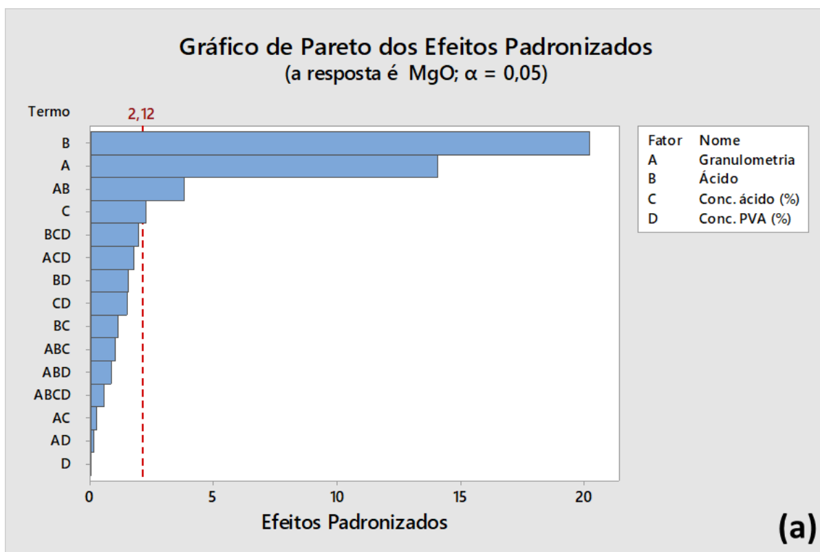
Figura 49 - Teor de MgO Planejamento Fatorial 2^4 (a) Gráfico de Pareto; (b) Gráfico Normal
