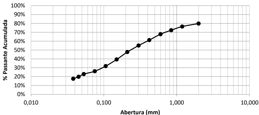
Figura 18 - Curva granulométrica da amostra britada
