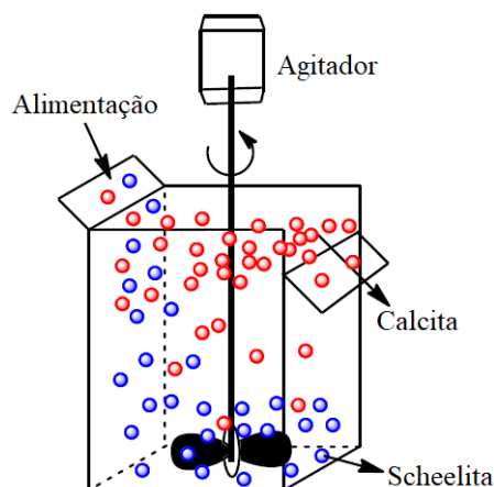
Figura 7 - Máquina de flotação empregada nos testes de flotação reativa
