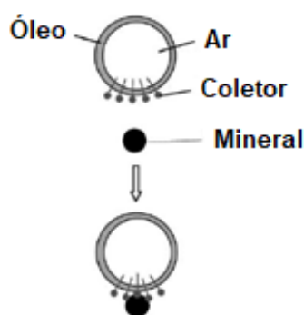
Figura 3 - Flotação empregando bolhas oleosas reativas
