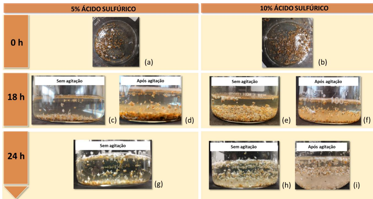
Figura 41- Avaliação das concentrações de ácido sulfúrico para a faixa -10# +20# (a) 5% (v/v) de \text{H}_2\text{SO}_4 após 0 h; (b) 10% (v/v) de \text{H}_2\text{SO}_4 após 0 h; (c) 5% (v/v) de \text{H}_2\text{SO}_4 após 18 h sem agitação; (d) 5% (v/v) de \text{H}_2\text{SO}_4 após 18 h com agitação; (e) 10% (v/v) de \text{H}_2\text{SO}_4 após 18 h sem agitação; (f) 10% (v/v) de \text{H}_2\text{SO}_4 após 18 h com agitação; (g) 5% (v/v) de \text{H}_2\text{SO}_4 após 24 h sem agitação; (h) 10% (v/v) de \text{H}_2\text{SO}_4 após 24 h sem agitação; (i) 10% (v/v) de \text{H}_2\text{SO}_4 após 24 h com agitação.
