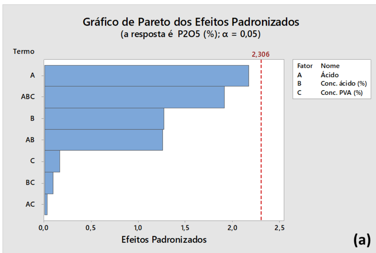
Figura 55 - Teor de \text{P}_2\text{O}_5 Planejamento Fatorial 2^3 (a) Gráfico de Pareto;(b) Gráfico Normal
