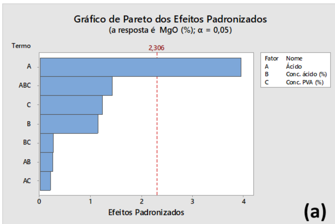
Figura 56 - Teor de MgO Planejamento Fatorial 2^3 (a) Gráfico de Pareto; (b) Gráfico Normal; (c) Gráfico de Efeitos Principais
