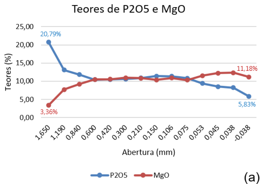
Figura 19 - Análise granulométrica da amostra britada de minério fosfático (a) Teores de P_2O_5 e MgO ; (b) Relação CaO/P_2O_5
