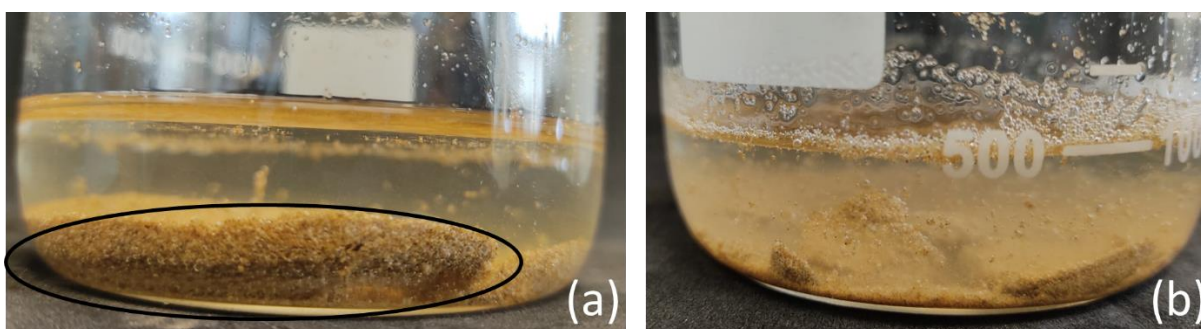
Figura 45 - Flotação reativa da faixa -65# +200# com 10% (v/v) de \text{H}_2\text{SO}_4 após 12 horas (a) Antes da agitação (b) Após agitação
