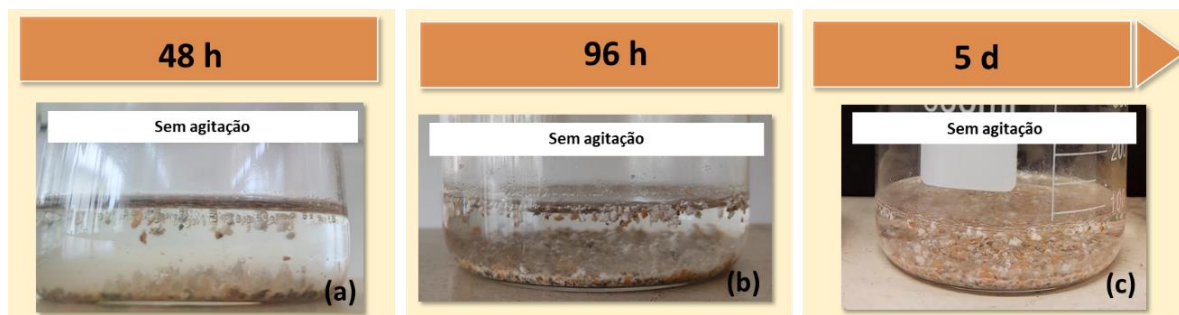
Figura 31 - Evolução da flotação reativa para a faixa -10# +20# para 100 ml de \text{H}_2\text{SO}_4 3% (v/v) e PVA 1% (m/v) (a) Após 48 h; (b) Após 96 h; (c) Após 5 dias
