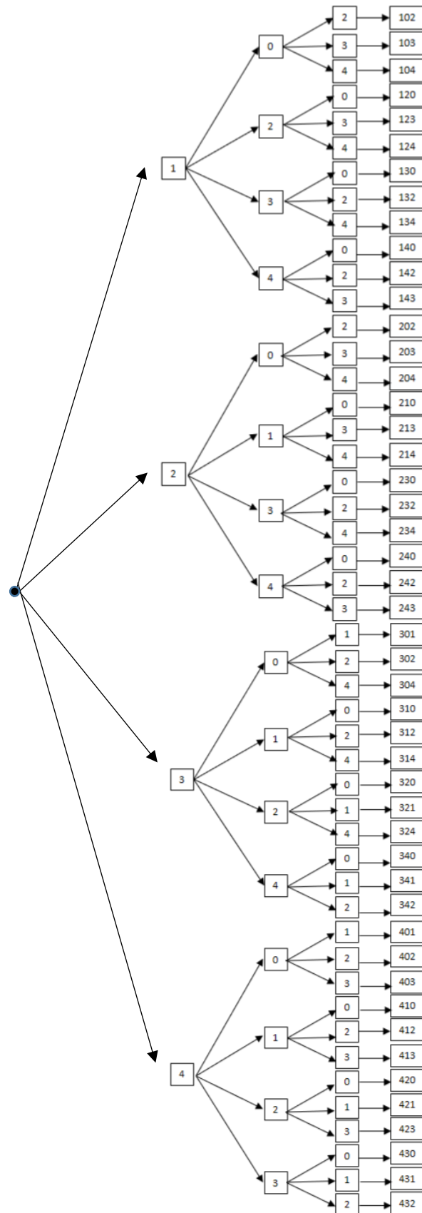
Figura 6.9 – Árvore de decisão do problema 2
