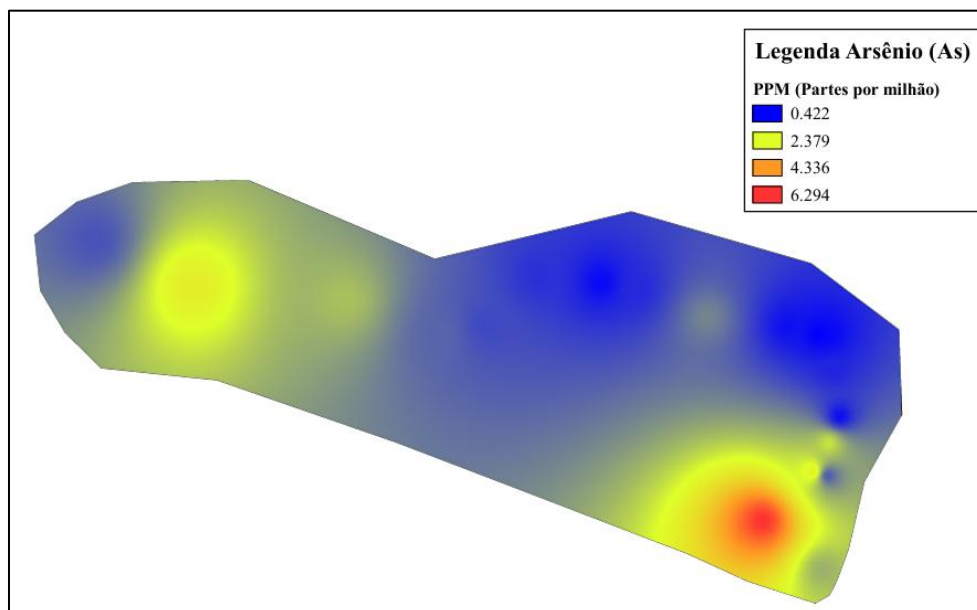
Figura 29 - Isoteores Arsênio
