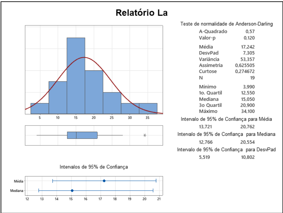
Figura 51 - Sumário gráfico para o lantânio
