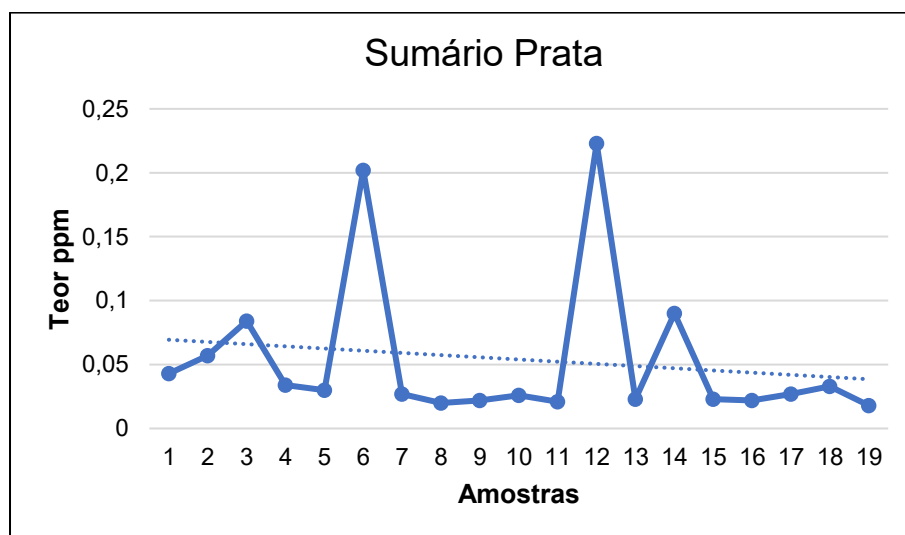
Figura 39 - Distribuição da prata
