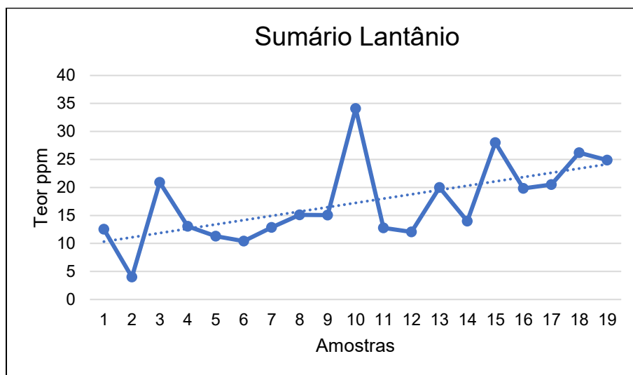
Figura 43 - Distribuição do lantânio
