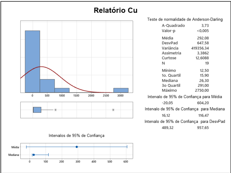
Figura 50 - Sumário gráfico para o cobre
