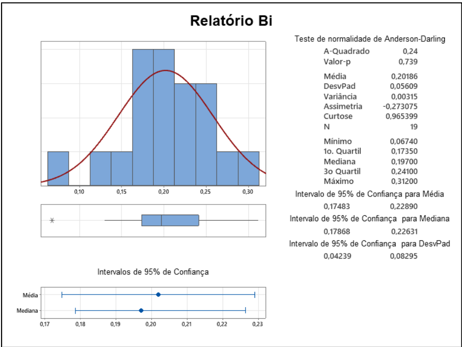
Figura 48 - Sumário gráfico para o bismuto
