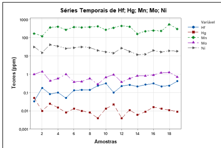
Figura 57 - Curva gráfica metais de transição (ppm)
