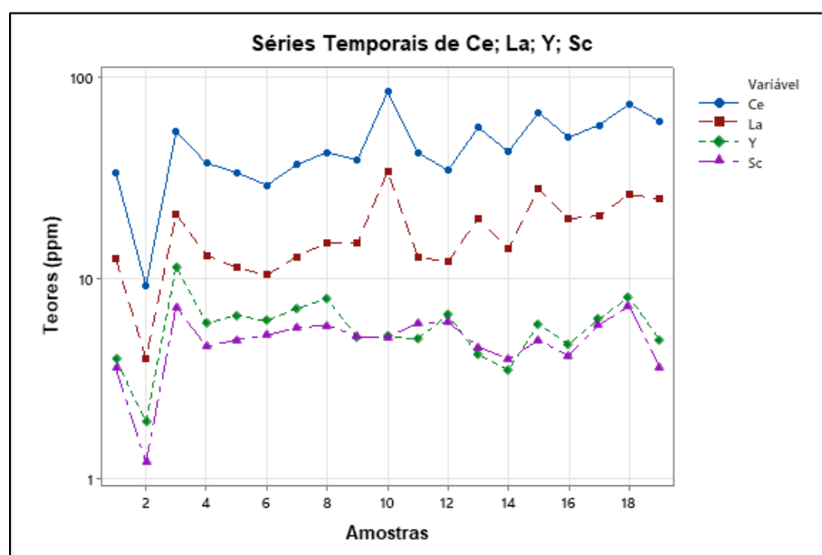
Figura 61 - Série gráfica dos elementos de terras raras
