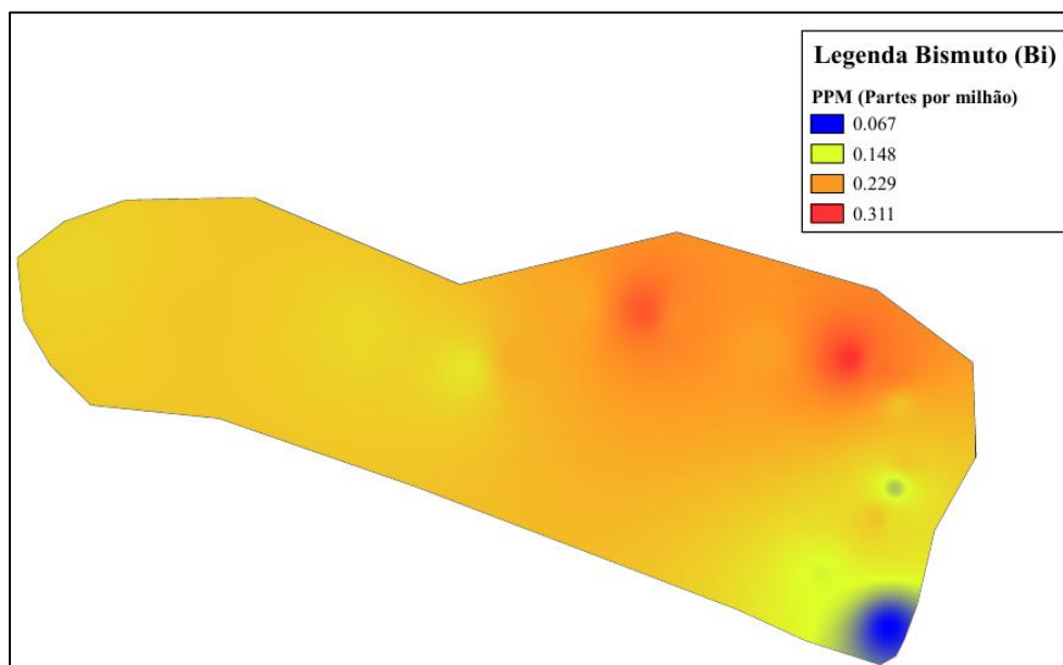
Figura 32 - Isotores Bismuto
