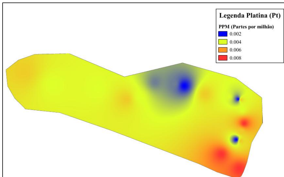
Figura 36 - Isoteores Platina
