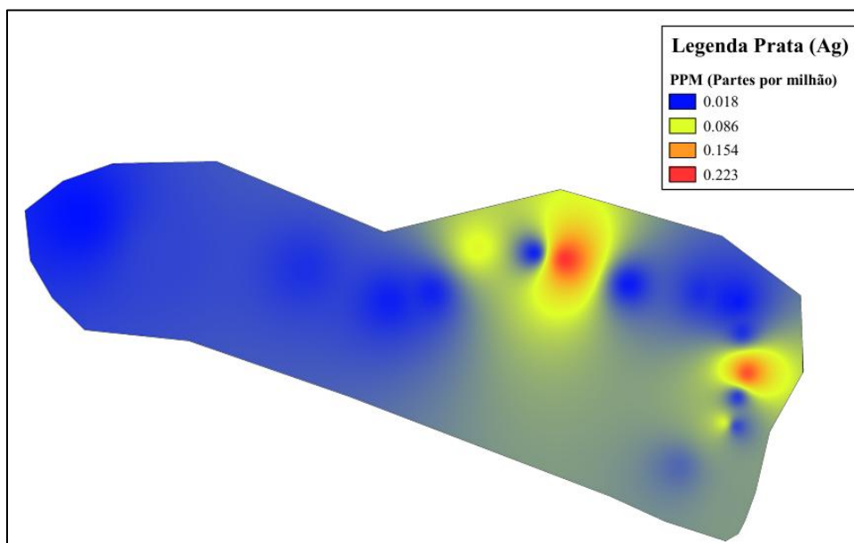
Figura 30 - Isoteores Prata
