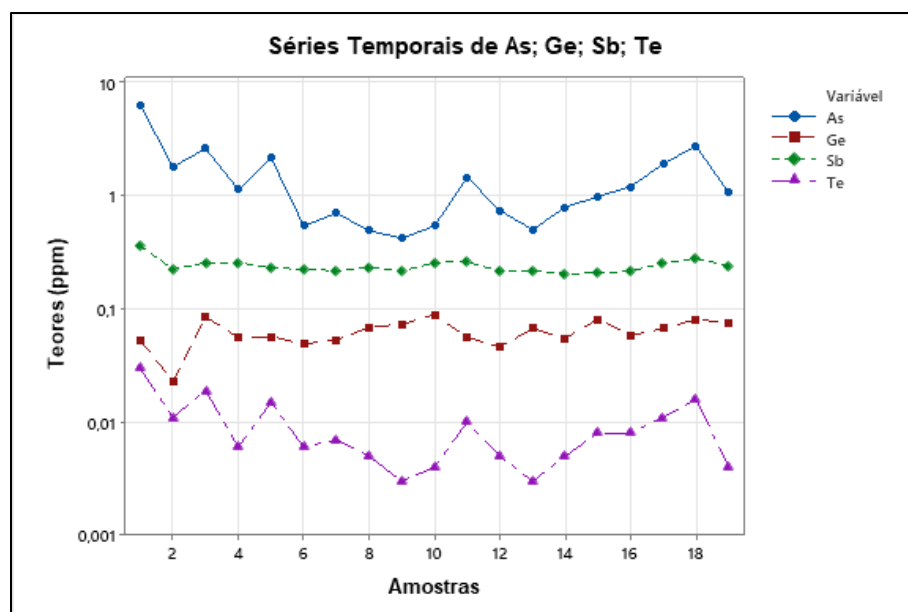
Figura 60 - Série gráfica dos semimetais
