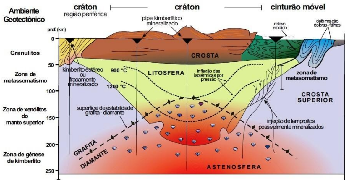
Figura 14 - Ambiente geotectônico dos limites de geração e cristalização de diamantes
