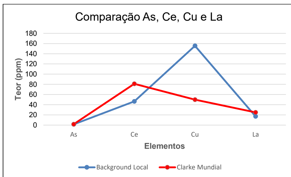
Figura 55 - Comparação dos elementos
