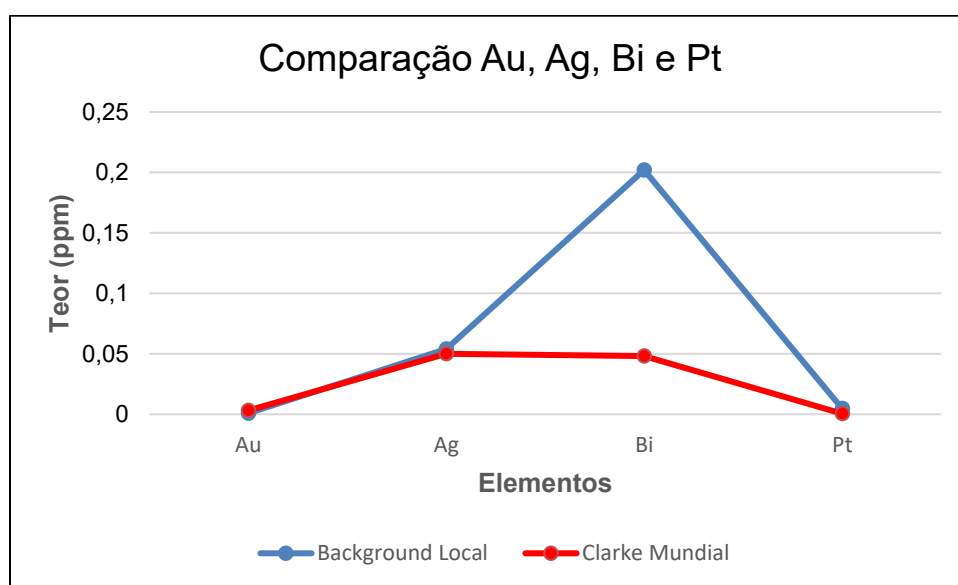
Figura 54 - Comparação dos elementos
