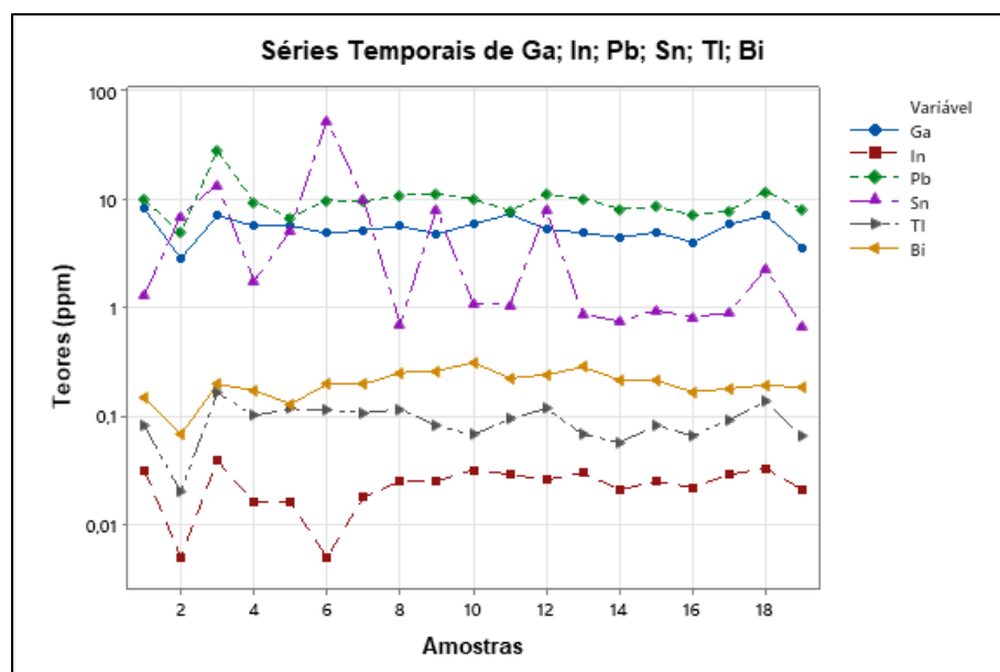
Figura 62 - Série gráfica de outros metais
