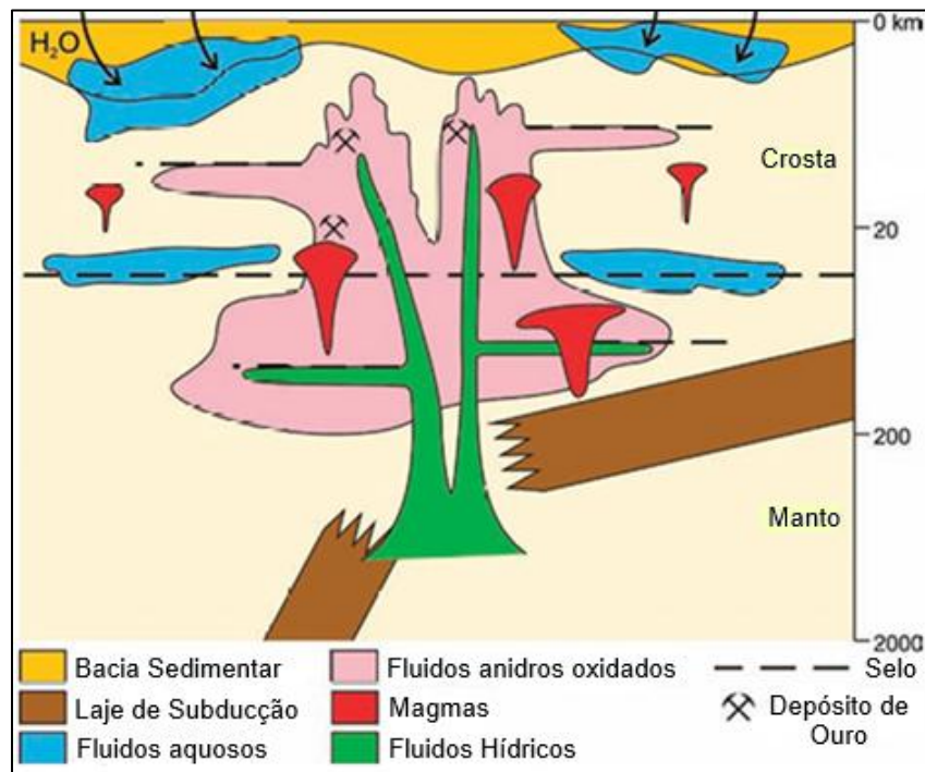
Figura 18 - Perspectiva crosta-manto sobre os sistemas de mineralização de ouro
