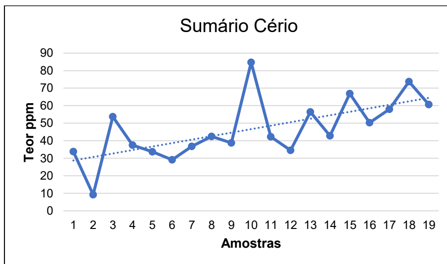
Figura 41 - Distribuição do cério
