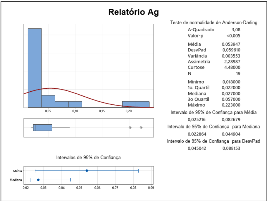
Figura 46 - Sumário gráfico para a prata
