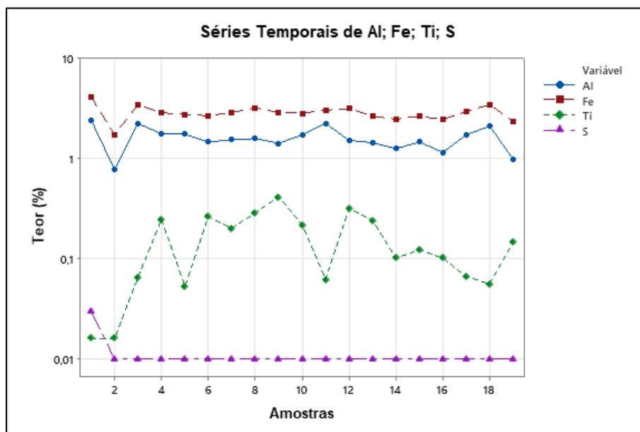
Figura 63 - Série gráfica de alguns elementos em %
