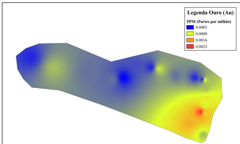
Figura 31 - Isoteores Ouro
