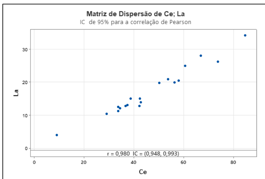
Figura 53 - Correlação gráfica entre Ce e La
