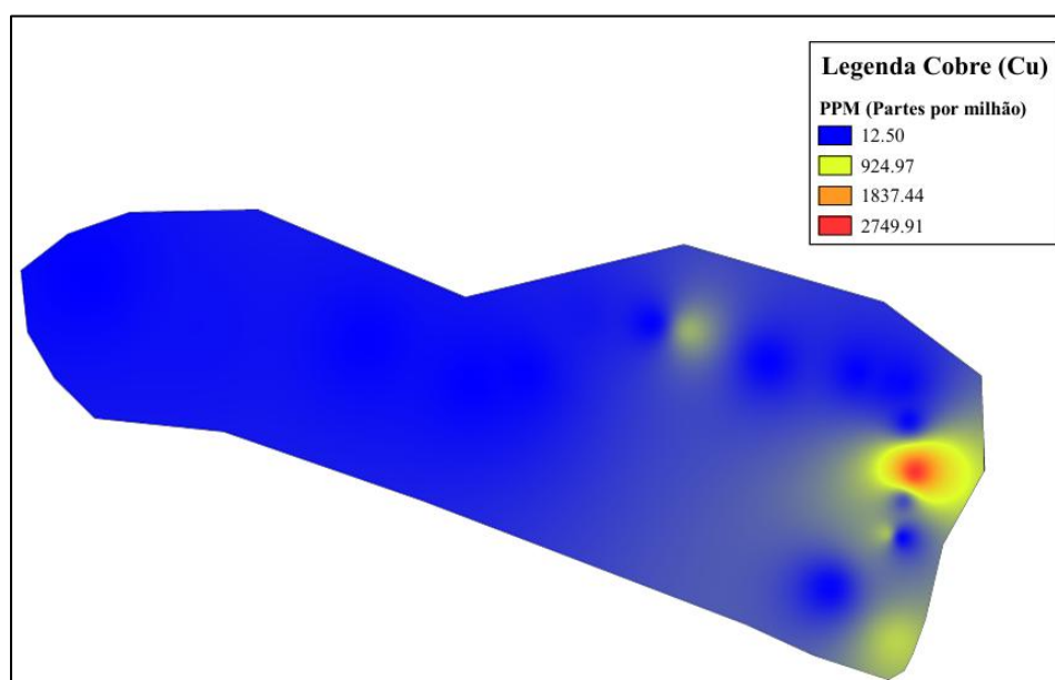
Figura 34 - Isoteores Cobre
