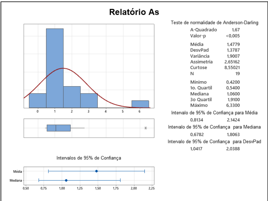
Figura 47 - Sumário gráfico para o arsênio
