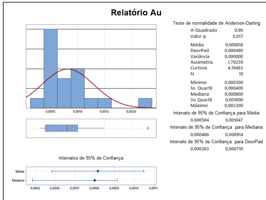
Figura 45 - Sumário gráfico para o ouro
