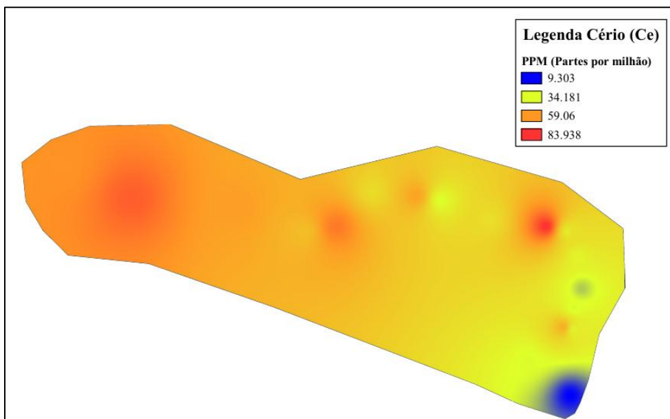
Figura 33 - Isotores Cério
