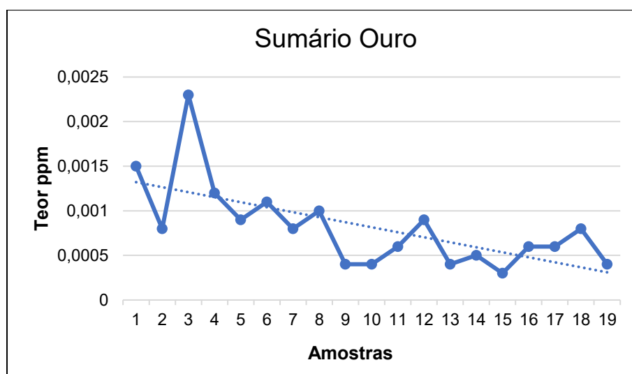
Figura 37 - Distribuição do ouro
