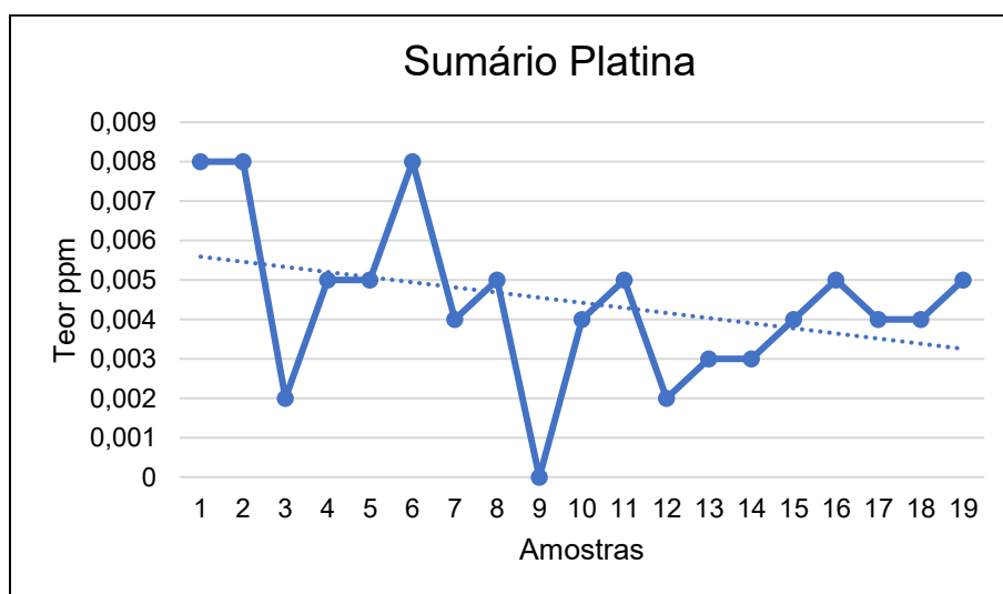
Figura 44 - Distribuição da Platina
