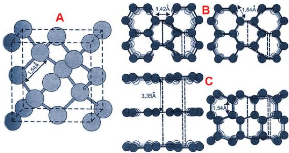
Figura 11 - Estruturas do carbono na natureza, com suas distâncias Inter atômicas
