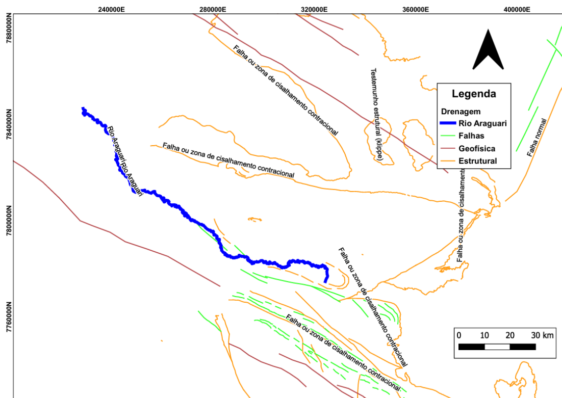
Figura 65 - Mapa Estrutural da região no entorno do rio Araguari
