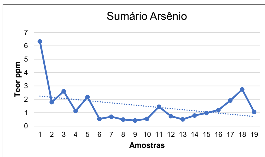
Figura 38 - Distribuição do arsênio
