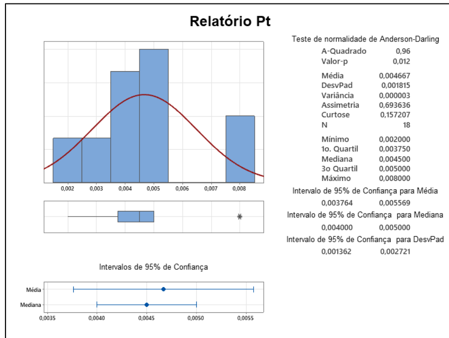
Figura 52 - Sumário gráfico para a platina
