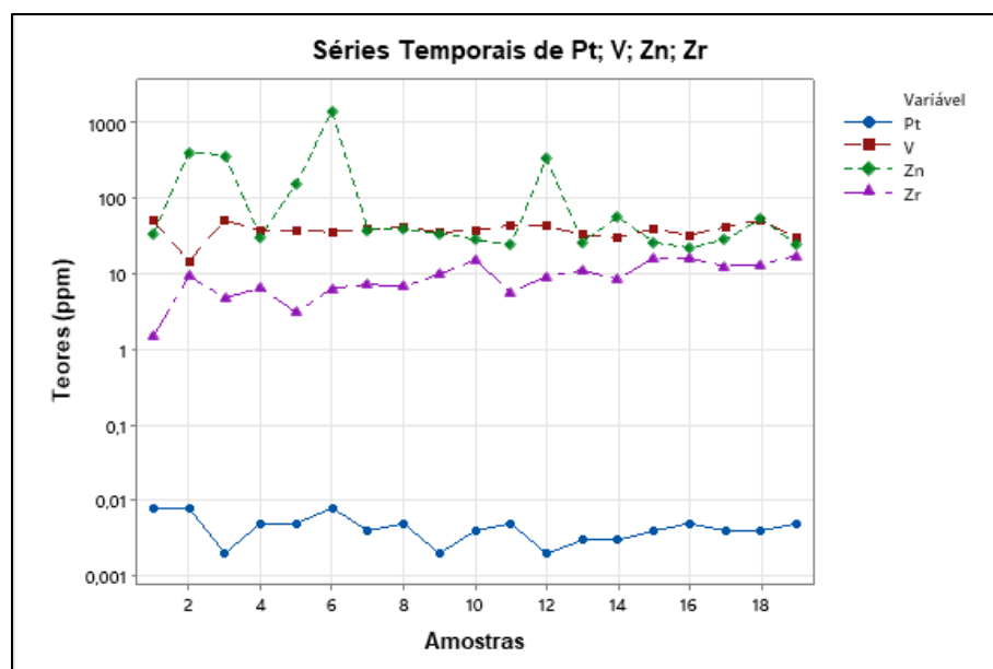
Figura 58 - Curva gráfica metais de transição (ppm)
