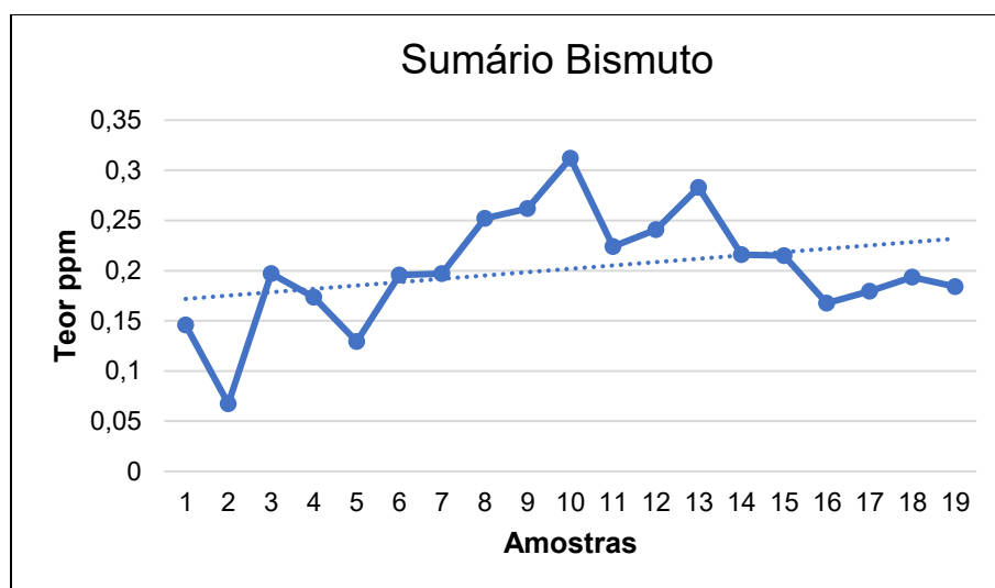
Figura 40 - Distribuição do bismuto
