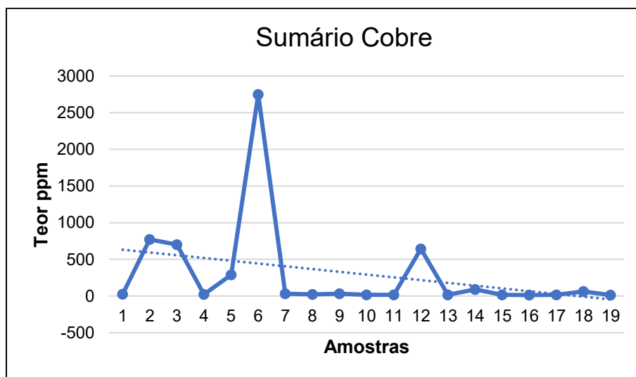
Figura 42 - Distribuição do cobre
