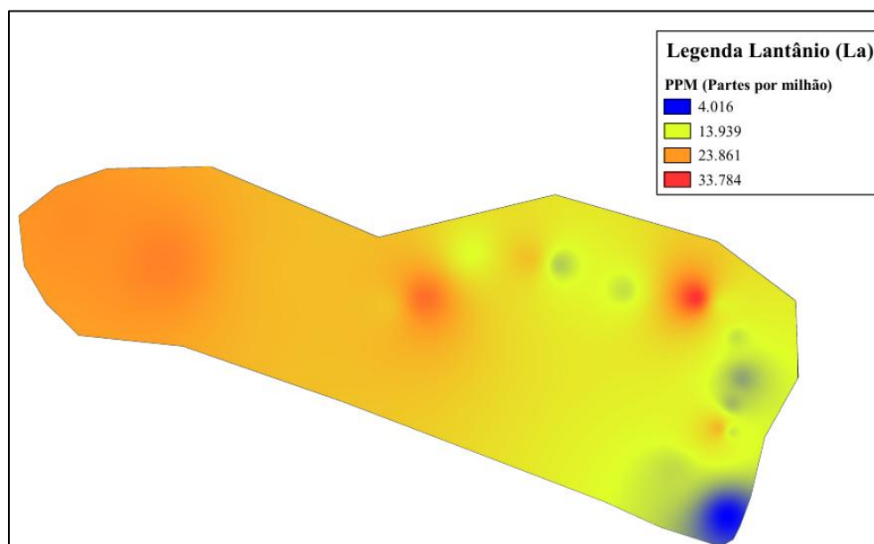
Figura 35 - Isoteores Lantânio
