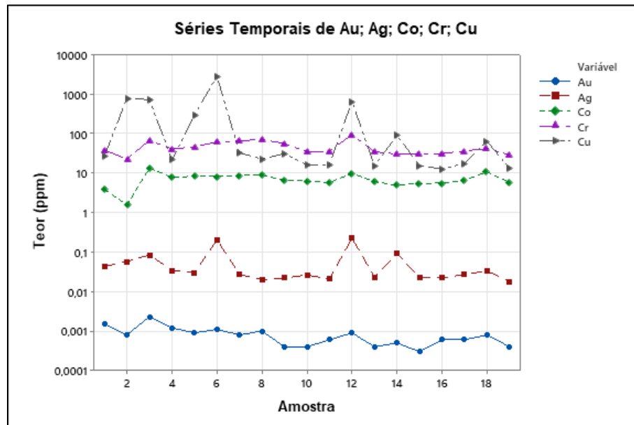
Figura 56 - Curva gráfica metais de transição (ppm)
