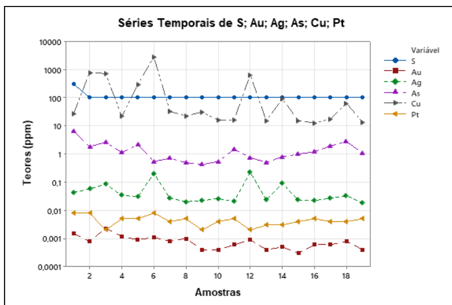
Figura 64 - Série gráfica de elementos estudados
