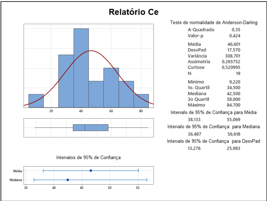
Figura 49 - Sumário gráfico para o cério
