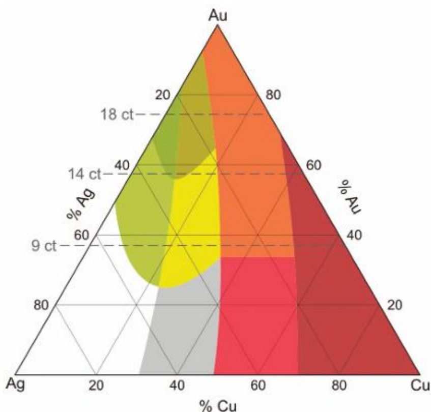
Figura 17 - Variações de cor do ouro no sistema ternário
