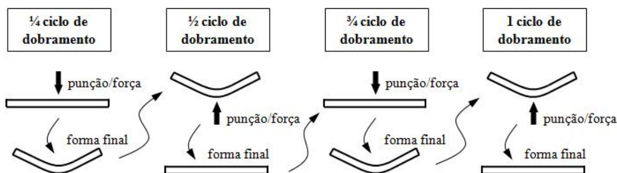
Figura 22 - Representação esquemática do processamento cíclico: \frac{1}{4} de ciclo, \frac{1}{2} ciclo, \frac{3}{4} de ciclo e 1 ciclo de dobramento.
