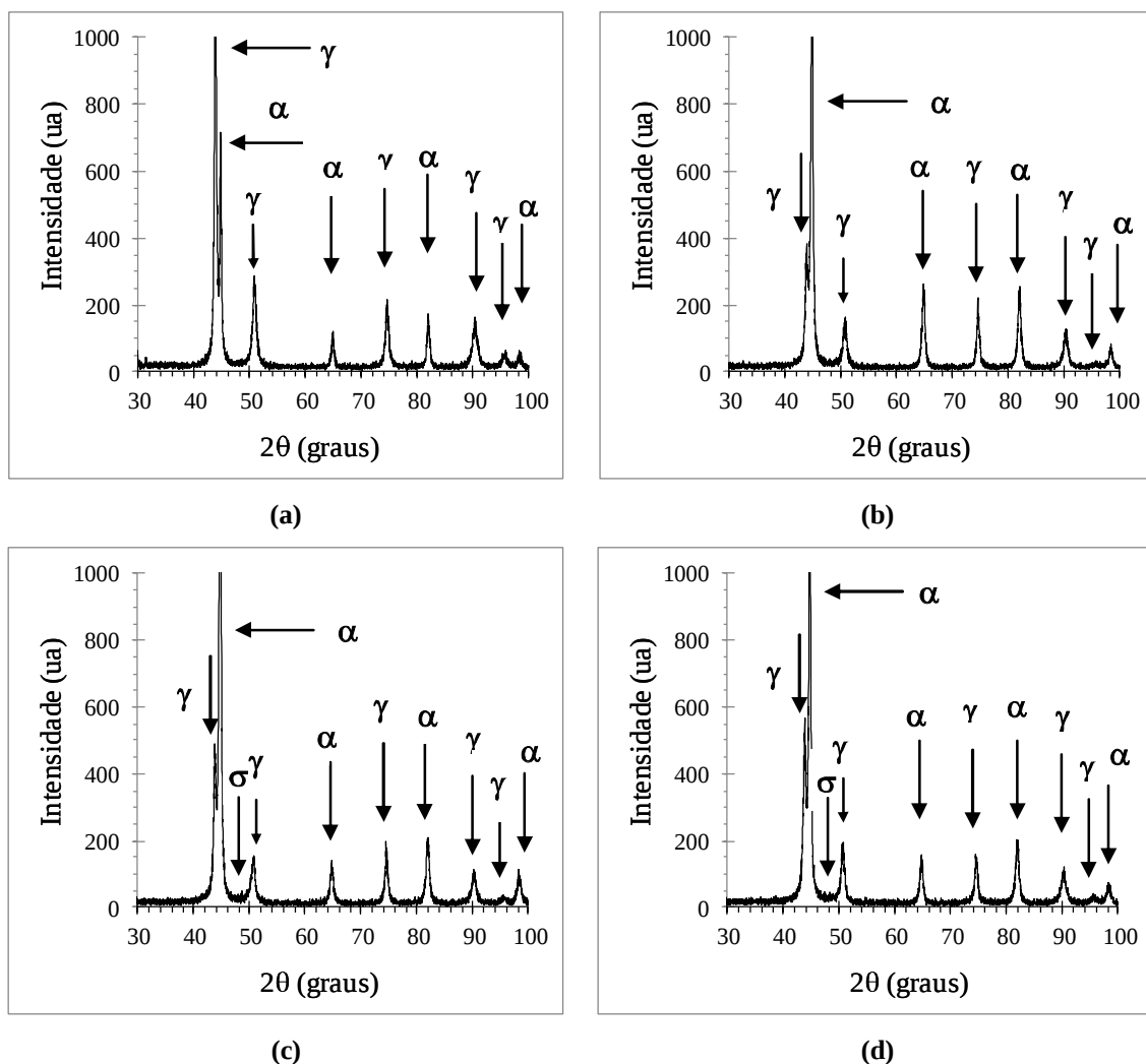
Figura 45 - Difrátogramas do aço UNS31803: (a) Como recebido; tratado termicamente 700°C: (b) 20 minutos; (c) 40 minutos; (d) 60 minutos.
