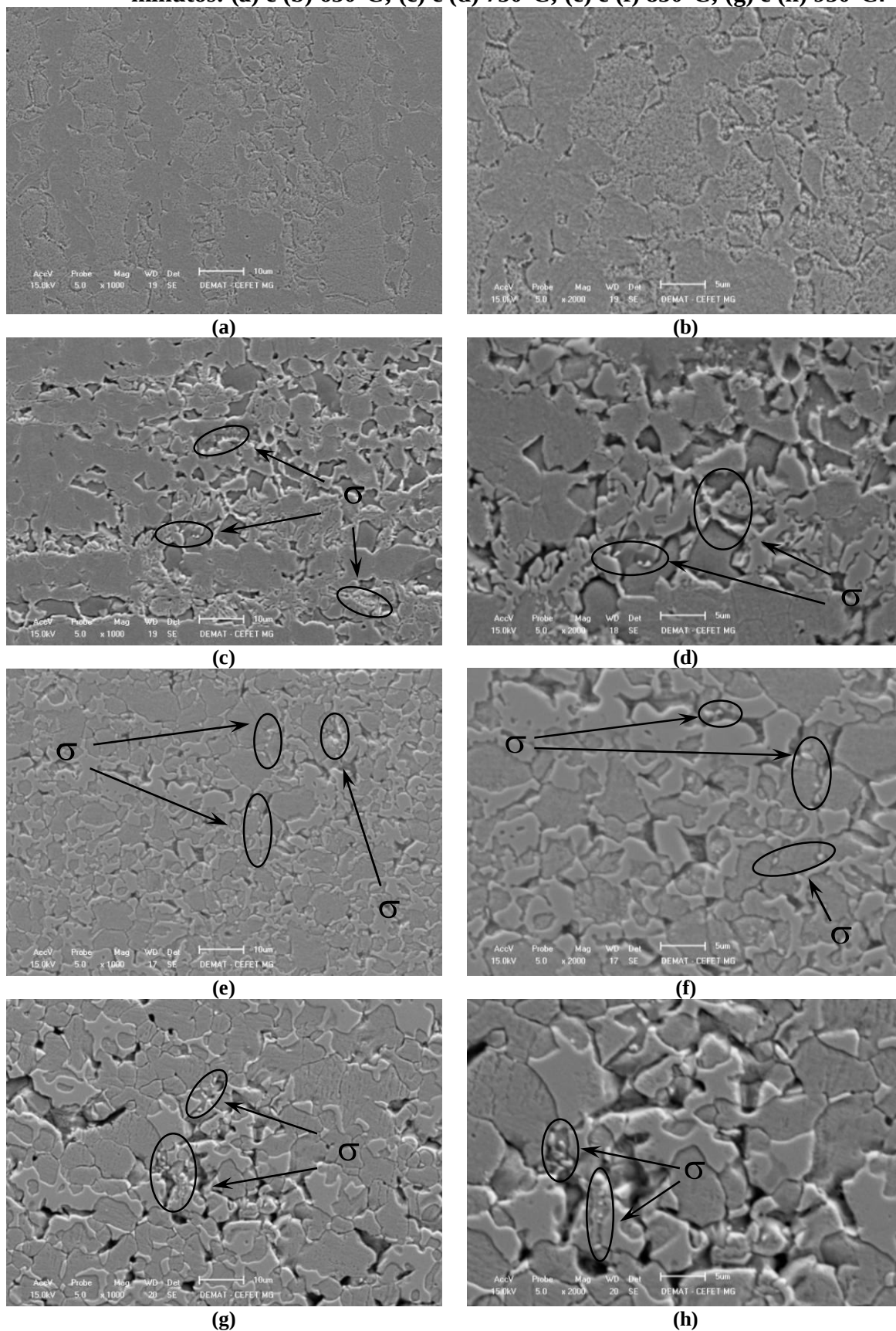
Figura 41 - Micrografias do aço UNS31803 tratado termicamente (MEV), durante 60 minutos: (a) e (b) 650°C; (c) e (d) 750°C; (e) e (f) 850°C; (g) e (h) 950°C.
