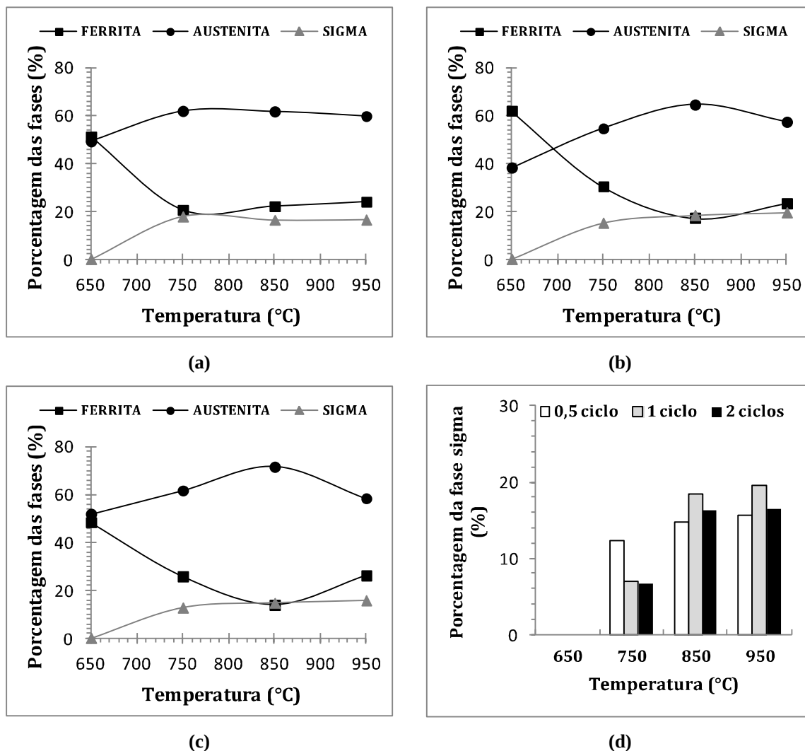
Figura 67 - Porcentagens das fases desenvolvidas no aço inoxidável UNS31803 dobrado e tratado termicamente a 60 minutos: (a) 0,5 ciclo - \alpha , \gamma e \sigma ; (b) 1 ciclo - \alpha , \gamma e \sigma ; (c) 2 ciclos - \alpha , \gamma e \sigma ; (d) todos os ciclos de dobramento - \sigma .
