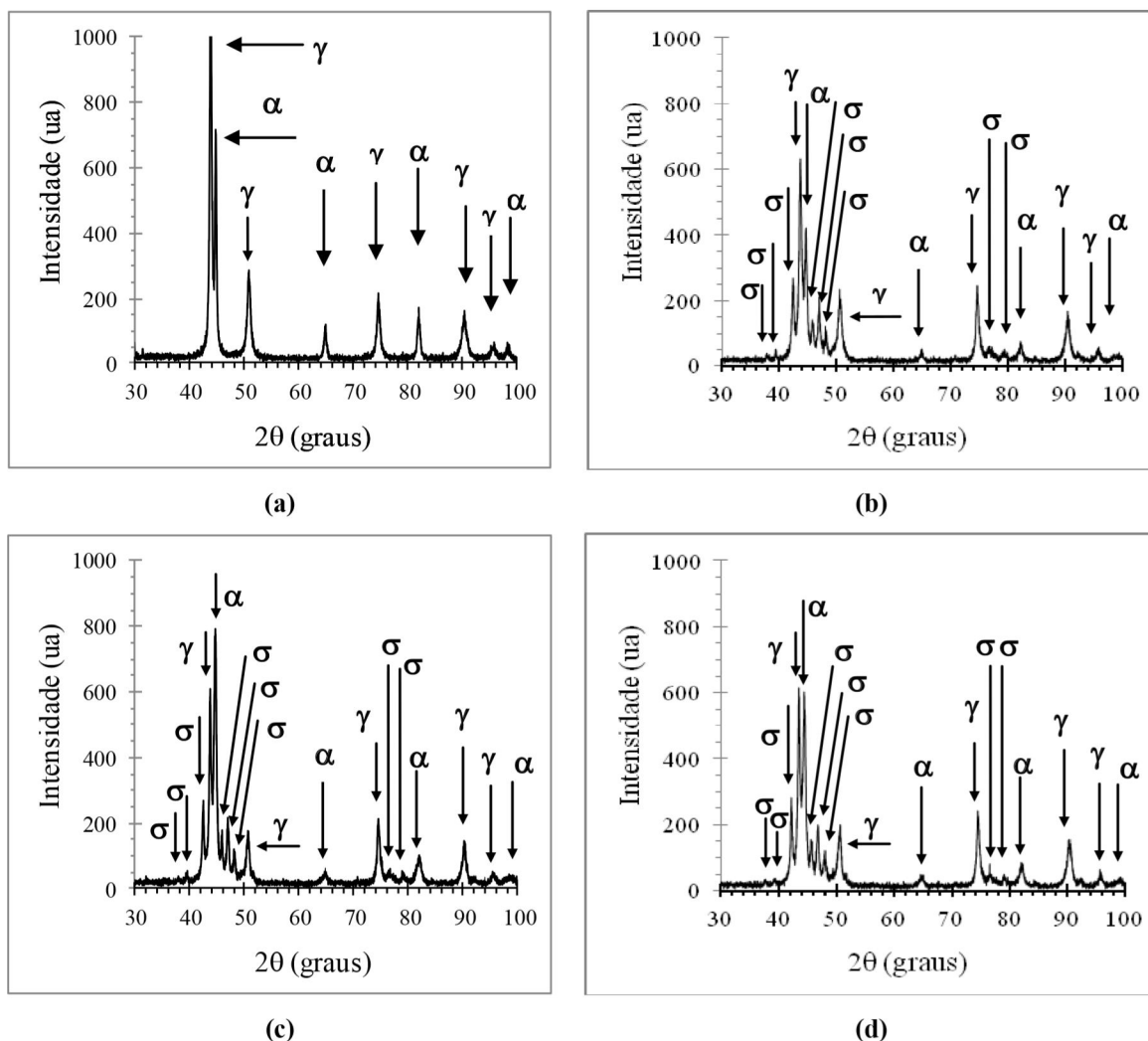
Figura 50 - Difrátogramas do aço UNS31803: (a) Como recebido; tratado termicamente 950°C: (b) 20 minutos; (c) 40 minutos; (d) 60 minutos.
