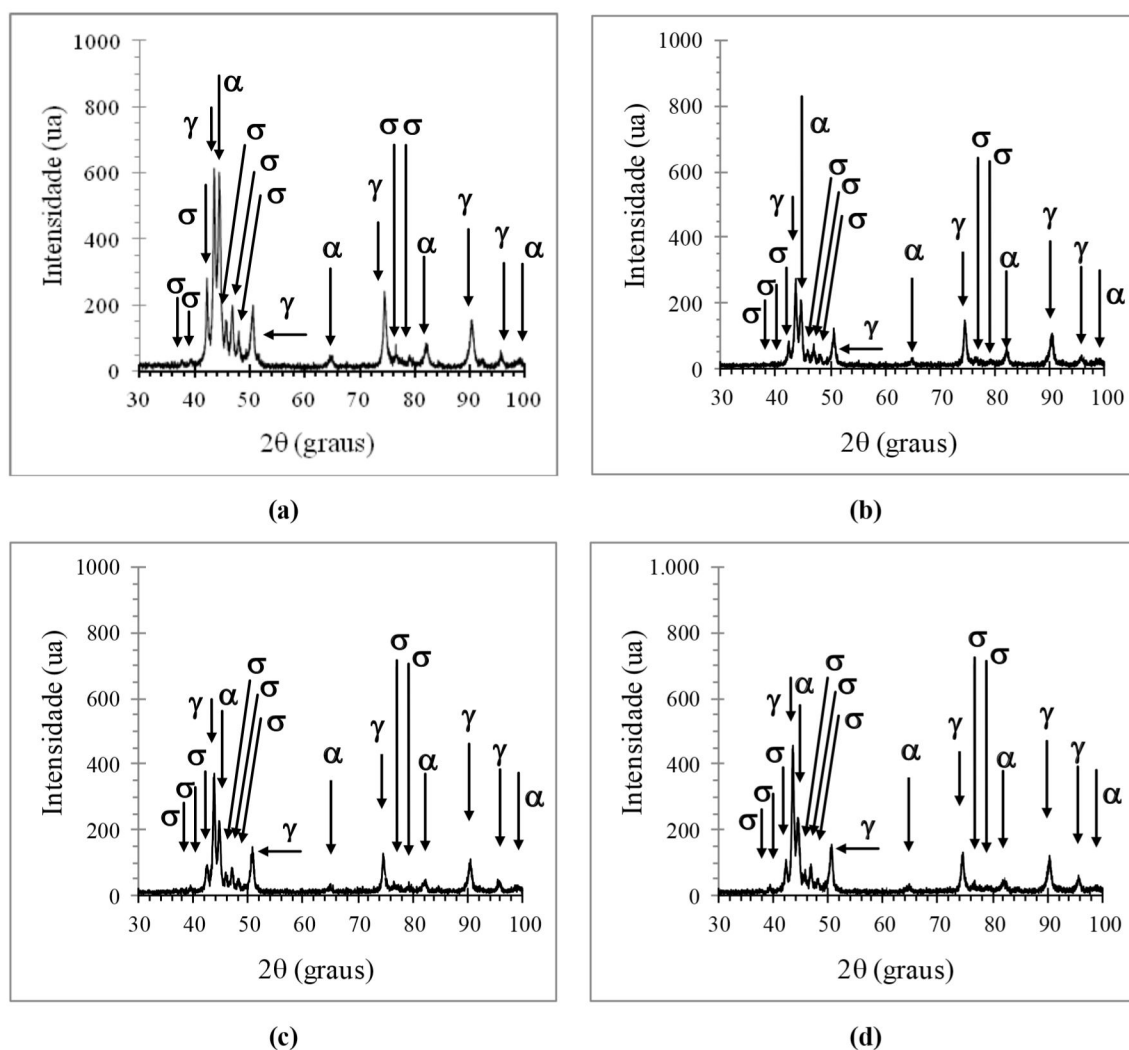
Figura 66 - Difratomogramas do aço UNS31803: (a) tratado termicamente a 950°C; processado mecanicamente (dobrado) e tratado termicamente 950°C: (b) 0,5 ciclo; (c) 1 ciclo; (d) 2 ciclos.
