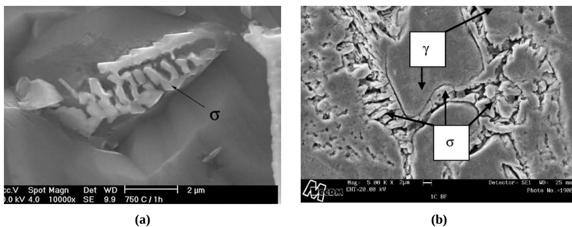
Figura 42 - Micrografias (MEV) de aços duplex evidenciando o desenvolvimento da fase sigma: (a) aço UNS31803 tratado a 750°C, por 60 minutos e resfriado em água; (b) aço ASTM 890 GR1C SDSS, resfriado a partir do estado líquido.
