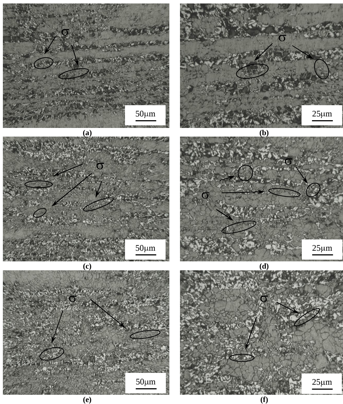
Figura 37 - Micrografias do aço UNS31803 tratado termicamente a 800°C: (a) 20 min. – 200X; (b) 20 min. – 400X; (c) 40 min. - 200X; (d) 40 min. - 400X; (e) 60 min. – 200X; (f) 60 min. – 400X.
