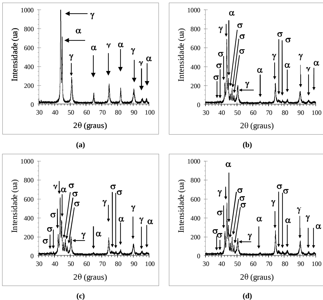
Figura 49 - Difrátogramas do aço UNS31803: (a) Como recebido; tratado termicamente 900°C: (b) 20 minutos; (c) 40 minutos; (d) 60 minutos.
