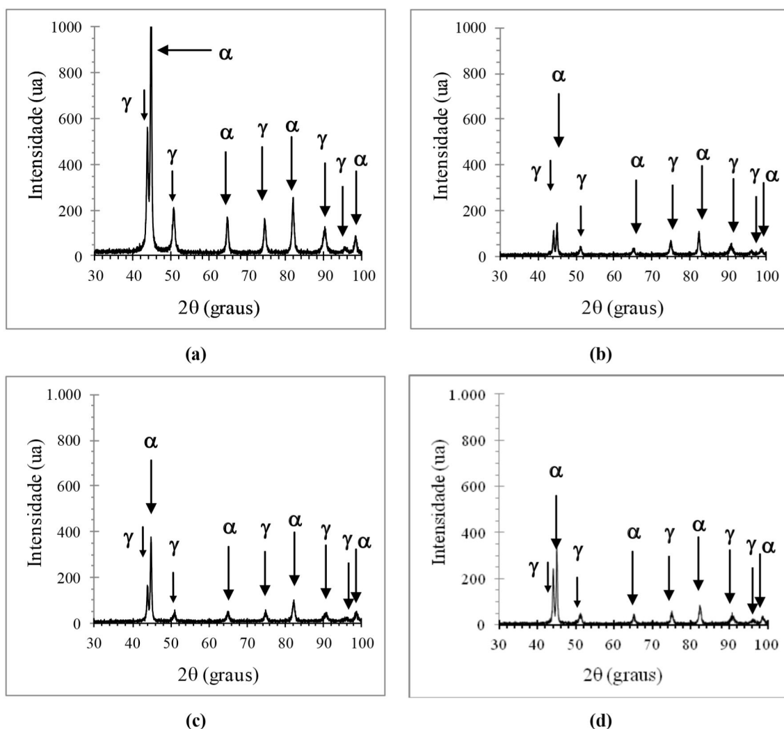
Figura 63 - Difratomogramas do aço UNS31803: (a) tratado termicamente 650°C; processado mecanicamente (dobrado) e tratado termicamente 650°C: (b) 0,5 ciclo; (c) 1 ciclo; (d) 2 ciclos.
