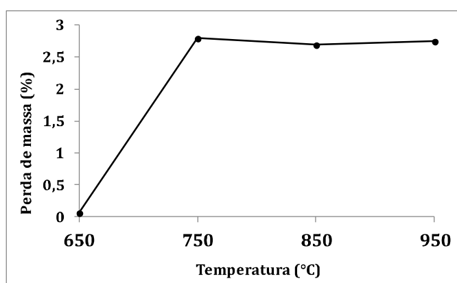
Figura 69 - Análise da porcentagem da perda de massa das amostras tratadas termicamente.
