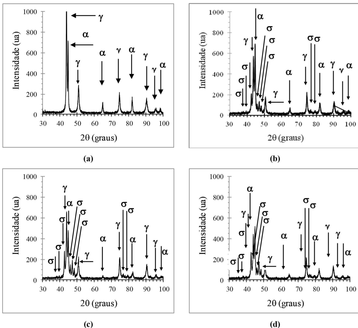
Figura 47 - Difrátogramas do aço UNS31803: (a) Como recebido; tratado termicamente 800°C: (b) 20 minutos; (c) 40 minutos; (d) 60 minutos.
