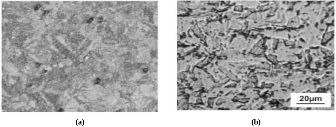
Figura 5 - Microestrutura de aços inoxidáveis endurecíveis por precipitação. (a) PH 13-8Mo, endurecível por precipitação à base de Cu, (b) Aço-Nb, endurecível por precipitação com uso de Nb.
