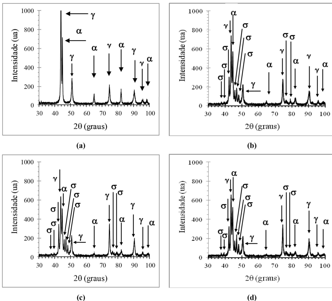
Figura 48 - Difrátogramas do aço UNS31803: (a) Como recebido; tratado termicamente 850°C: (b) 20 minutos; (c) 40 minutos; (d) 60 minutos.
