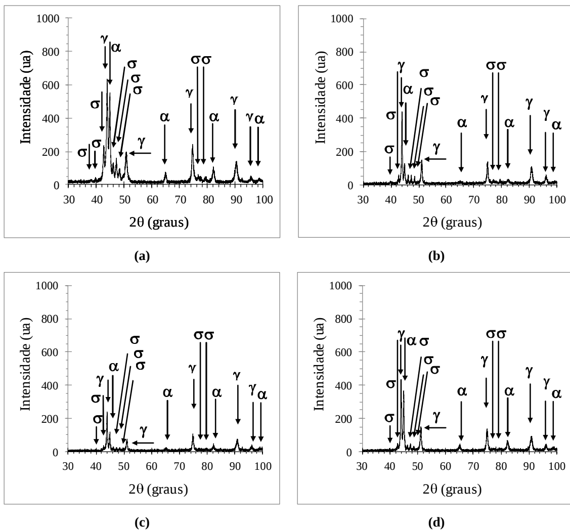
Figura 64 - Difratomogramas do aço UNS31803: (a) tratado termicamente a 750°C; processado mecanicamente (dobrado) e tratado termicamente 750°C: (b) 0,5 ciclo; (c) 1 ciclo; (d) 2 ciclos.
