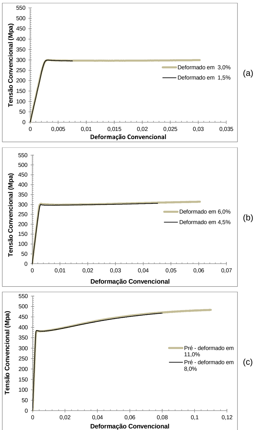
Figura 6. 8 - Curvas tensão X deformação do aço GO deformado em diferentes magnitudes
