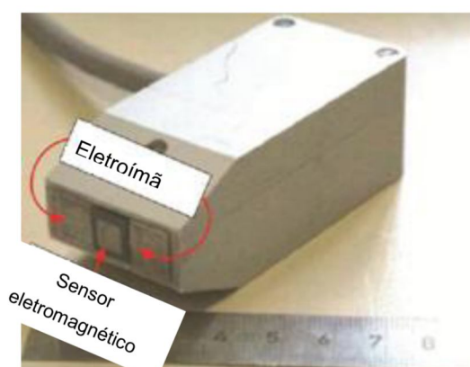
Figura 3. 13 - Sonda magnetoelástica
