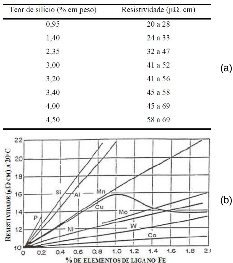
Figura 4. 3 - Resistividade elétrica
