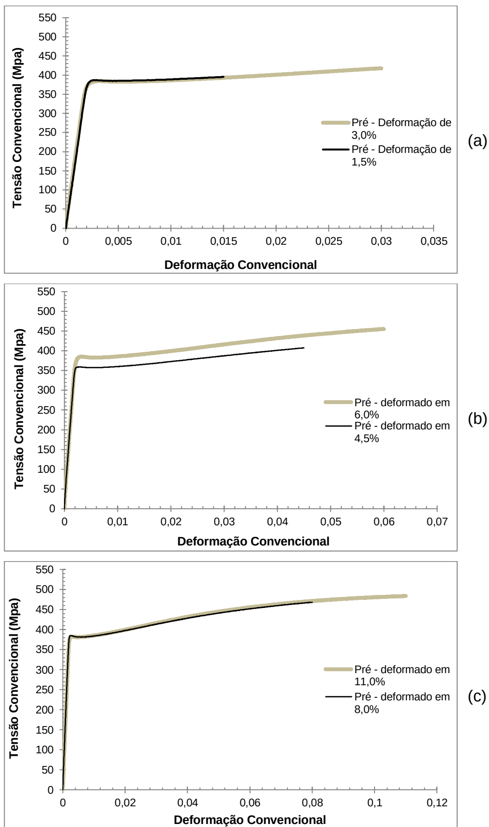
Figura 6. 7 - Curvas tensão X deformação do aço GNO deformado em diferentes magnitudes
