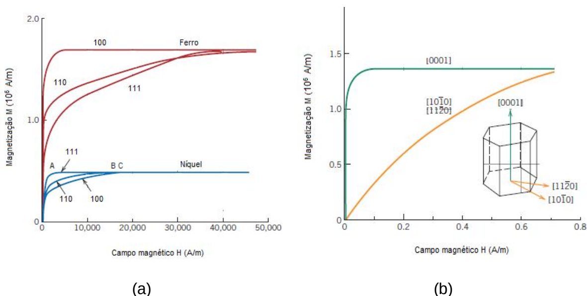
Figura 3. 2 - Direções de magnetização
