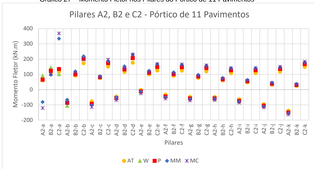
Gráfico 27 – Momento Fletor nos Pilares do Pórtico de 11 Pavimentos
