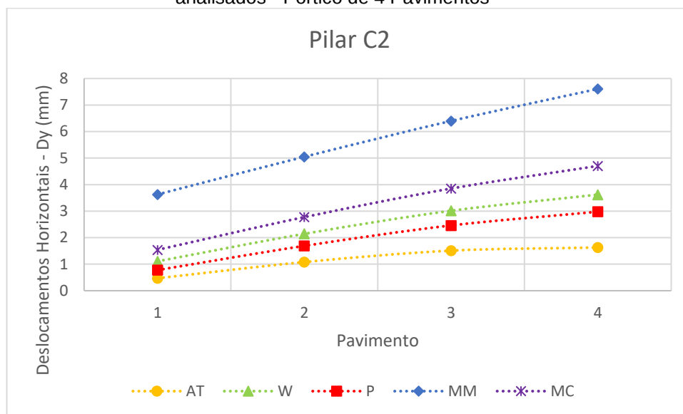
Gráfico 1 - Comparação dos deslocamentos horizontais no topo dos andares para todos os modelos analisados - Pórtico de 4 Pavimentos
