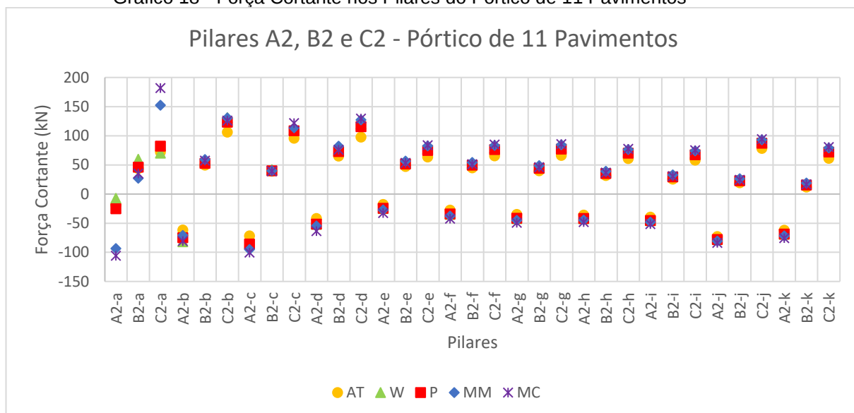
Gráfico 18 - Força Cortante nos Pilares do Pórtico de 11 Pavimentos
