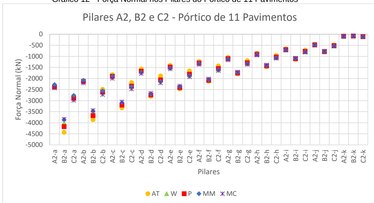
Gráfico 12 - Força Normal nos Pilares do Pórtico de 11 Pavimentos
