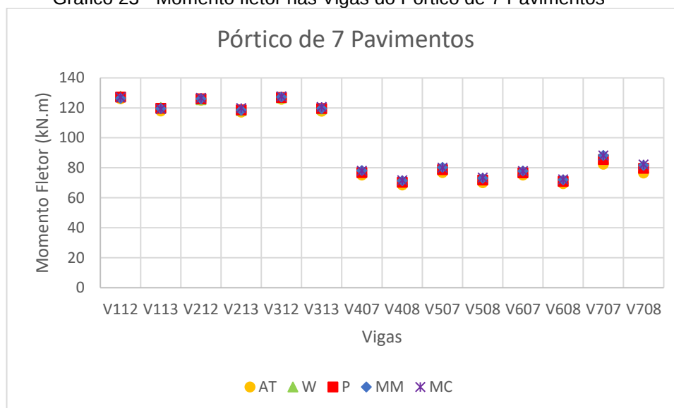
Gráfico 23 - Momento fletor nas Vigas do Pórtico de 7 Pavimentos
