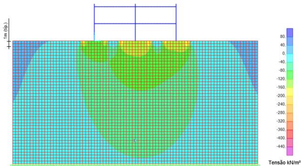
Figura 19 - Bulbo de Tensões - Pórtico de 11 pavimentos
