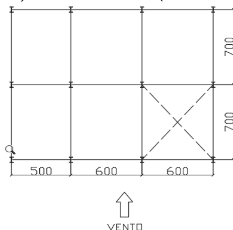
Figura 17 - Direção do vento analisada (medidas em cm)
