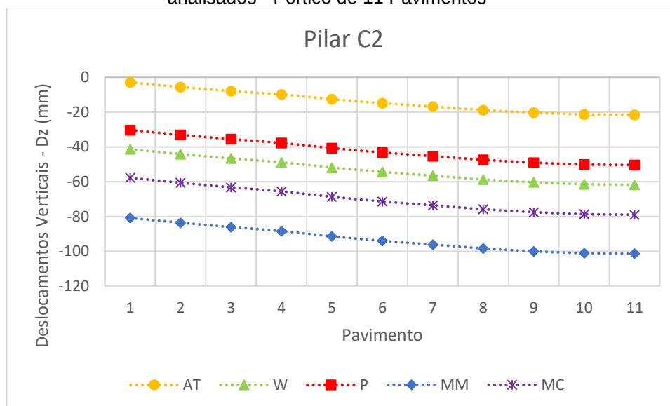
Gráfico 6 - Comparação dos deslocamentos verticais no topo dos andares para todos os modelos analisados - Pórtico de 11 Pavimentos
