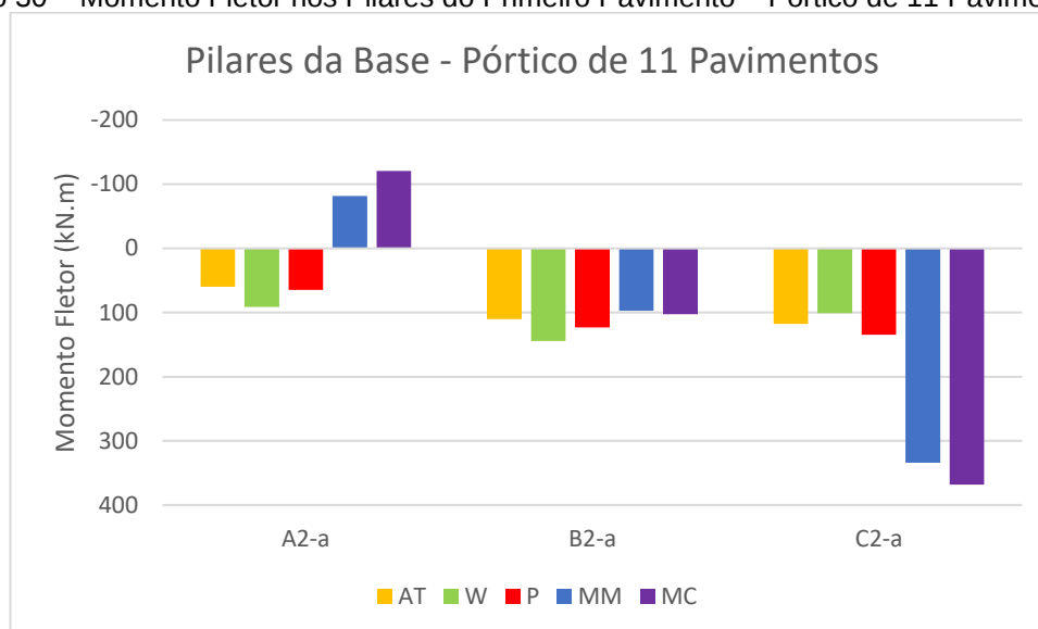
Gráfico 30 – Momento Fletor nos Pilares do Primeiro Pavimento – Pórtico de 11 Pavimentos
