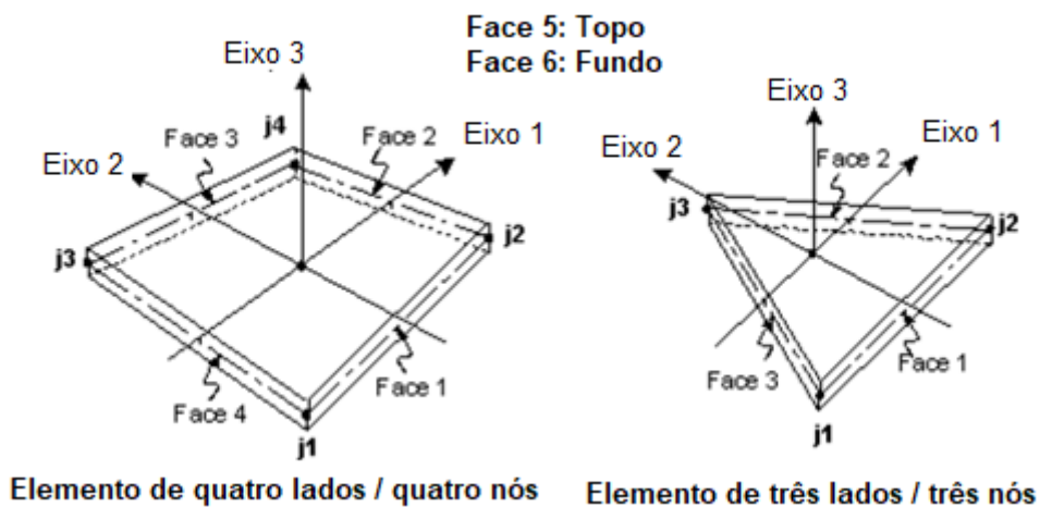
Figura 15 - Sistema de coordenadas locais dos elementos de placa no SAP 2000
