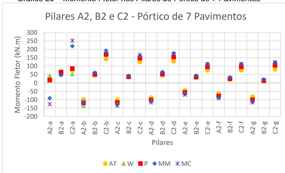
Gráfico 26 – Momento Fletor nos Pilares do Pórtico de 7 Pavimentos
