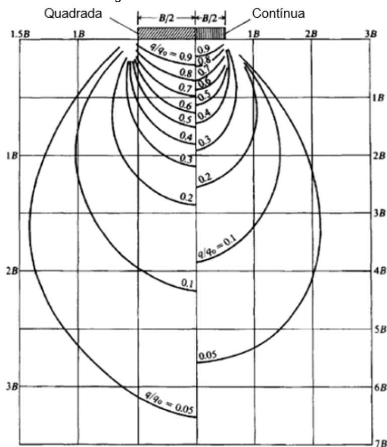
Figura 9 - Bulbo de tensões
