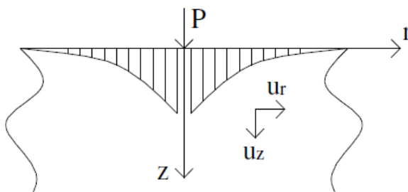
Figura 8 - Superfície de deslocamentos para carregamento no semi-espaço.
