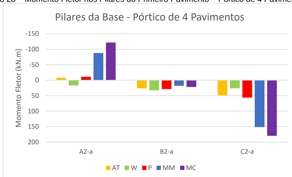
Gráfico 28 – Momento Fletor nos Pilares do Primeiro Pavimento – Pórtico de 4 Pavimentos
