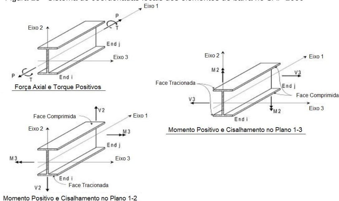
Figura 13 - Sistema de coordenadas locais dos elementos de barra no SAP 2000
