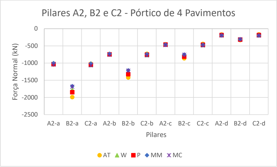
Gráfico 10 - Força Normal nos Pilares do Pórtico de 4 Pavimentos
