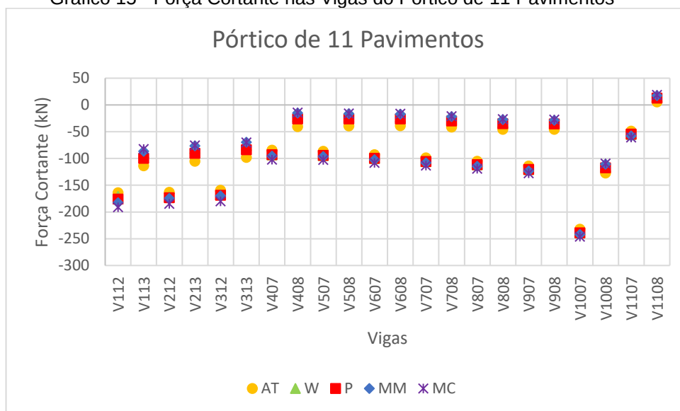
Gráfico 15 - Força Cortante nas Vigas do Pórtico de 11 Pavimentos
