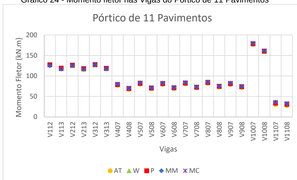
Gráfico 24 - Momento fletor nas Vigas do Pórtico de 11 Pavimentos
