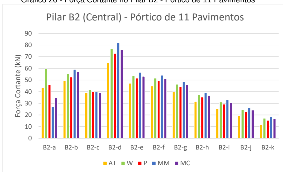
Gráfico 20 - Força Cortante no Pilar B2 - Pórtico de 11 Pavimentos
