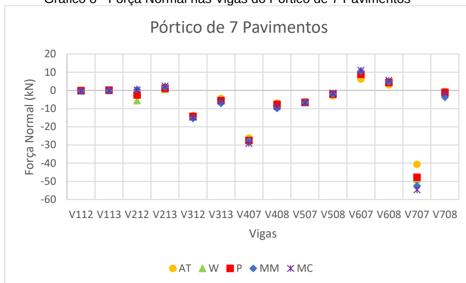
Gráfico 8 - Força Normal nas Vigas do Pórtico de 7 Pavimentos
