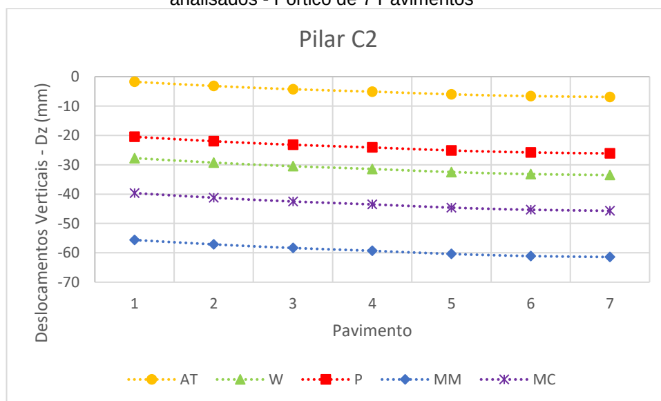
Gráfico 5 - Comparação dos deslocamentos verticais no topo dos andares para todos os modelos analisados - Pórtico de 7 Pavimentos
