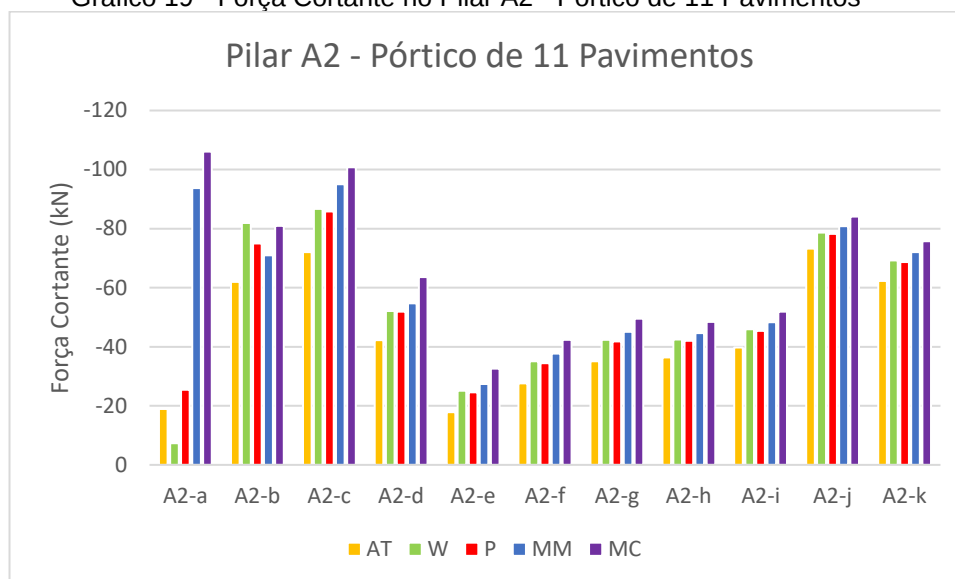
Gráfico 19 - Força Cortante no Pilar A2 - Pórtico de 11 Pavimentos
