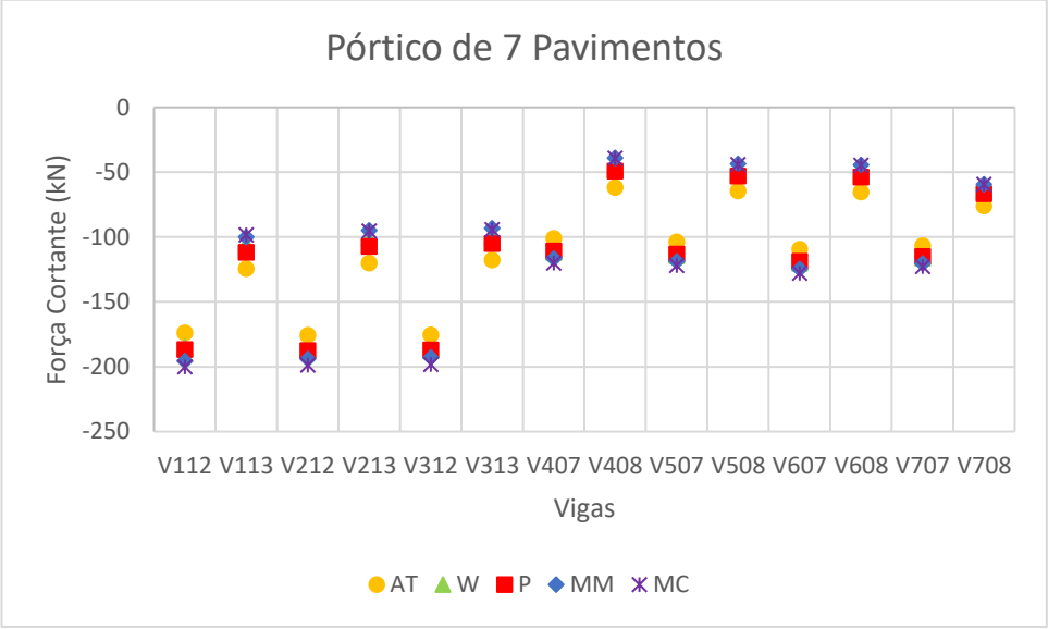
Gráfico 14 - Força Cortante nas Vigas do Pórtico de 7 Pavimentos
