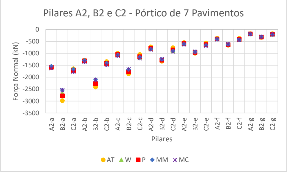
Gráfico 11 - Força Normal nos Pilares do Pórtico de 7 Pavimentos
