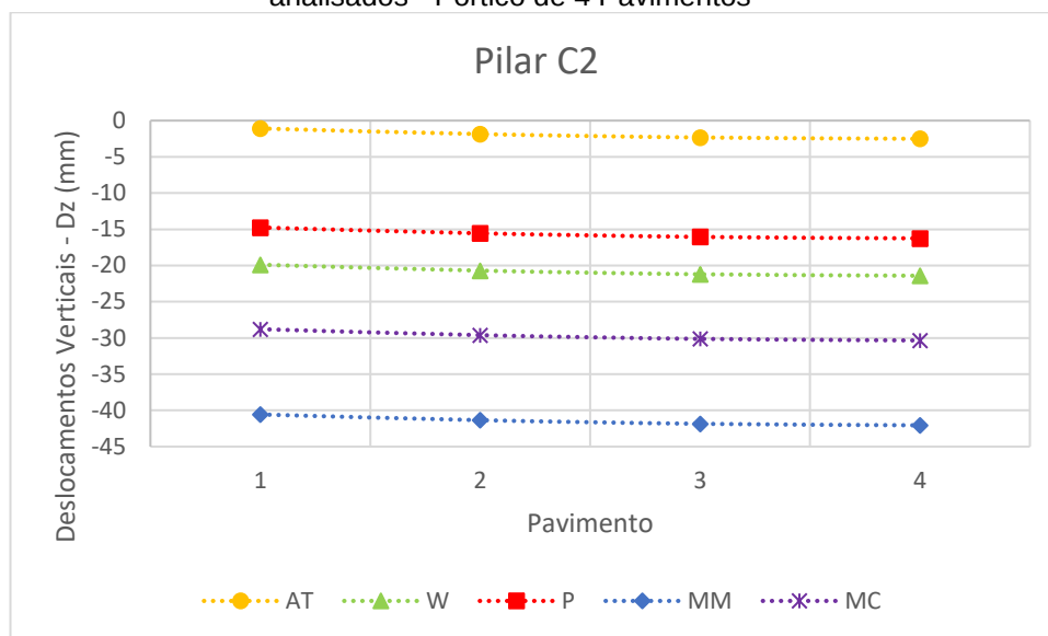
Gráfico 4 - Comparação dos deslocamentos verticais no topo dos andares para todos os modelos analisados - Pórtico de 4 Pavimentos
