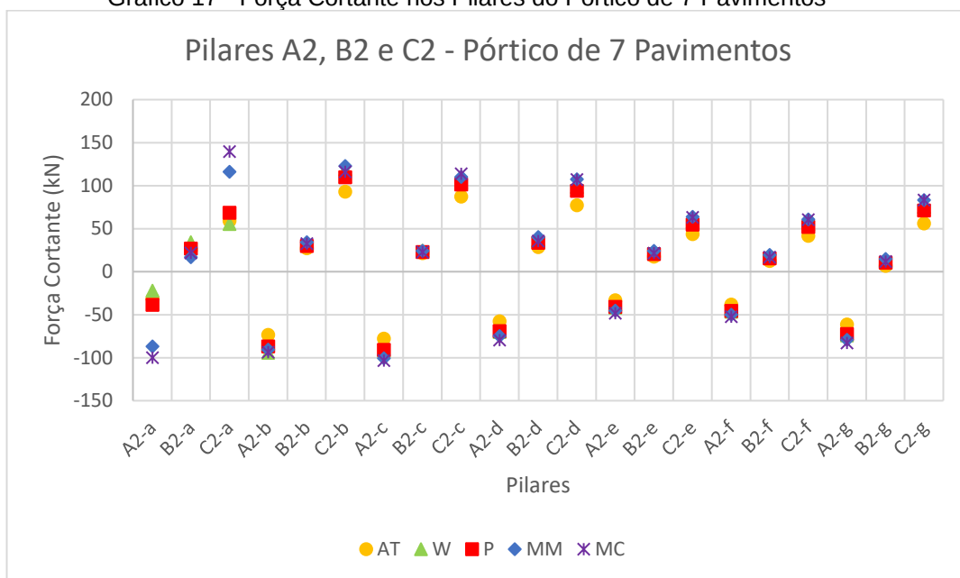
Gráfico 17 - Força Cortante nos Pilares do Pórtico de 7 Pavimentos
