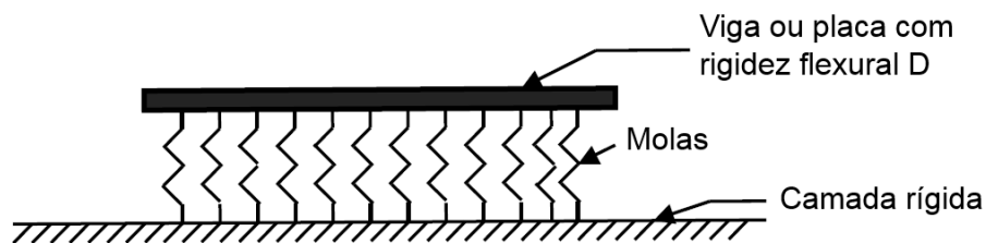
Figura 3 - Modelo de Hetenyi
