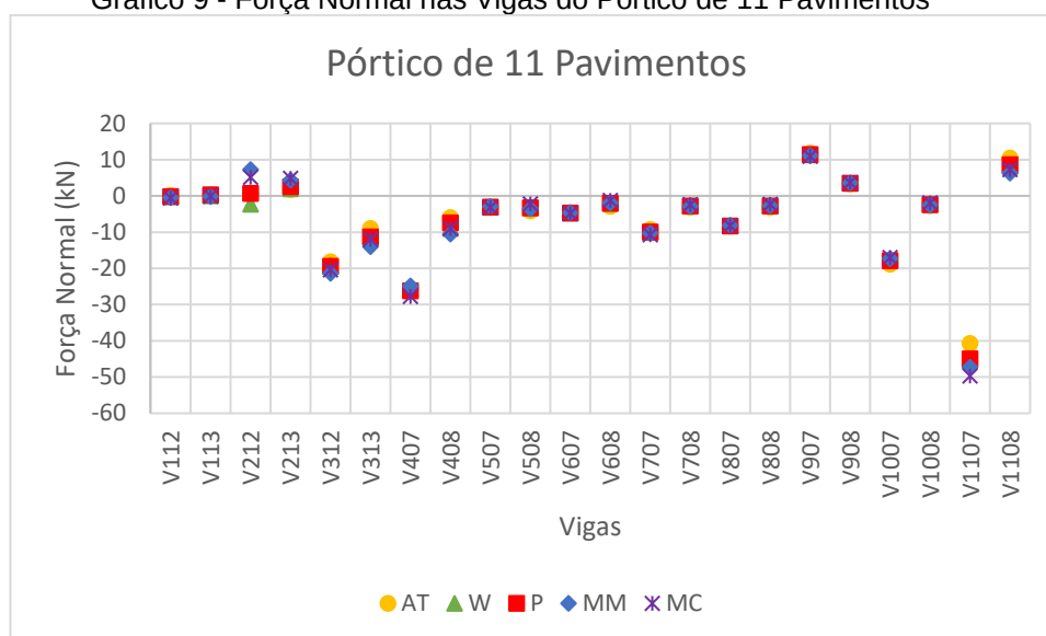
Gráfico 9 - Força Normal nas Vigas do Pórtico de 11 Pavimentos
