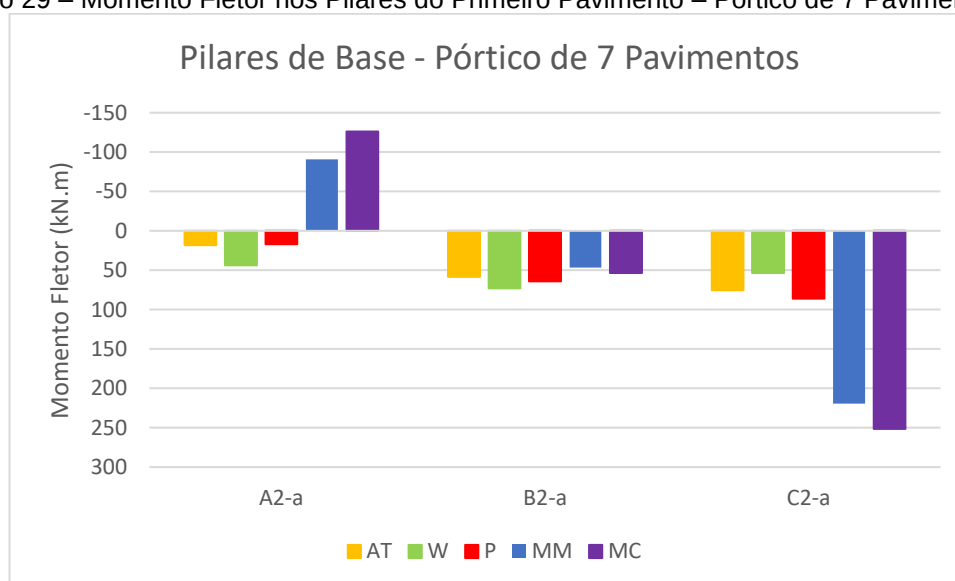
Gráfico 29 – Momento Fletor nos Pilares do Primeiro Pavimento – Pórtico de 7 Pavimentos
