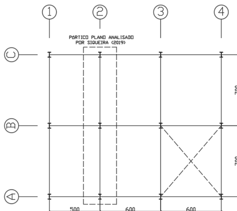
Figura 11 – Planta baixa do edifício em estudo (medidas em cm).
