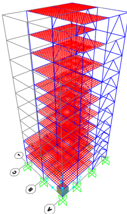
Figura 12 – Modelo 3D do edifício.
