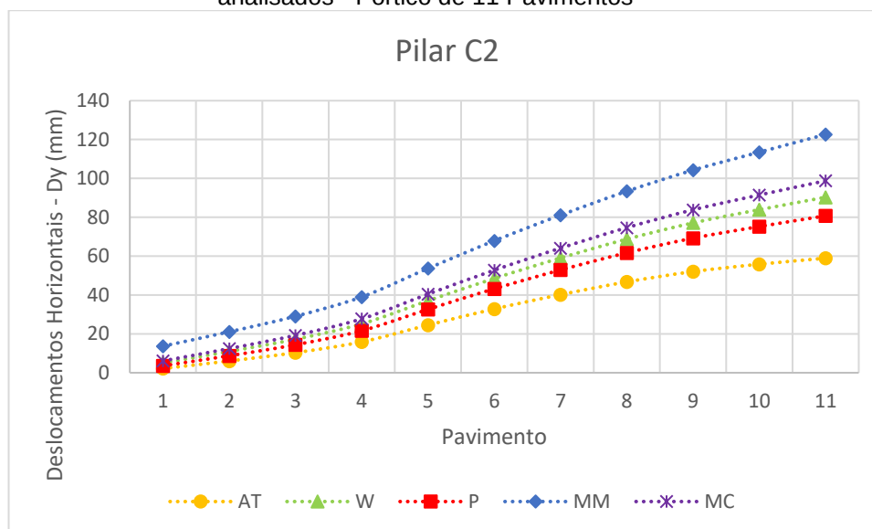
Gráfico 3 - Comparação dos deslocamentos horizontais no topo dos andares para todos os modelos analisados - Pórtico de 11 Pavimentos
