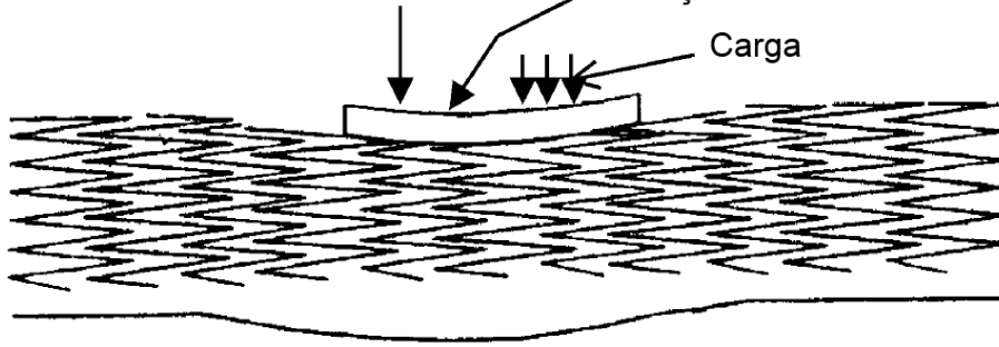
Figura 7 - Modelo de Malha de Molas Fundação
