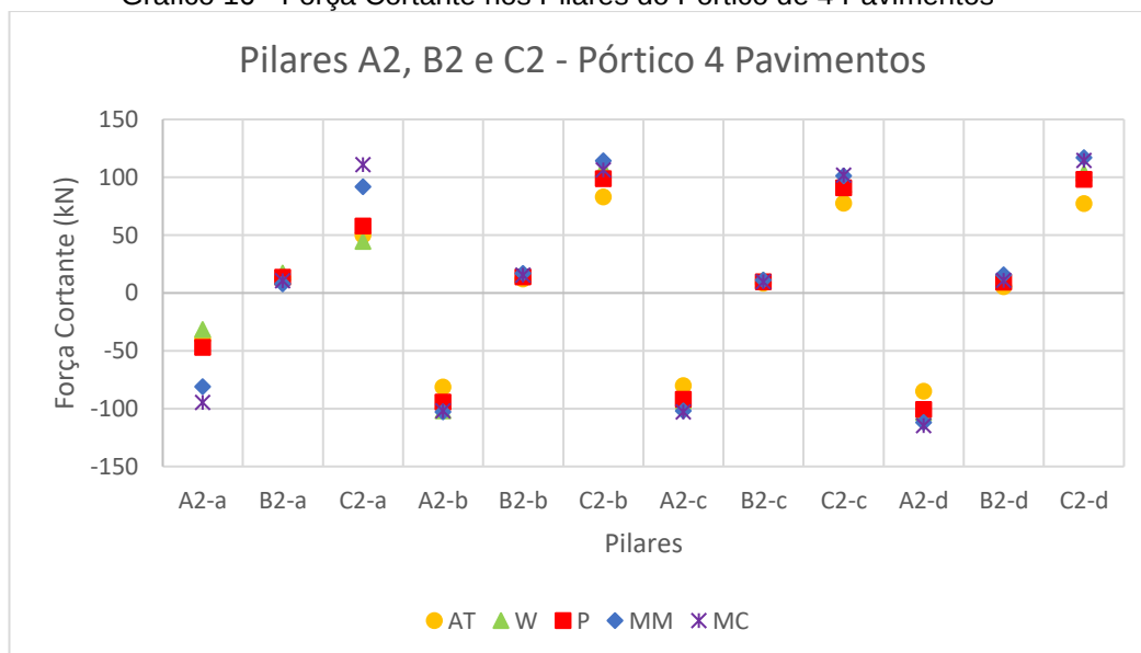
Gráfico 16 - Força Cortante nos Pilares do Pórtico de 4 Pavimentos
