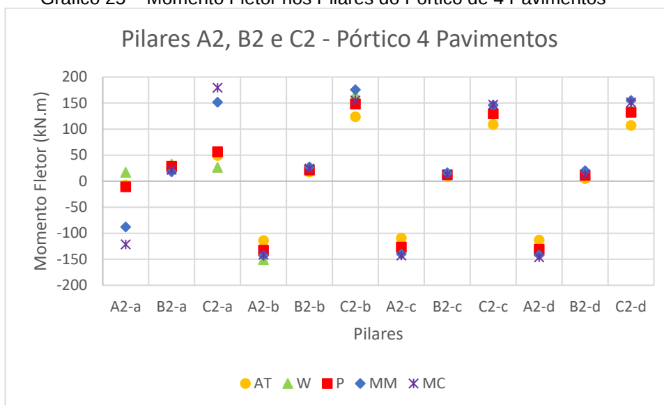
Gráfico 25 – Momento Fletor nos Pilares do Pórtico de 4 Pavimentos
