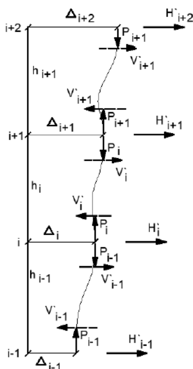
Figura 10 - Sistema de forças laterais e verticais aplicadas nos nós.
