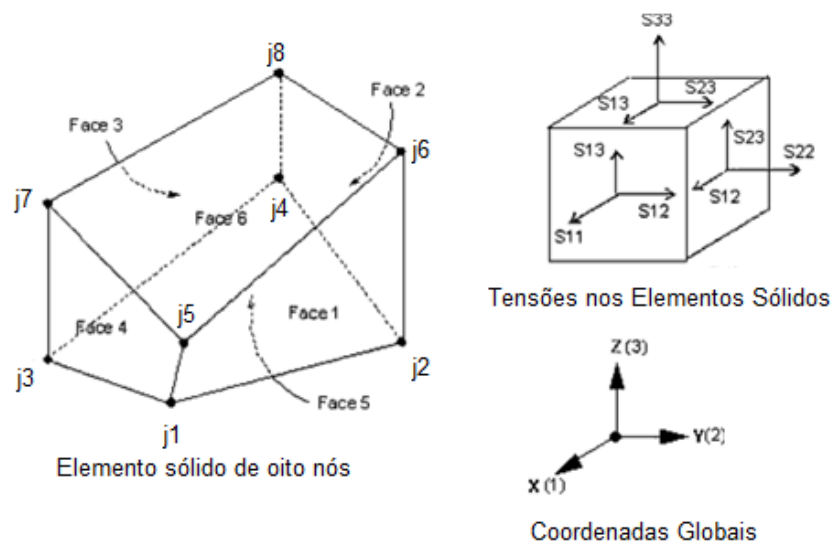
Figura 16 - Sistema de coordenadas locais dos elementos sólidos do SAP 2000
