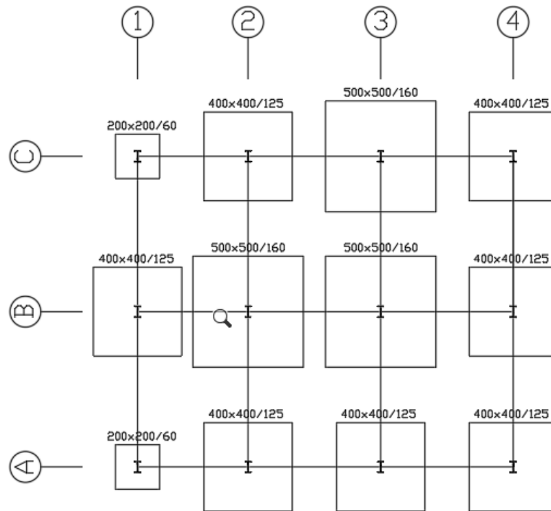
Figura 18 – Dimensões das sapatas (cm)
