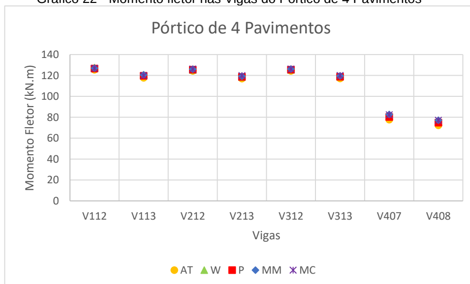
Gráfico 22 - Momento fletor nas Vigas do Pórtico de 4 Pavimentos
