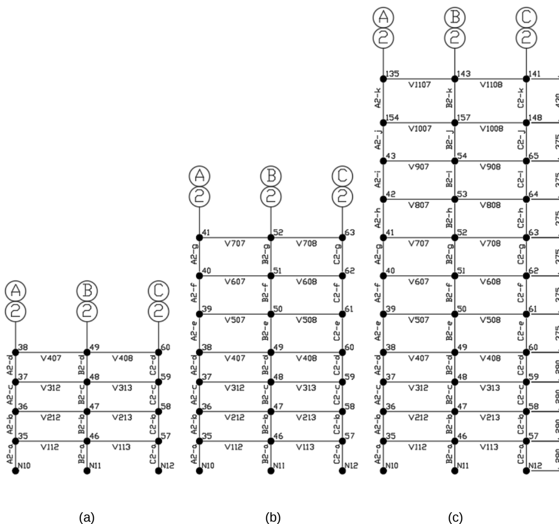
Figura 14 – Numeração das barras e nós do pórtico plano analisado por Siqueira (2019)
