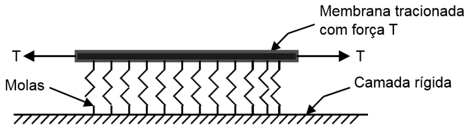
Figura 2 - Modelo de Filonenko-Borodich
