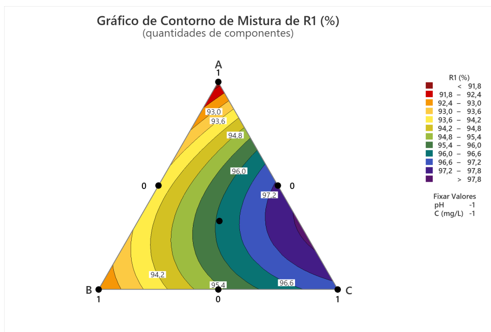
Figura 4.4 – Gráfico de contorno de misturas de R1, com pH e concentração no nível -1 (6 e 10 mg/L, respectivamente).
