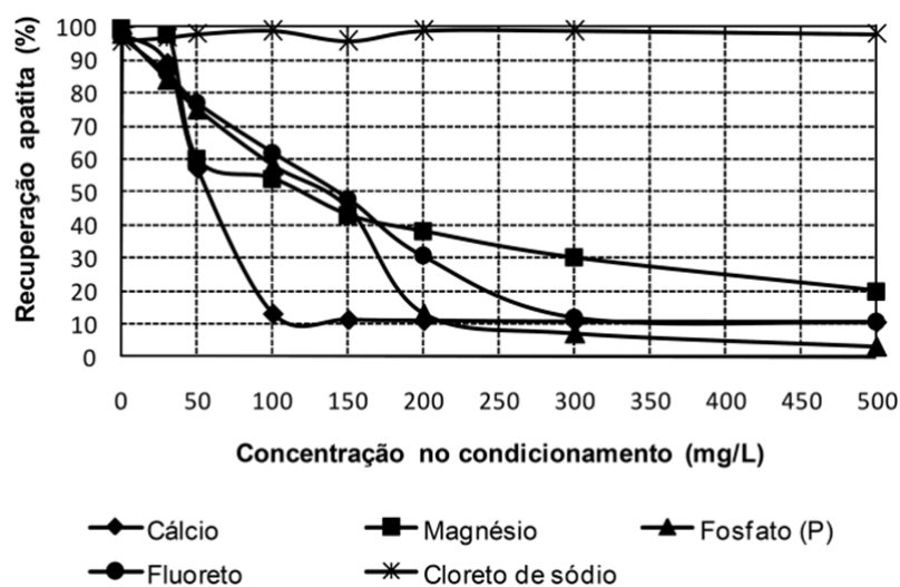
Figura 2.16 – Recuperação de apatita em relação a concentração dos íons determinantes de potencial.
