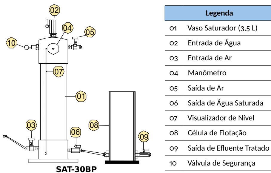
Figura 2.20 – Representação esquemática do equipamento de flotação por ar dissolvido.
