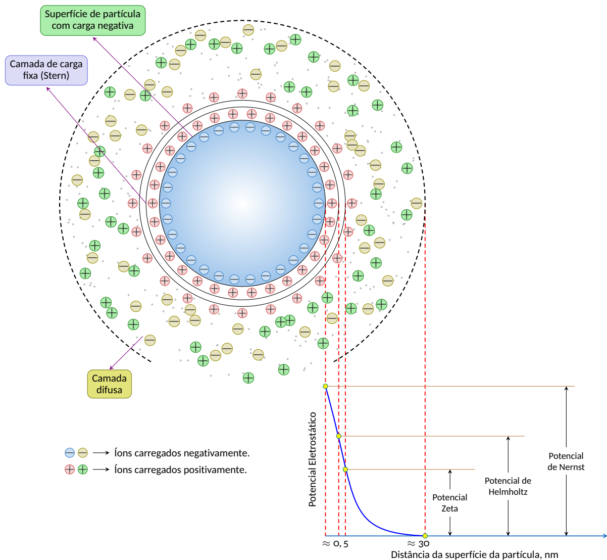
Figura 2.12 – Diagrama que representa uma partícula coloidal.
