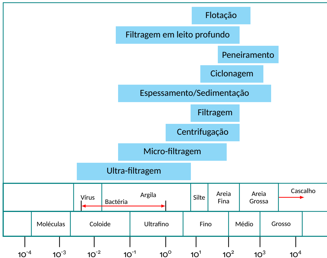
Figura 2.5 – Técnicas de separação sólido-líquido em função do tamanho de partícula ou micro-organismo.
