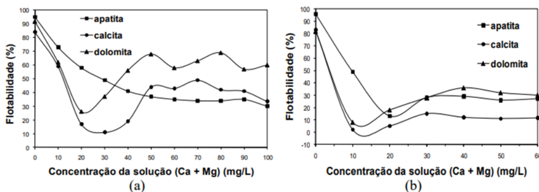
Figura 2.18 – Flotabilidade, em pH 8, dos minerais apatita, calcita e dolomita: (a) minério flogopitítico, polpa mineral com íons cálcio/magnésio na proporção de 1:1 e concentração de oleato de potássio de 13,34 mg/L e, (b) minério foscorítico, polpa mineral com íons cálcio/magnésio na proporção de 2:1 e concentração de oleato de potássio de 10,67 mg/L.
