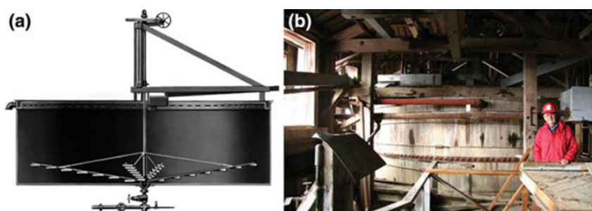
Figura 2.6 – O primeiro espessador. (a) Esquemático e (b) foto do espessador original de Dorr.
