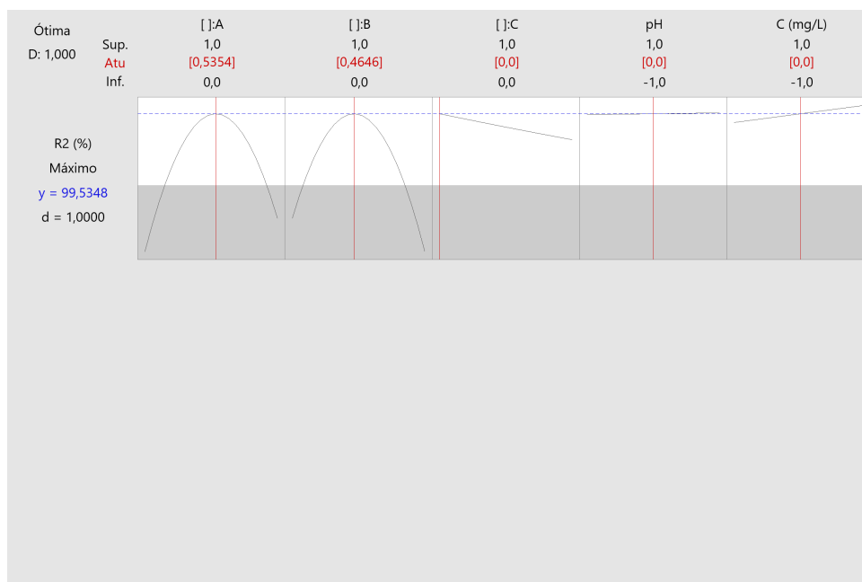
Figura 5.1 – Otimização da Resposta 2.
