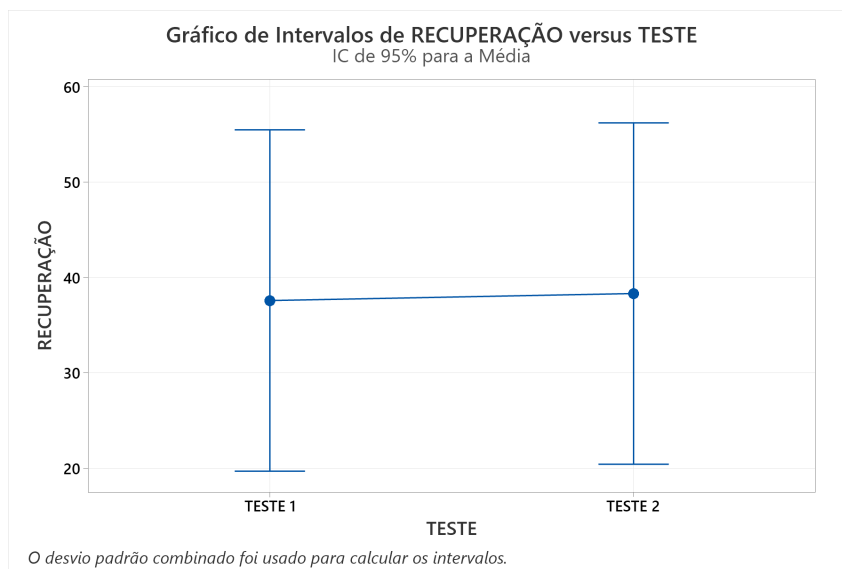
Figura 4.6 – Gráfico de intervalos dos testes de flotação após o tratamento da água do espessador.
