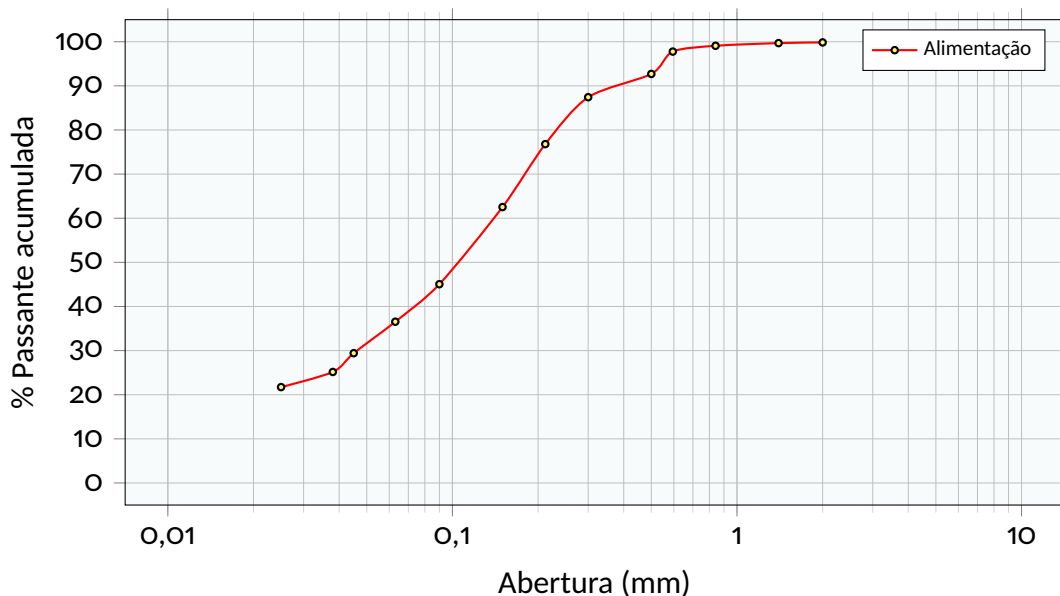
Figura 4.1 – Distribuição Granulométrica.
