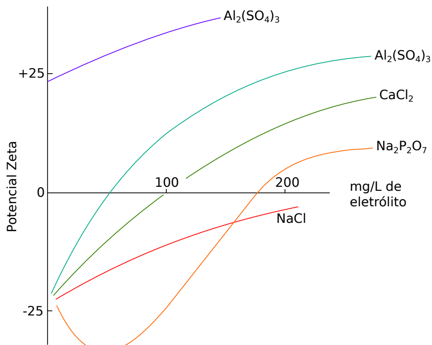
Figura 2.11 – Potencial zeta versus concentração de eletrólito.
