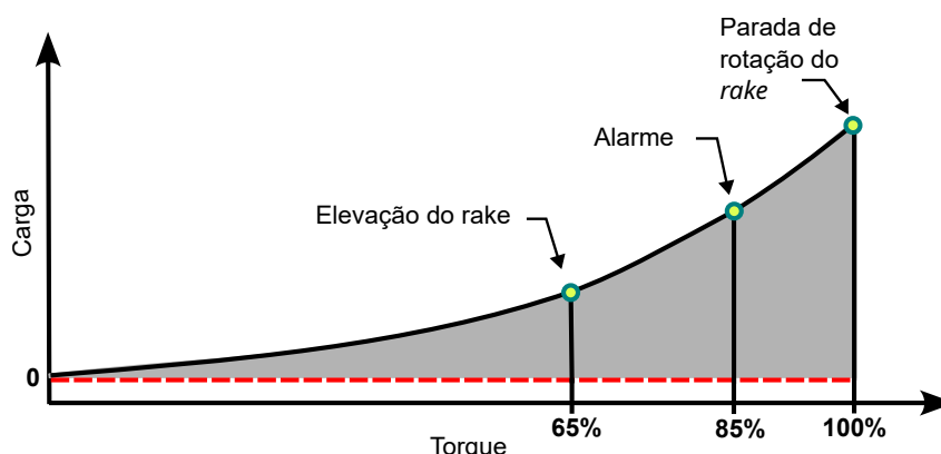
Figura 2.7 – Curva de variação do torque e medidas de segurança tomadas e circuito eletrônico para a operação dos rakes.
