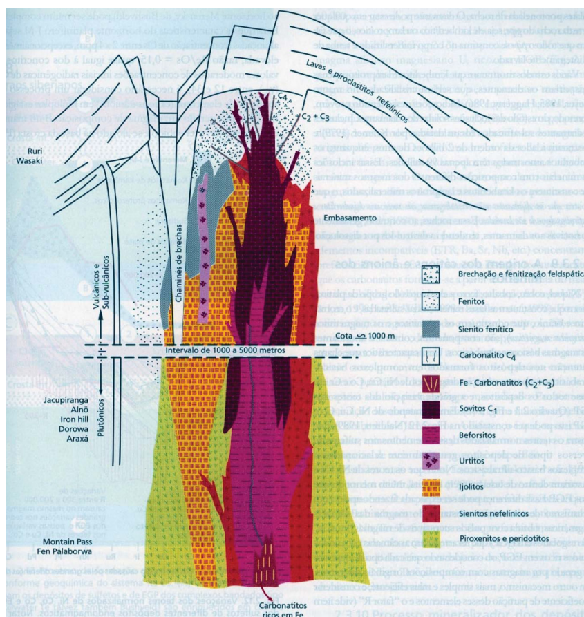
Figura 2.3 – Seção esquemática de um complexo alcalino-carbonatítico mostrando a distribuição dos litotipos e as principais mineralizações a eles associados.
