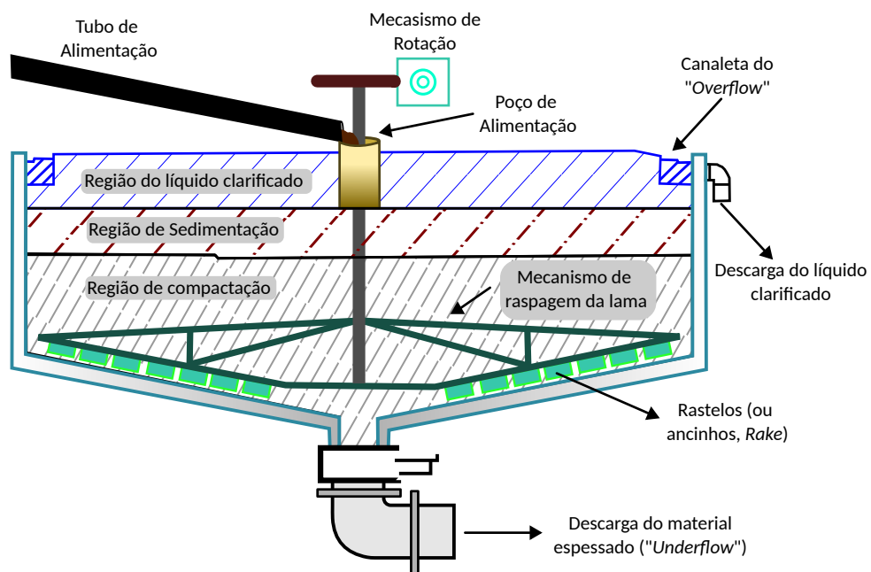
Figura 2.9 – Vista lateral de um espessador convencional.
