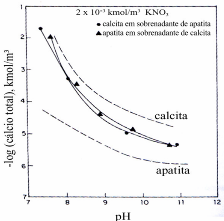
Figura 2.15 – Solubilidade de calcita e apatita em água (linha tracejada) e em soluções sobrenadantes (linha cheia).
