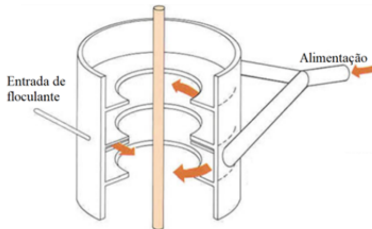
Figura 2.8 – Poço de alimentação com suas entradas tangenciais e defletores internos.
