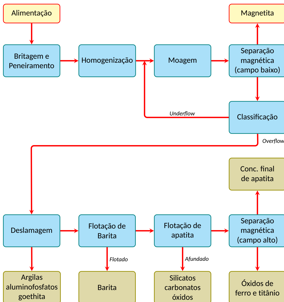
Figura 2.4 – Beneficiamento de minério fosfático.
