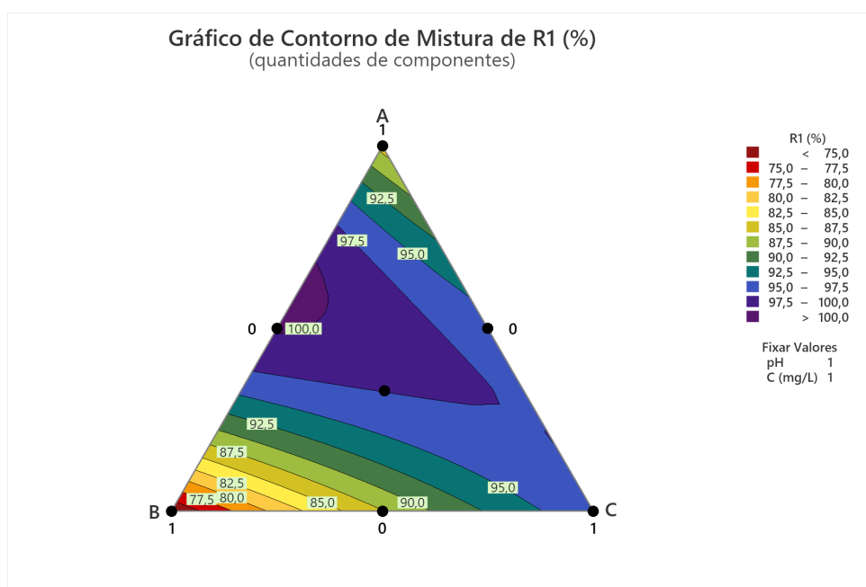
Figura 4.5 – Gráfico de contorno de misturas de R1, com pH e concentração no nível +1 (8 e 50 mg/L, respectivamente).
