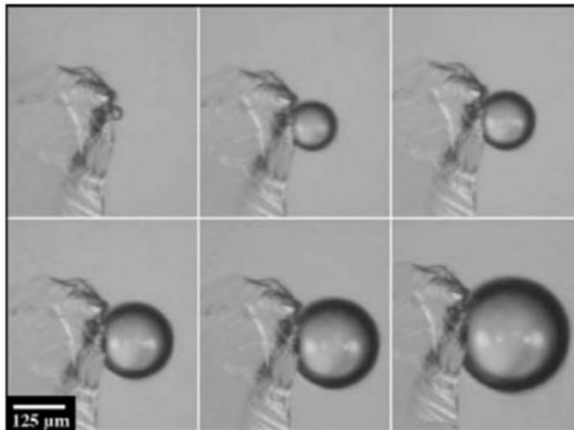
Figura 2.21 – Nucleação e crescimento de uma microbolha na superfície de uma partícula de quartzo hidrofobizada.
