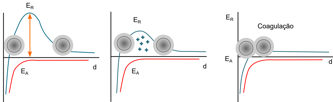
Figura 2.10 – Mecanismo simplificado de Coagulação. E_R = Energia de repulsão; E_A = Energia de atração.
