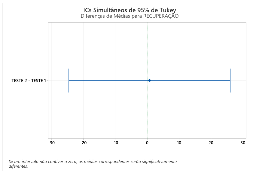
Figura 4.7 – Gráfico de ICs Simultâneos.
