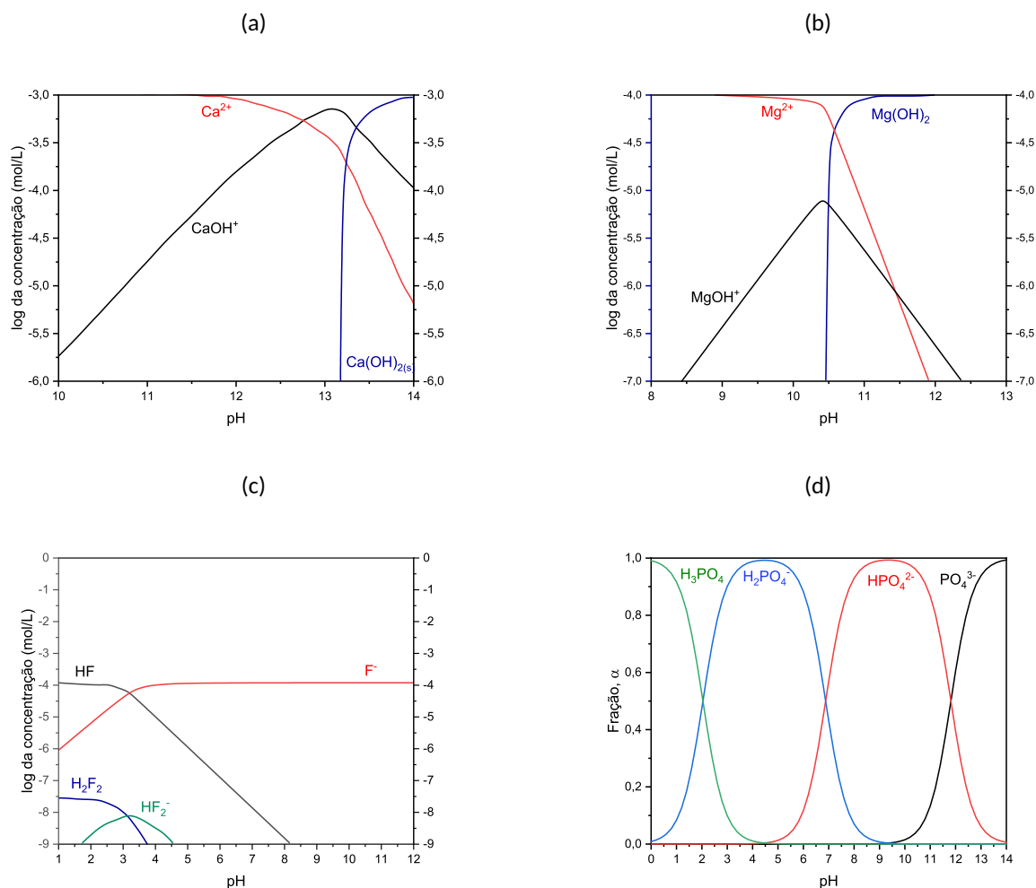
Figura 2.17 – Diagramas de concentração logarítmica: (a) para 1 \times 10^{-3} mol/L de cálcio; (b) para 1 \times 10^{-4} mol/L de magnésio; (c) para 1 \times 10^{-4} mol/L de fluoreto e (d) diagrama de distribuição de espécie para 1 \times 10^{-3} mol/L de fosfato.
