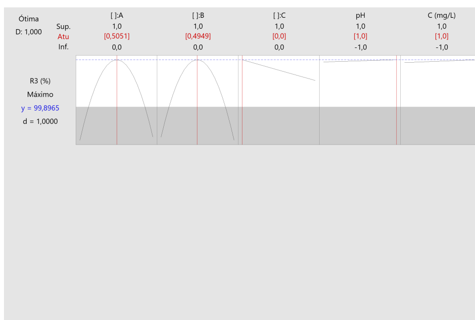
Figura 5.2 – Otimização da Resposta 3.
