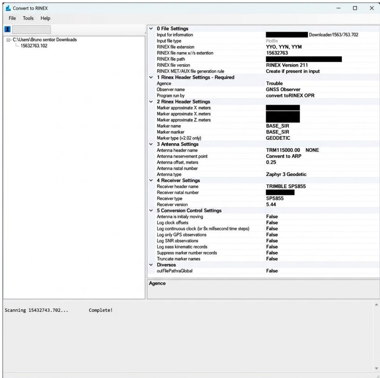
Figura 22 - Software de conversão de arquivos Trimble GNSS.
