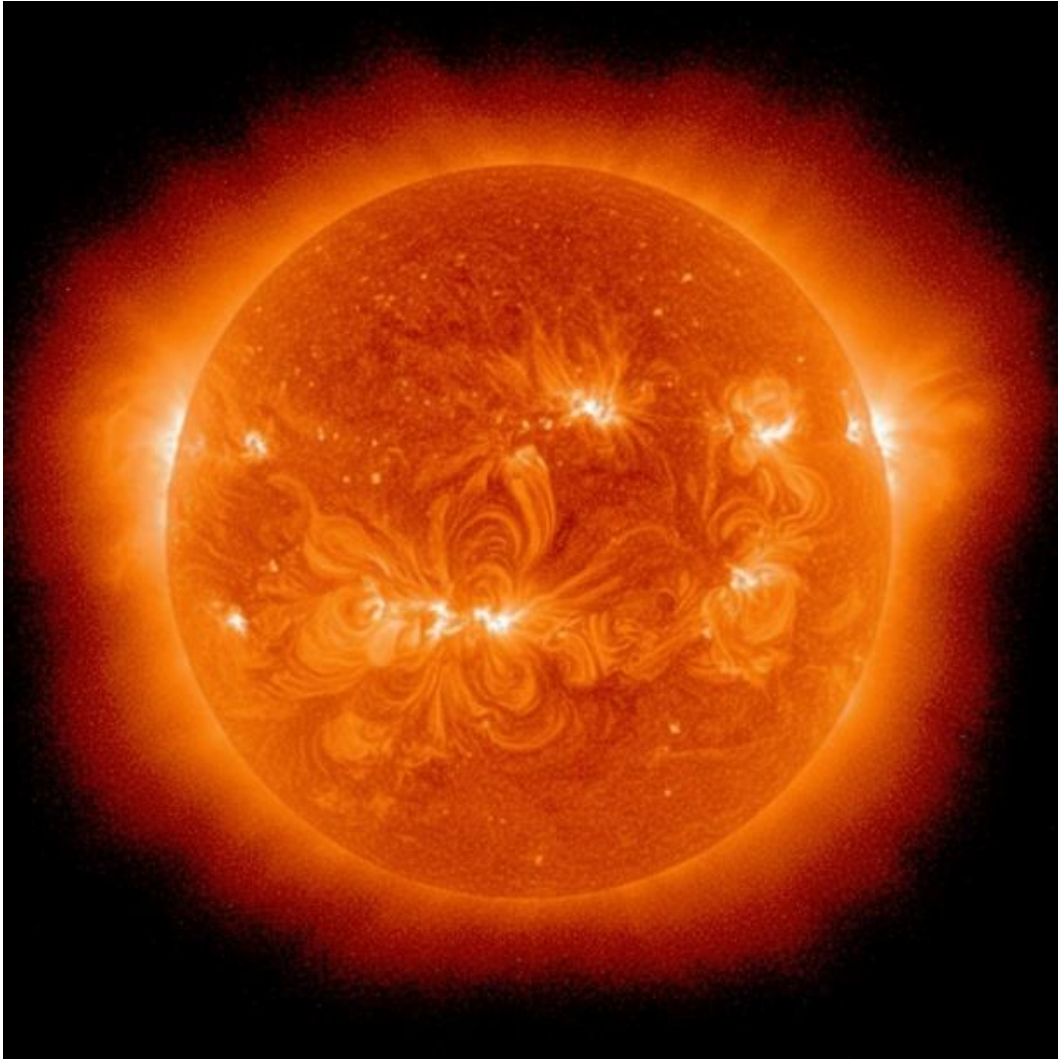
Figura 3 - Exemplo de buraco coronal, que aparece na imagem como região mais escura.
