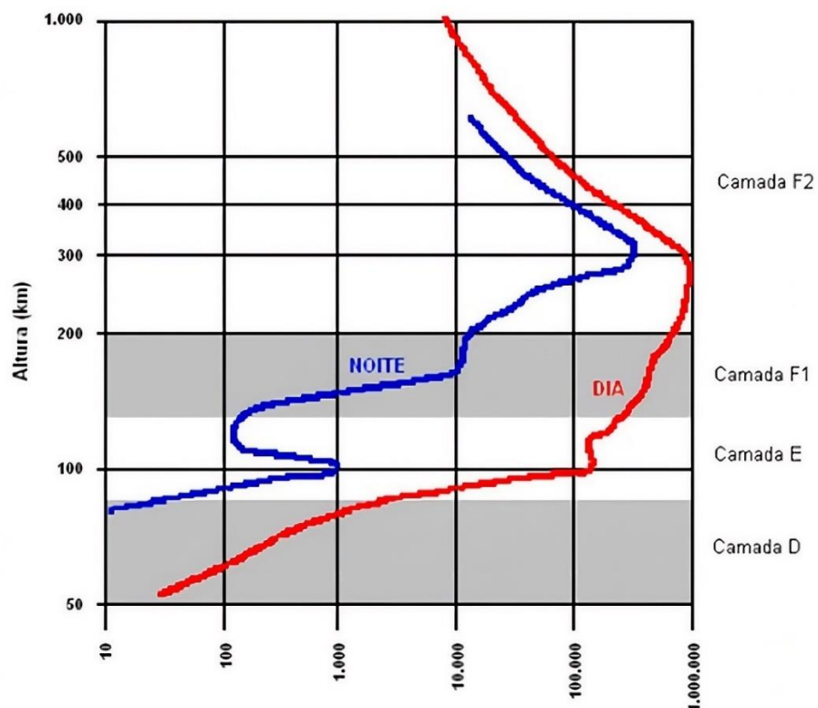
Figura 2 - Divisão da ionosfera em camadas.
