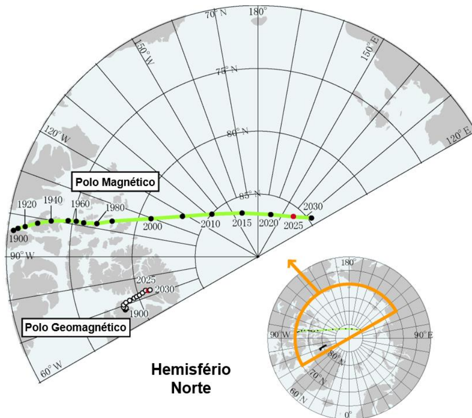
Figura 10 - Variação dos polos magnéticos e geomagnético no hemisfério Norte.
