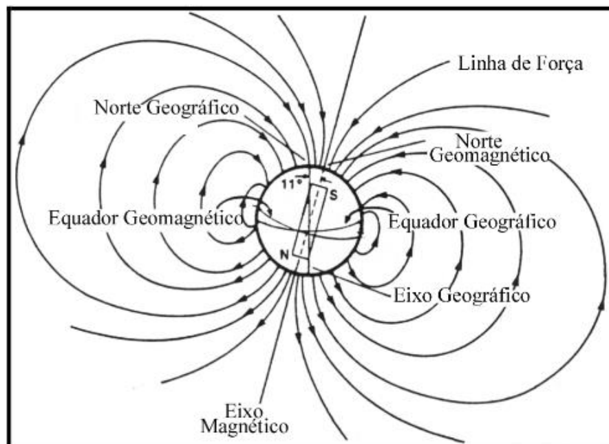
Figura 4 - Estrutura do campo magnético da Terra.
