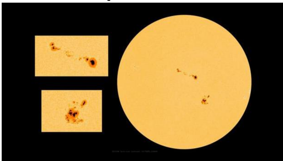
Figura 25 - Manchas solares.
