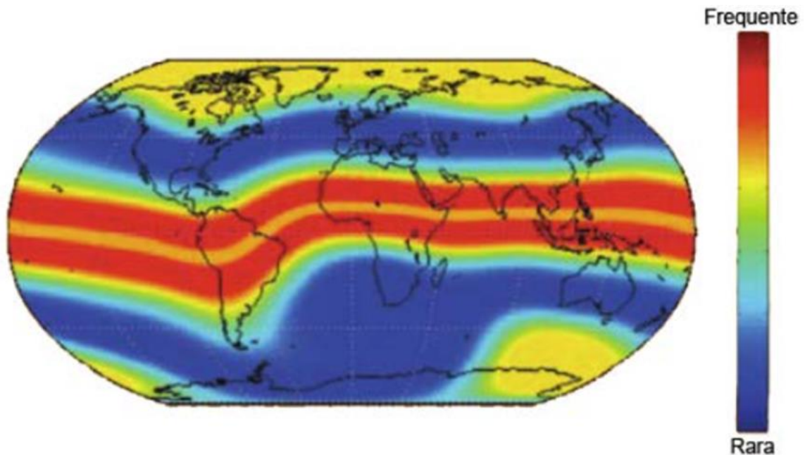
Figura 13 - Frequência de ocorrência de cintilação de acordo com a localização geográfica.
