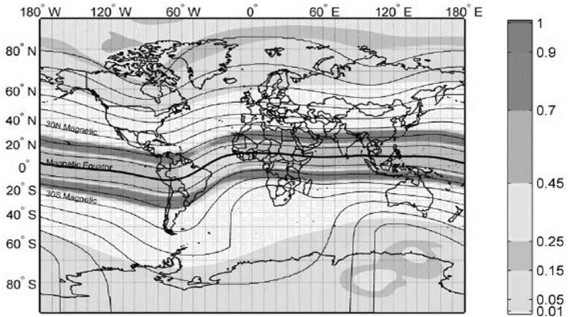
Figura 15 - Distribuição global do índice S4 em 15 de setembro de 2000 às 21h local.
