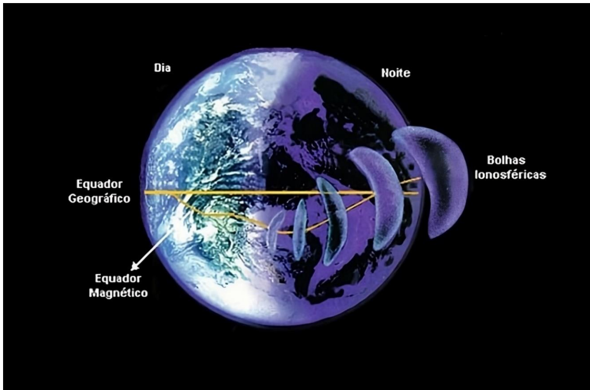
Figura 11 - Comportamento temporal e espacial das irregularidades ionosféricas.
