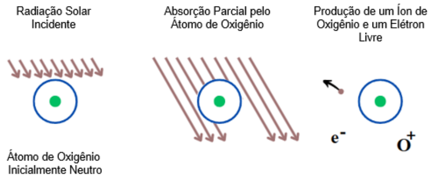
Figura 1 - Fotoionização.
