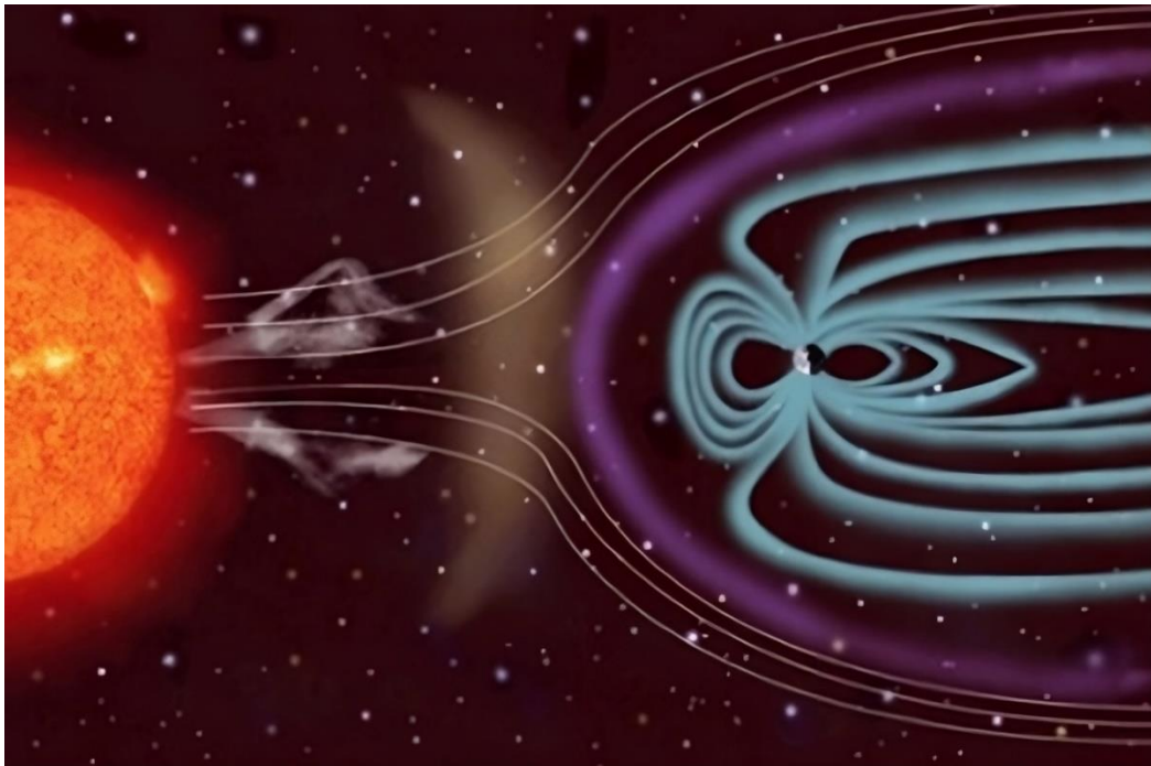
Figura 6 - Influência do vento solar no campo geomagnético.
