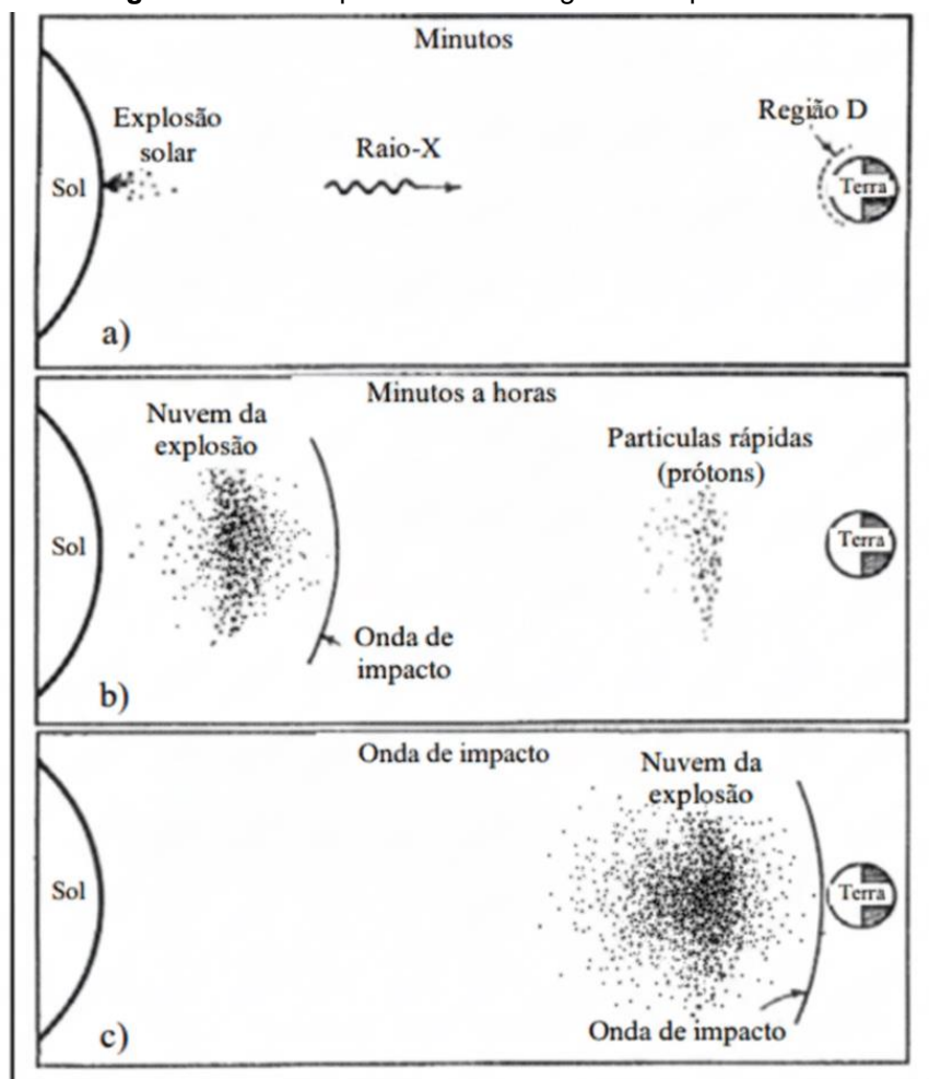
Figura 8 – Consequências de uma grande explosão solar.
