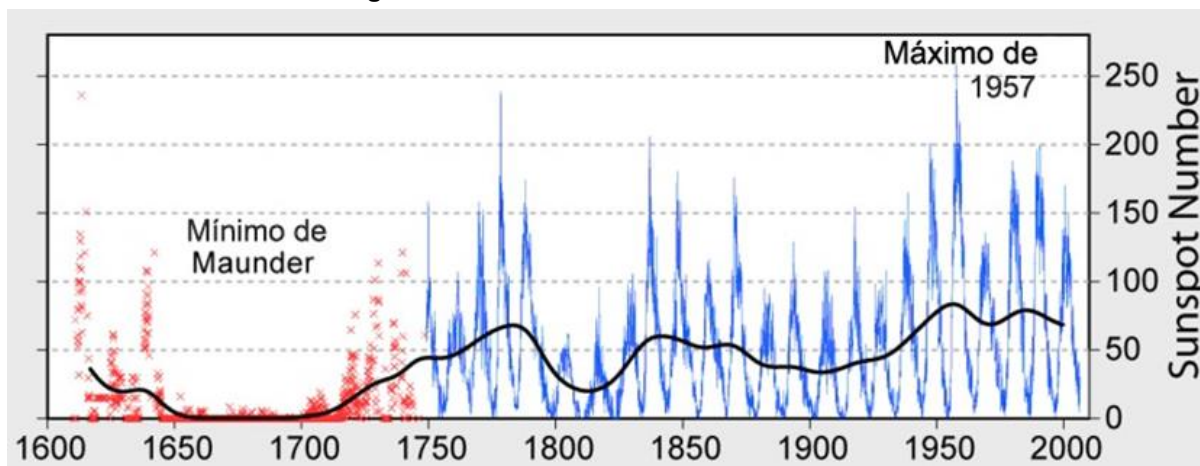
Figura 26 - Manchas solares entre 400 anos.
