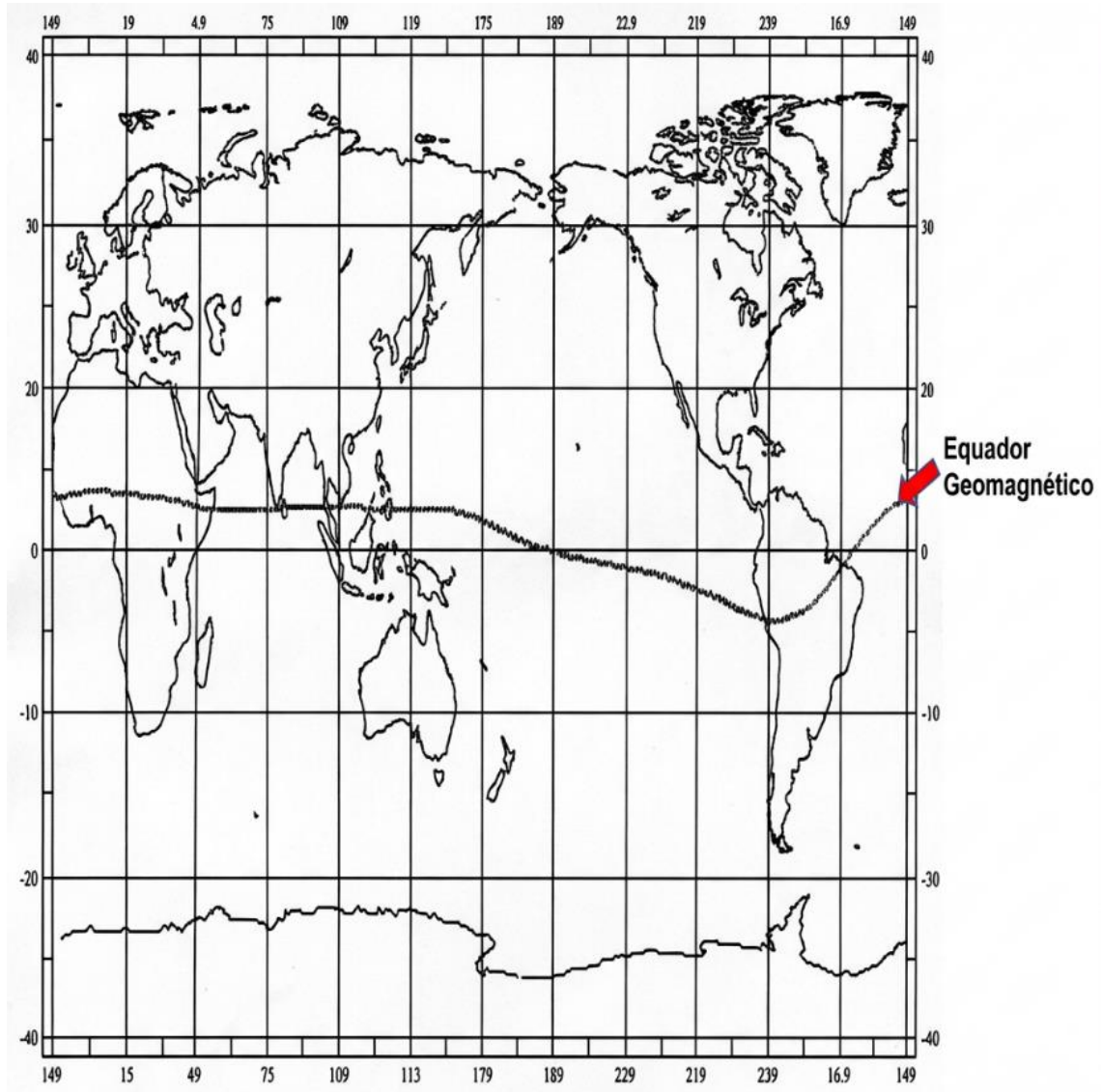
Figura 5- Equador geomagnético no hemisfério Norte no ano de 2020.
