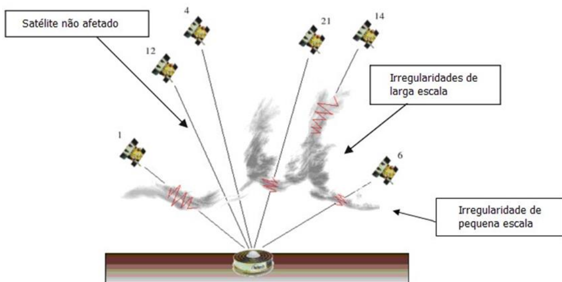
Figura 12 - Esquematisação da cintilação nos sinais GNSS.
