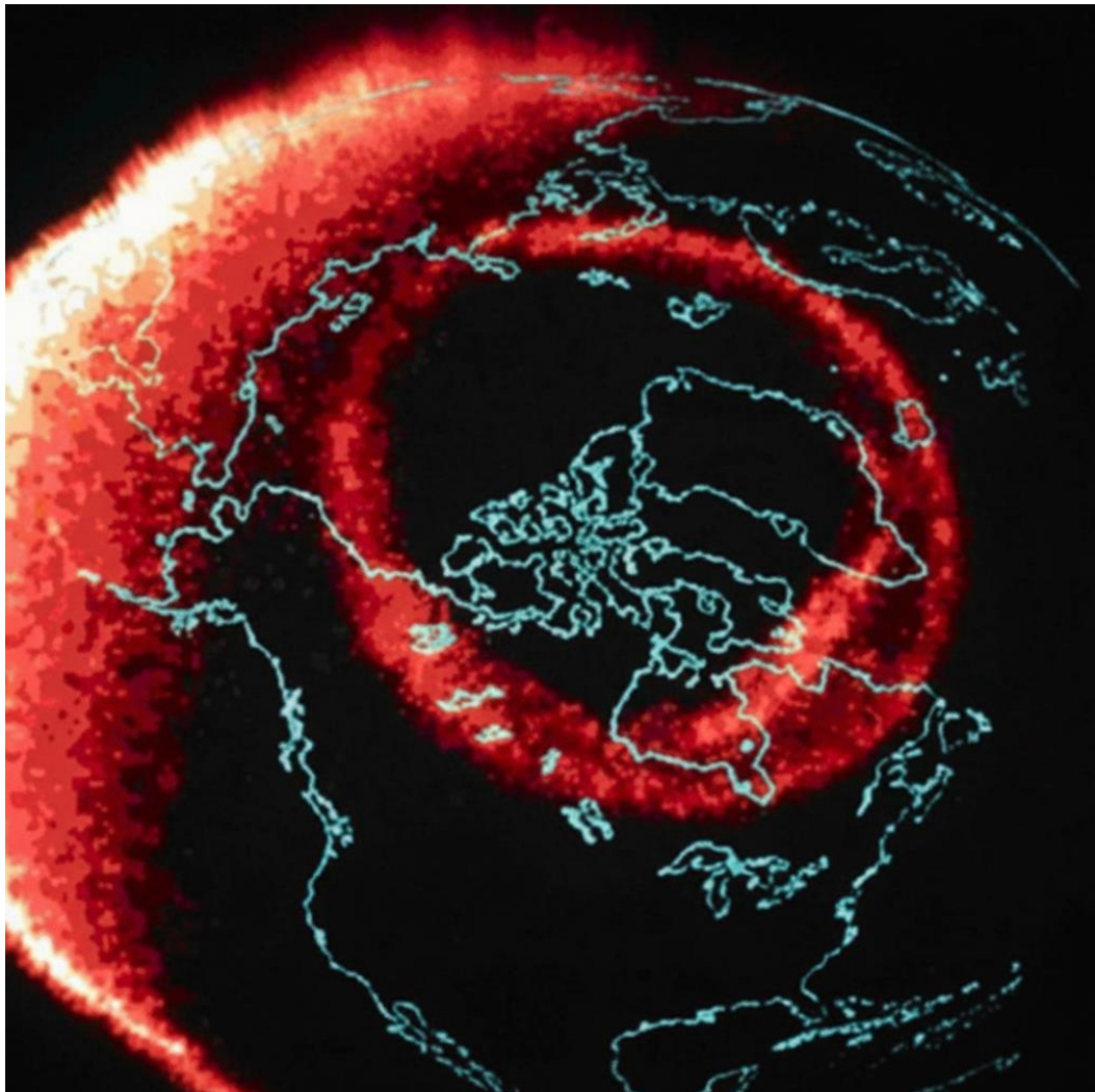
Figura 14 - Oval auroral sobre a América do Norte.
