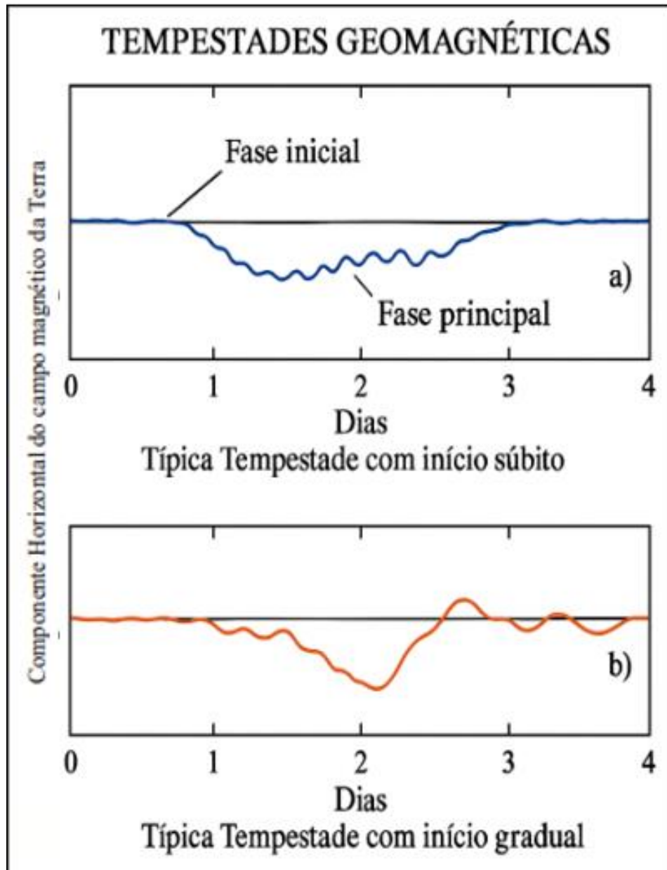
Figura 7- Tempestades com início súbito e gradual.
