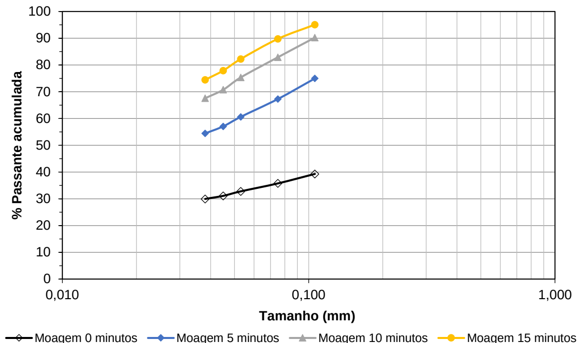
Figura 13 – Curvas de distribuição granulométrica do KF em diferentes tempos de moagem.
