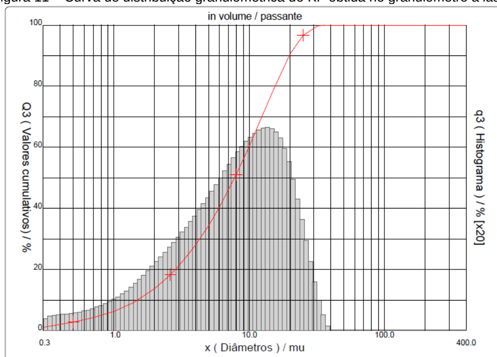
Figura 11 – Curva de distribuição granulométrica do KF obtida no granulômetro a laser .
