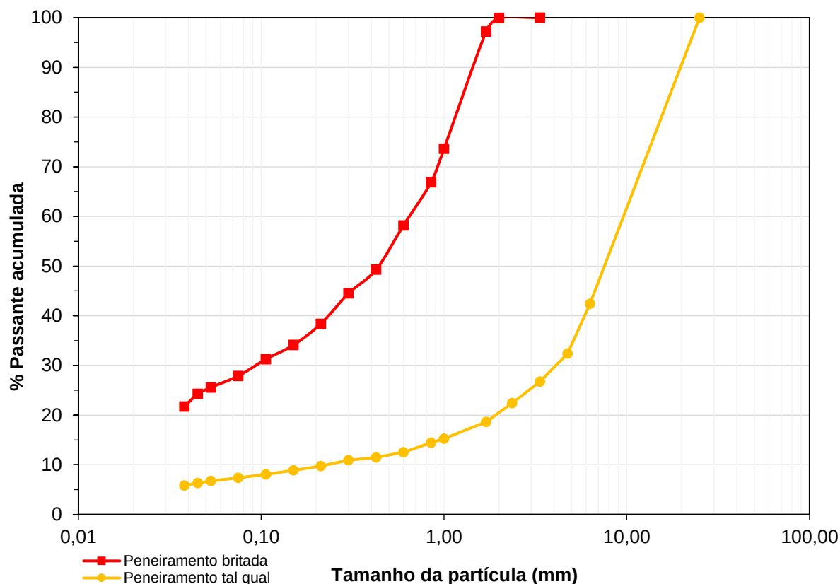
Figura 10 – Curva de distribuição granulométrica da amostra KF tal qual (amarela) e britada (vermelho).
