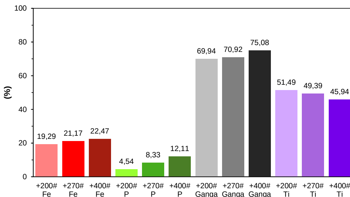
Figura 33 – Diagrama de porcentagem de grãos liberados da classe >90\% por composição de partícula para as frações +200#, +270# e +400# do KF referente aos grupos dos minerais de ferro, fósforo, titânio e ganga.
