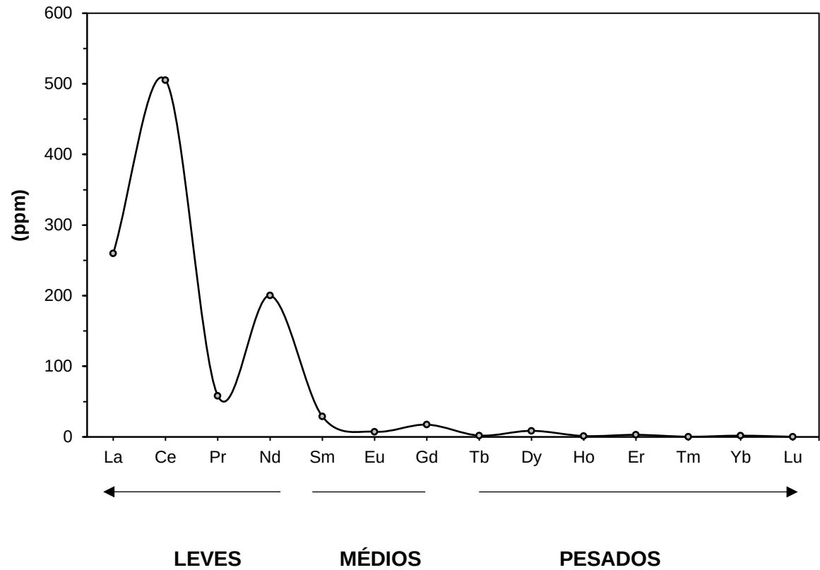
Figura 17 – Composição química de ETRs da amostra cabeça do KF.
