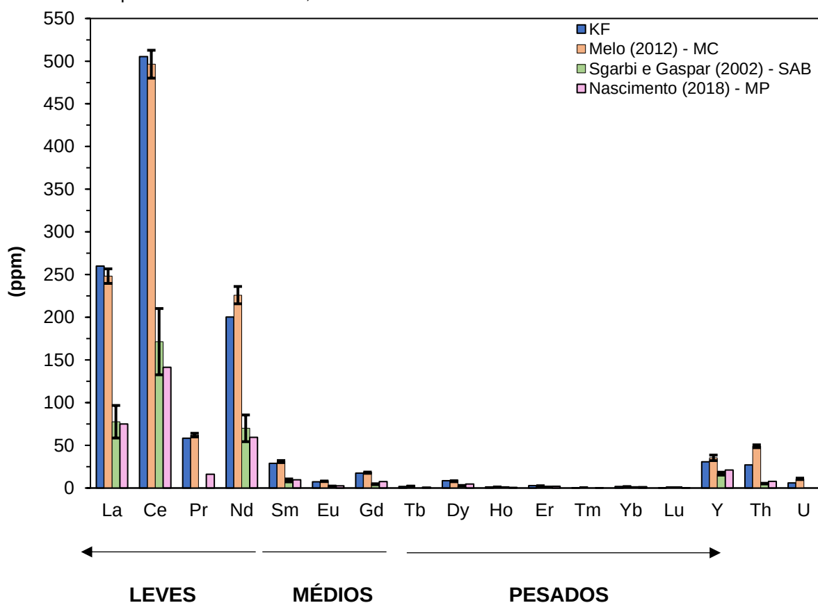
Figura 19 – Comparação da composição química dos ETRs do KF em relação a outros kamafugitos. MC: Grupo Mata da Corda-MG, SAB: Santo Antônio da Barra-GO e MP: Morro Preto-GO.
