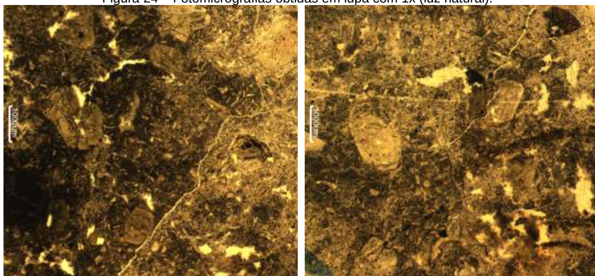
Figura 24 – Fotomicrografias obtidas em lupa com 1x (luz natural).
