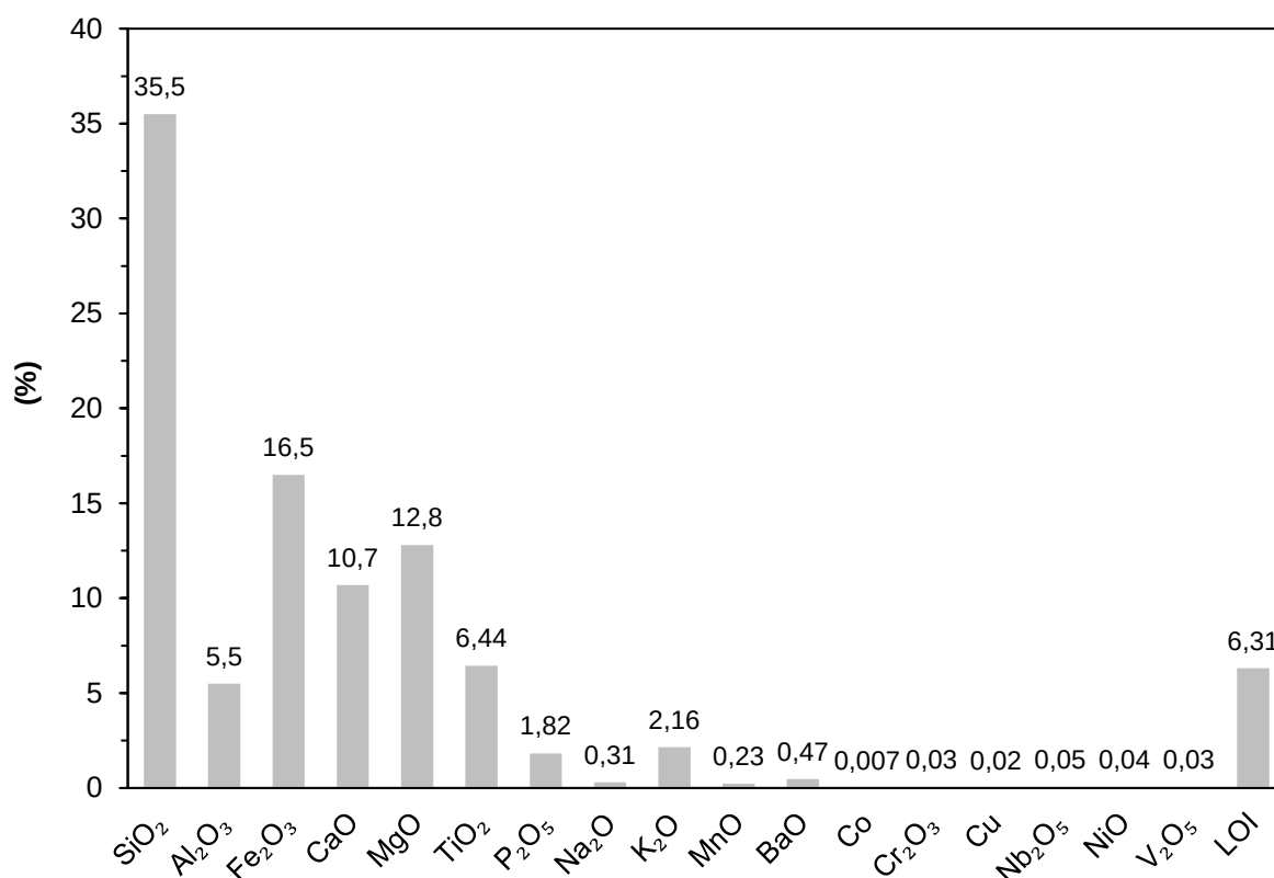
Figura 14 – Composição química de óxidos majoritários e LOI da amostra cabeça do KF.
