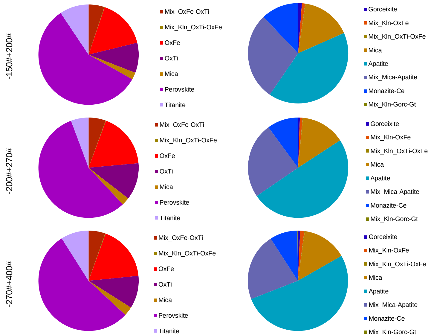
Figura 29 – Distribuição do titânio (à esquerda) e do fósforo (à direita) nas frações +200#, +270# e +400# da amostra KF.
