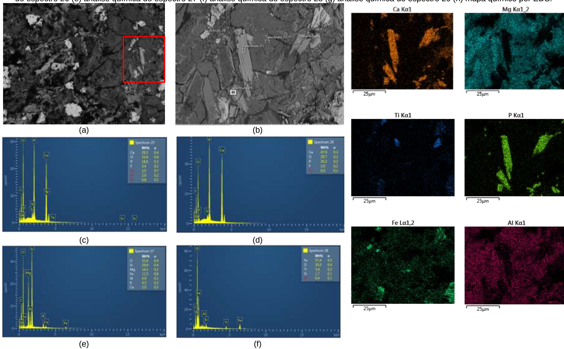
Figura 26 – Imagens de MEV-EDS (a) Região com os minerais analisados (b) Pontos de espectro EDS (c) análise química do espectro 25 (d) análise química do espectro 26 (e) análise química do espectro 27 (f) análise química do espectro 28 (g) análise química do espectro 29 (h) mapa químico por EDS.
