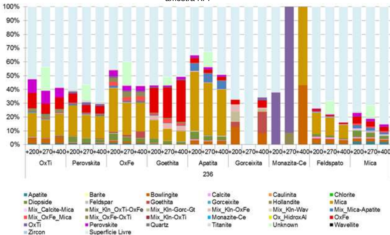
Figura 31 – Associação dos minerais em partículas livres (azul claro) e associados a outras fases na amostra KF.
