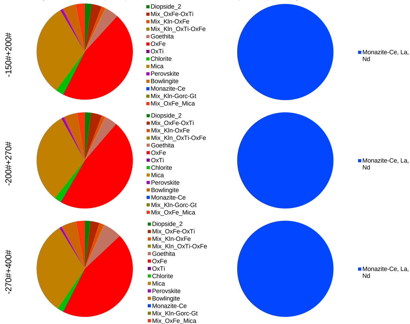
Figura 30 – Distribuição do ferro (à esquerda) e do cério, lantânio e neodímio (à direita) nas frações +200#, +270# e +400# da amostra KF.
