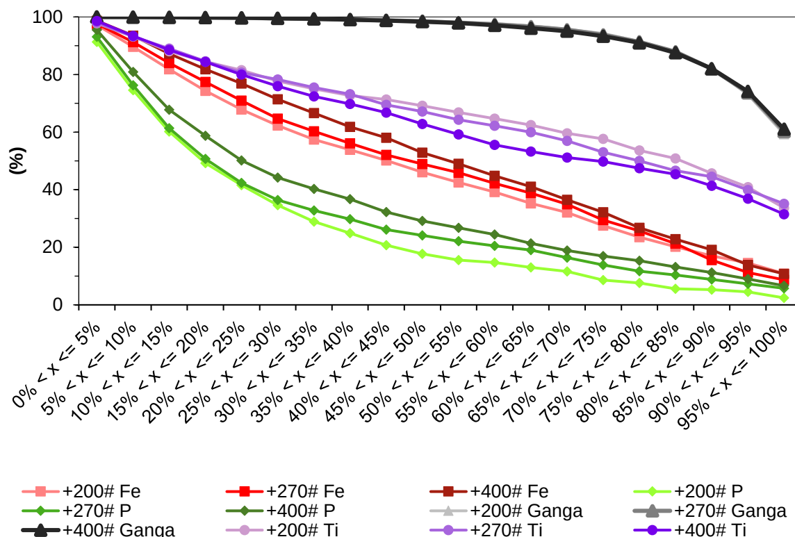
Figura 34 – Diagrama acumulado de liberação mineral por superfície livre obtido para as frações +200#, +270# e +400# do KF referente aos grupos dos minerais de ferro, fósforo, titânio e ganga.
