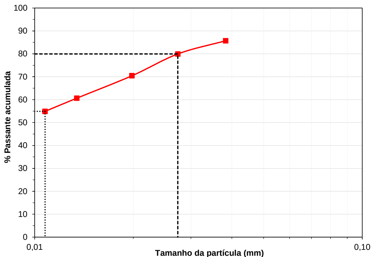
Figura 12 – Curva de distribuição granulométrica do KF obtida no cyclosizer .
