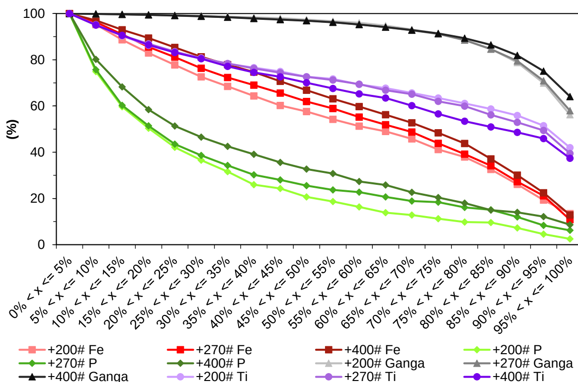
Figura 32 – Diagrama acumulado de liberação mineral por composição de partícula obtido para as frações +200#, +270# e +400# do KF referente aos grupos dos minerais de ferro, fósforo, titânio e ganga.
