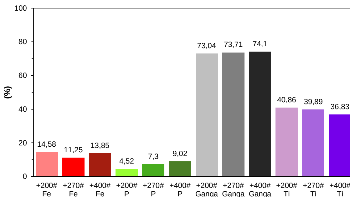
Figura 35 – Diagrama de porcentagem de grãos liberados da classe > 90% por superfície livre para as frações +200#, +270# e +400# do KF referente aos grupos dos minerais de ferro, fósforo, titânio e ganga.
