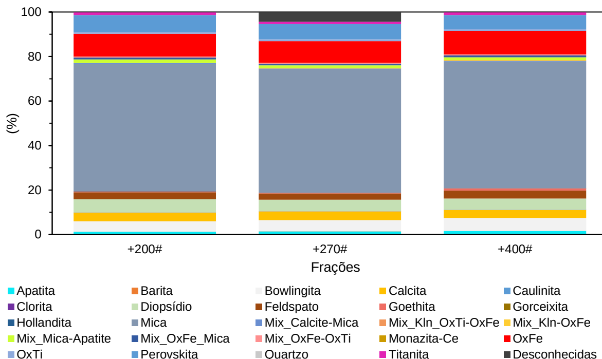
Figura 28 – Proporção dos minerais nas frações +200#, +270# e +400# no litotipo KF (% peso).
