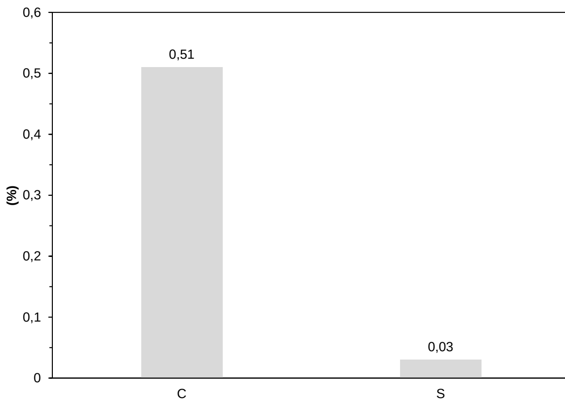
Figura 22 – Composição química de carbono e enxofre da amostra cabeça referente ao KF.
