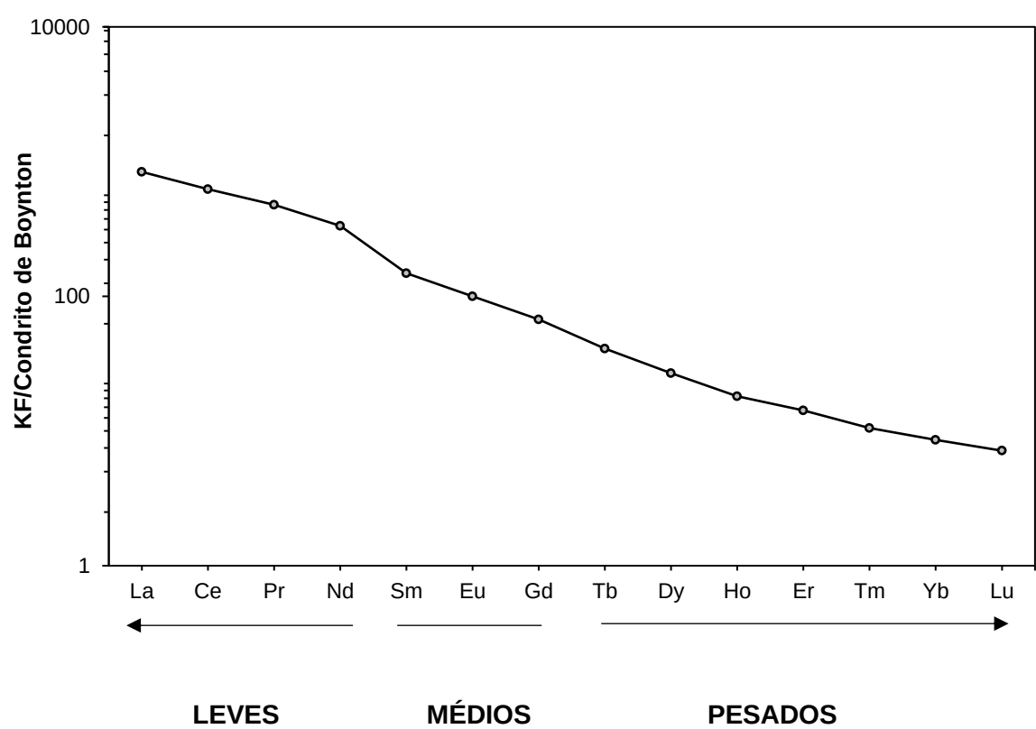
Figura 18 – Padrão de ETRs normalizado pelo condrito de Boynton (1984).
