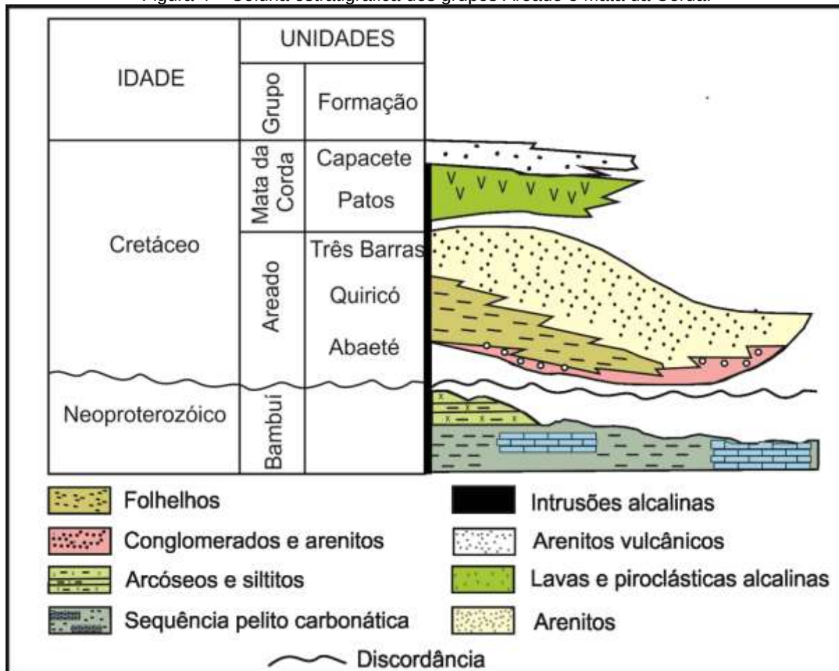
Figura 4 – Coluna estratigráfica dos grupos Areado e Mata da Corda.
