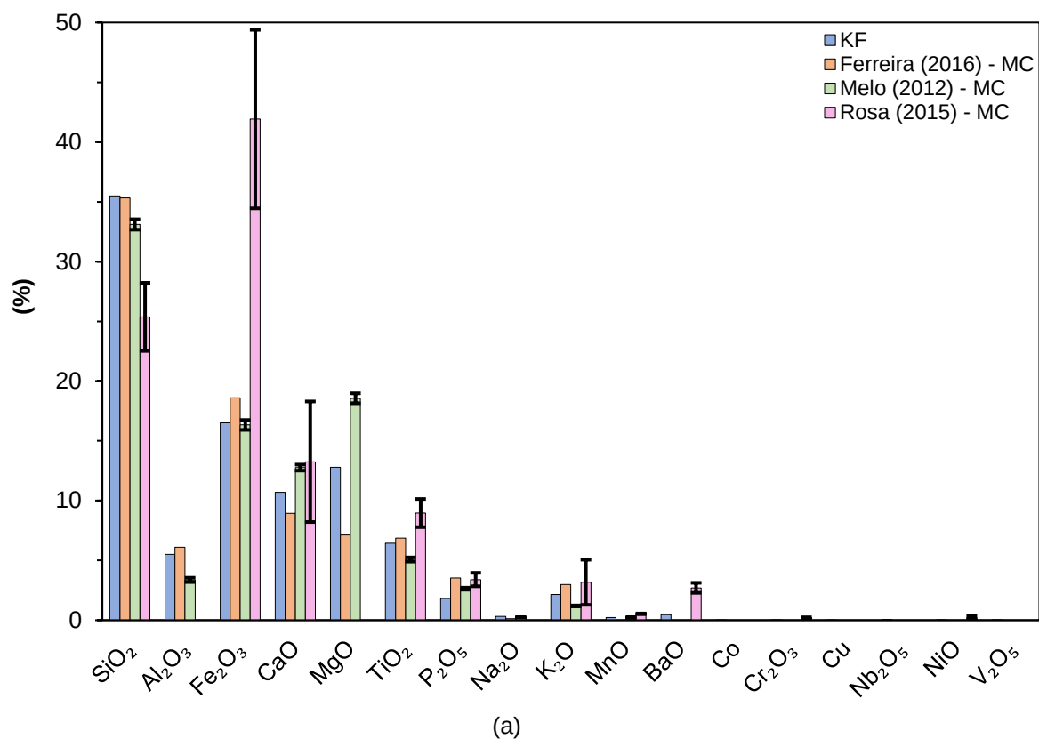
Figura 15 – Comparação da composição química dos óxidos majoritários do KF em relação a outros kamafugitos (a) MC: Grupo Mata da Corda-MG (b) SAB: Santo Antônio da Barra-GO e MP: Morro Preto-GO (c) de outras regiões (África, Itália).
