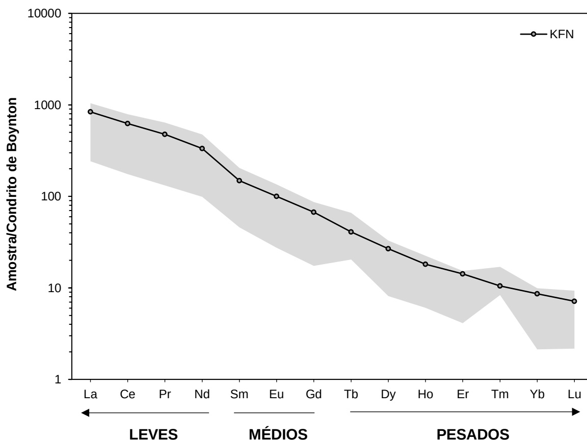
Figura 20 – Comparação entre o padrão de ETRs do KF normalizado (KFN) pelo condrito de Boynton (1984) em relação aos dados máximos e mínimos de ETRs normalizados pelo condrito de Boynton (1984) de kamafugitos brasileiros.
