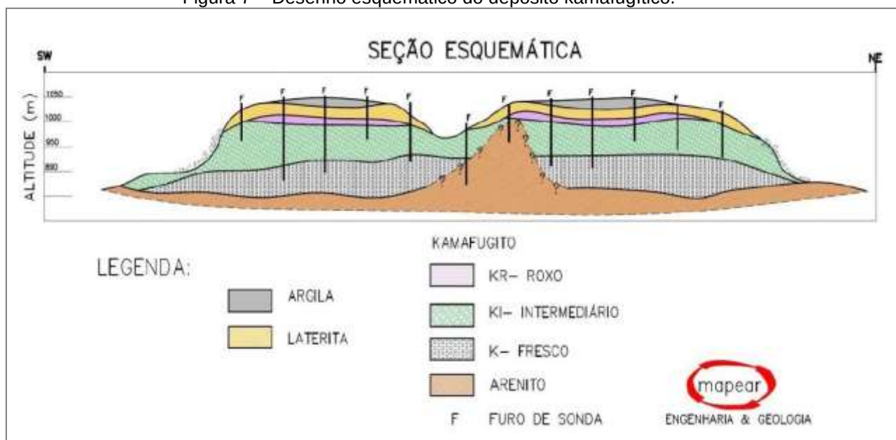
Figura 7 – Desenho esquemático do depósito kamafugítico.
