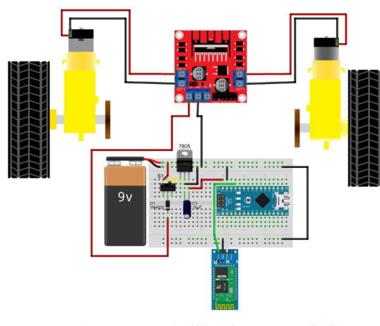
Figura 7.8: Conexão da ponte com motores e fonte [21]
