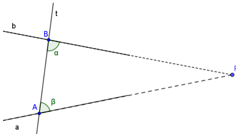
Figura 5 - Retas concorrentes
