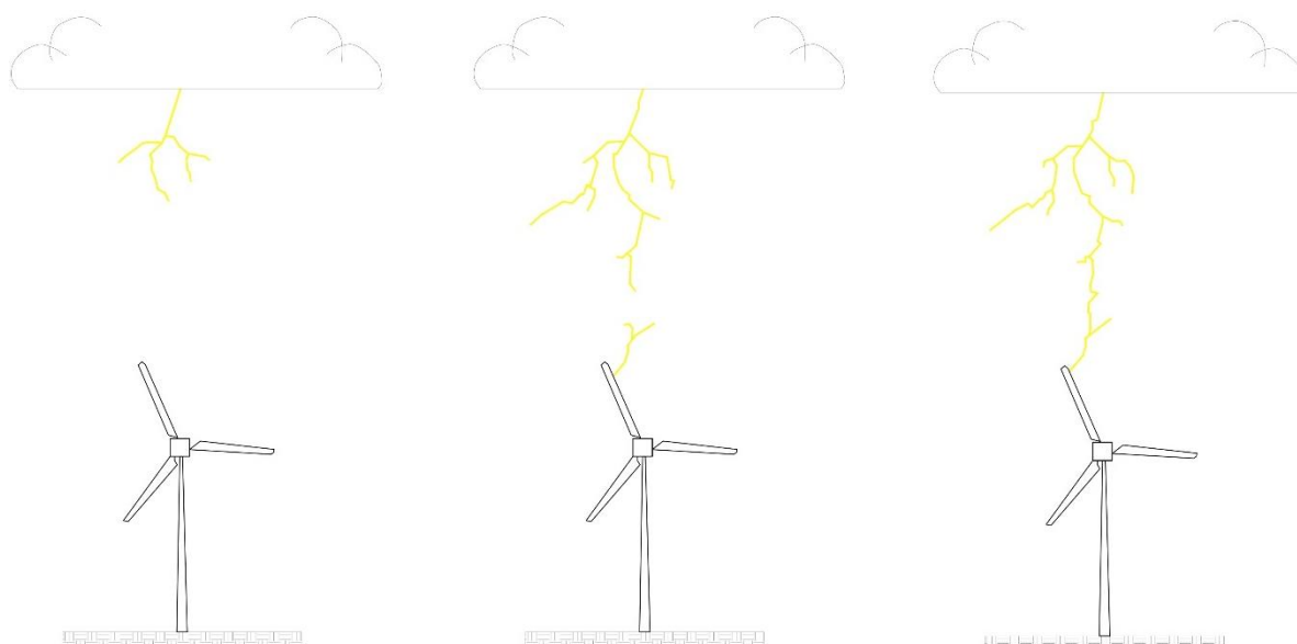
Figura 2.3 Processo de conexão entre o canal descendente (base da nuvem) e ascendente (estrutura aterrada).
