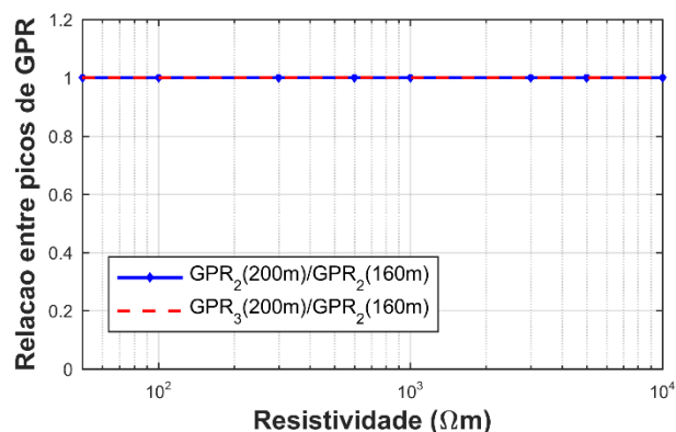
(c) GPR_2(200m)/GPR_2(160m) e GPR_3(200m)/GPR_2(160m)
