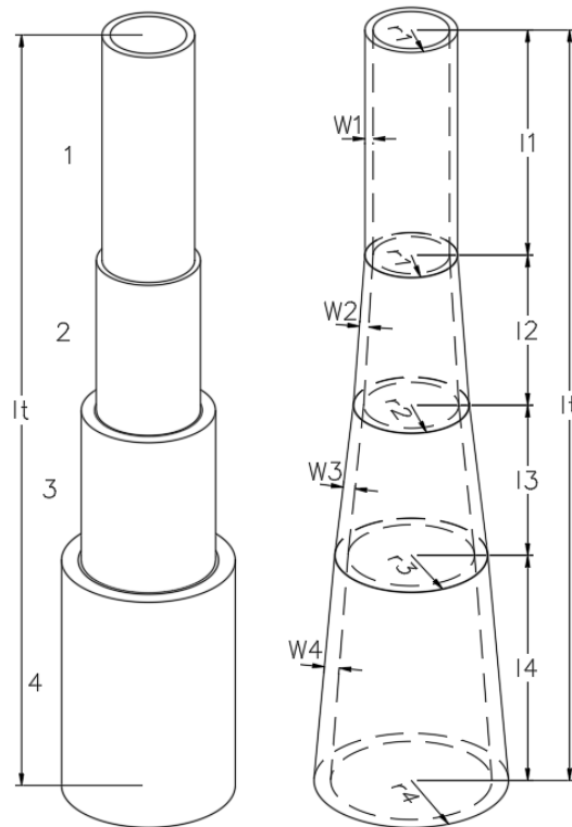
Figura 2.12 Modelo da torre da turbina eólica.
