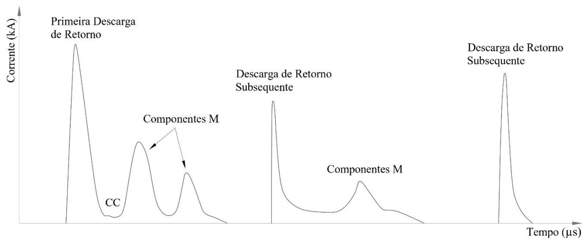
Figura 2.4 Representação estilizada da forma de onda de corrente associada com uma descarga descendente – Adaptado de [11].
