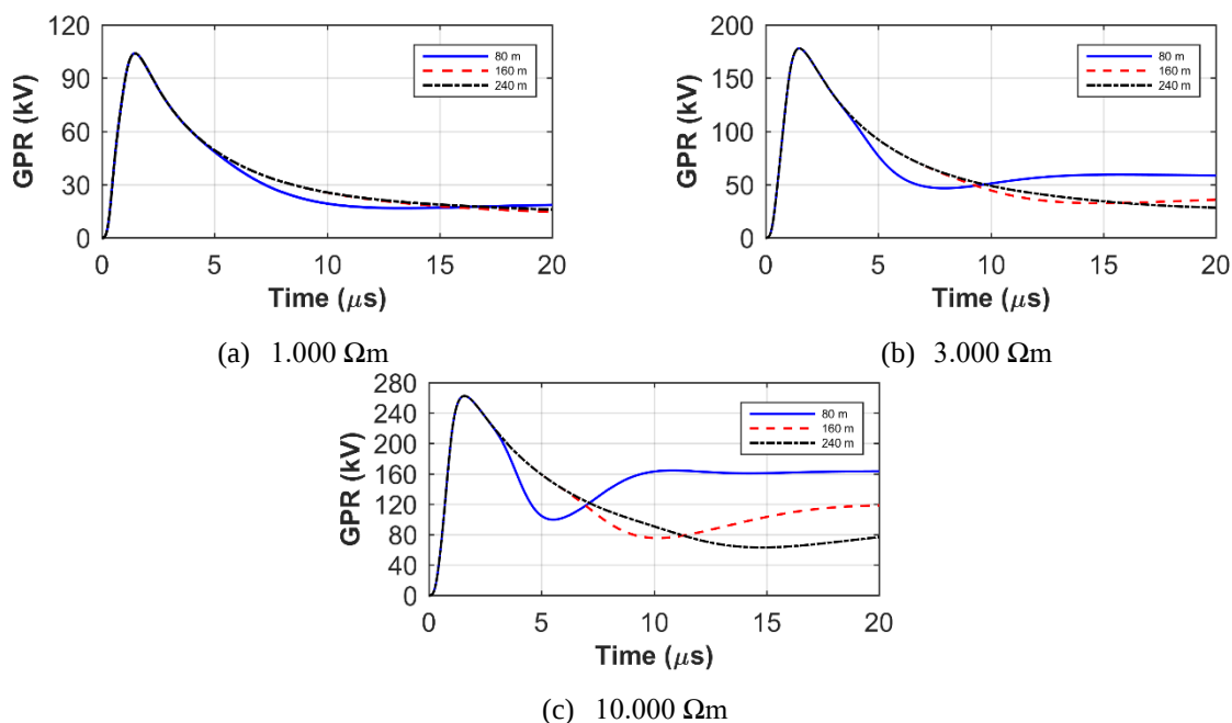
Figura 3.7 GPRs desenvolvidos em resposta a correntes representativas de descargas subsequentes associada às descendentes negativas e associada às ascendentes negativas (a) 1.000 Ωm, (b) 3.000 Ωm, (c) 10.000 Ωm.
