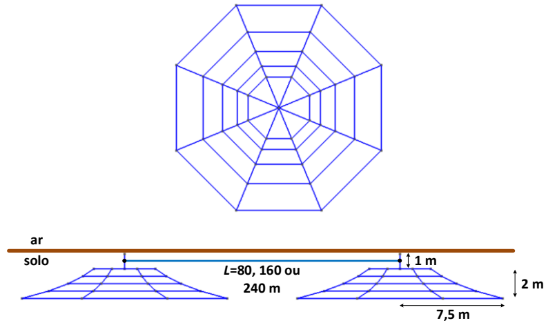
Figura 3. 1 (a) Sistema de aterramento de cada turbina eólica individual (vista superior), e (b) sistema de aterramento interligado (vista lateral).
