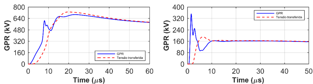
(a) \rho = 10.000 \Omega m e L = 80 m
