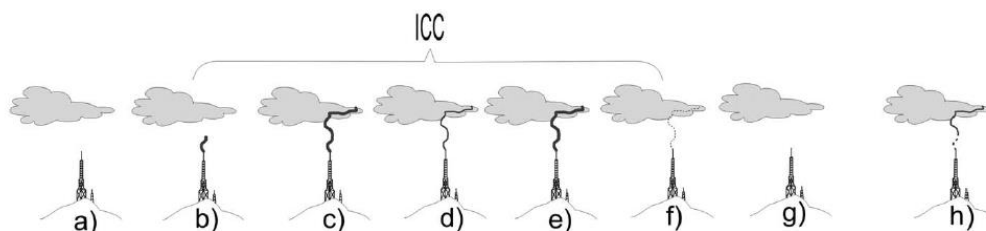
Figura 2.5 Estágios da descarga ascendente: (a) atividade anterior intra-nuvem (b) início de ICC na descarga nuvem-solo; (c) canal completo ascendente até a nuvem; (d) diminuição da luminosidade ou intensidade da corrente; (e) pulso de ICC intensificam a luminosidade do canal; (f) diminui a luminosidade do canal, fim de ICC; (g) cessa o fluxo de corrente ou luminosidade do canal; (h) a corrente de retorno utilizando o canal formado anteriormente pode acontecer. Retirado de [20].
