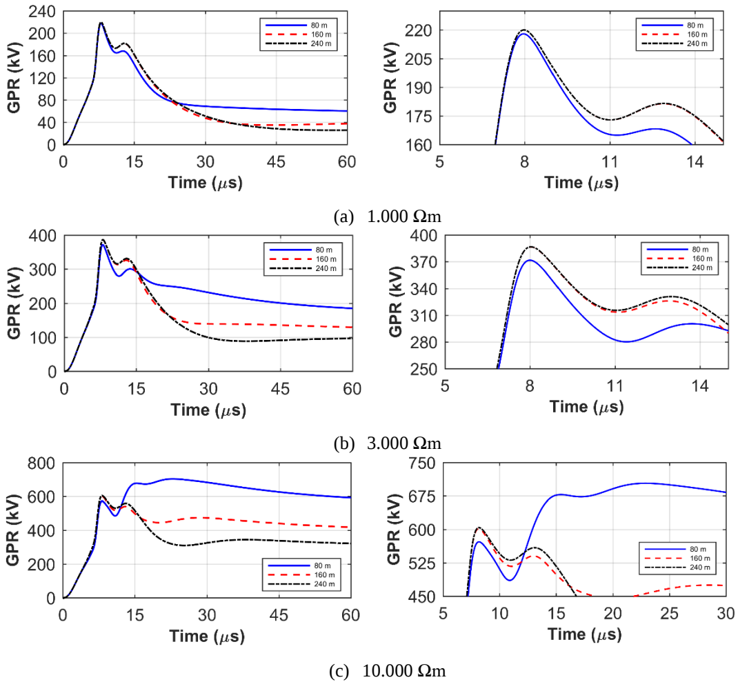
Figura 3.6 GPRs desenvolvidos em resposta a correntes representativas de primeiras descargas, a curva à direita representa a imagem a esquerda ampliada na região do pico do GPR (a) 1.000 \Omega m , (b) 3.000 \Omega m , (c) 10.000 \Omega m .
