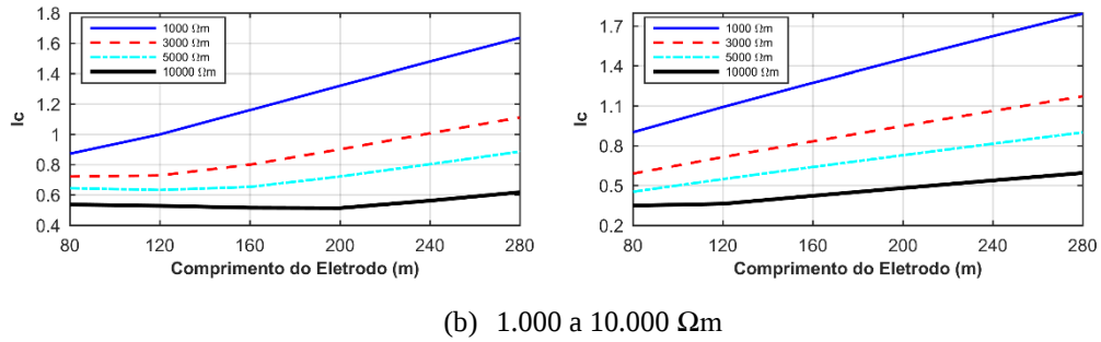
Figura 3.7 Coeficiente de impulso em função do comprimento do eletrodo de interligação, em resposta a correntes representativas de primeiras descargas (curvas à esquerda) e descargas subsequentes (curvas à direita) descendentes negativas e ascendentes negativas, para solos de resistividade (a) 50 a 600 Ωm, (b) 1.000 a 10.000 Ωm.
