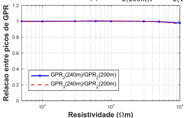
(d) GPR_2(240m)/GPR_2(200m) e GPR_3(240m)/GPR_2(200m)
