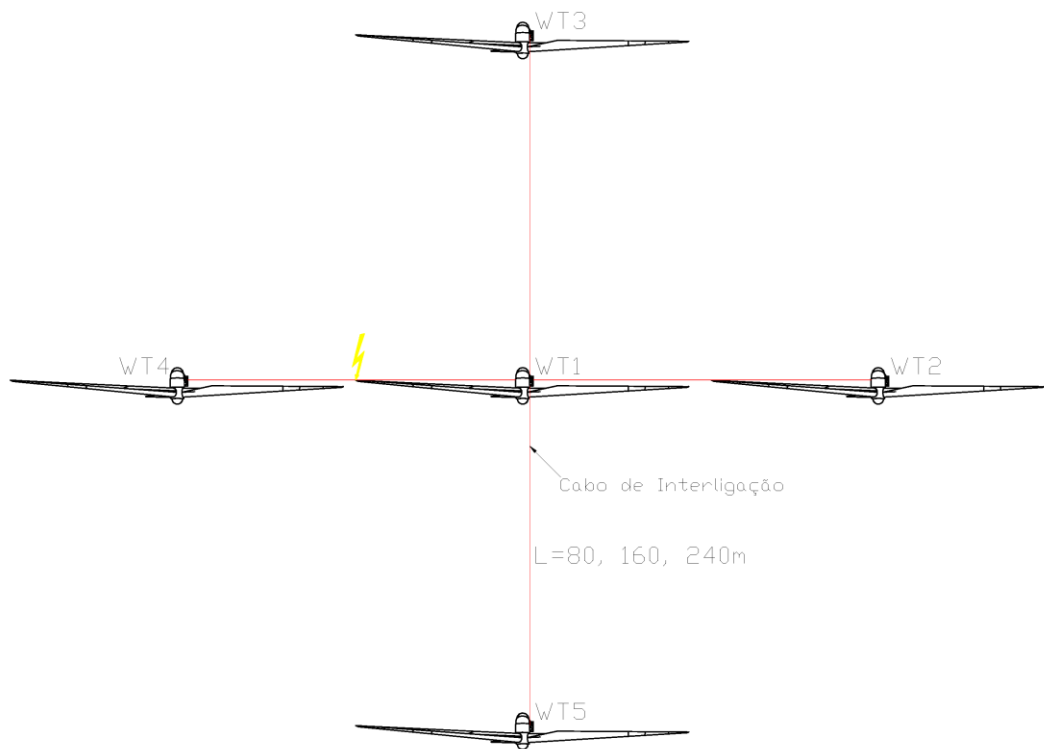
Figura 3.5 Representação do trecho do parque eólico simulado. A torre WT1, atingida pela descarga atmosférica, com sistema de aterramento interligado aos aterramentos das outras 4 torres adjacentes: WT2, WT3, WT4 e WT5.
