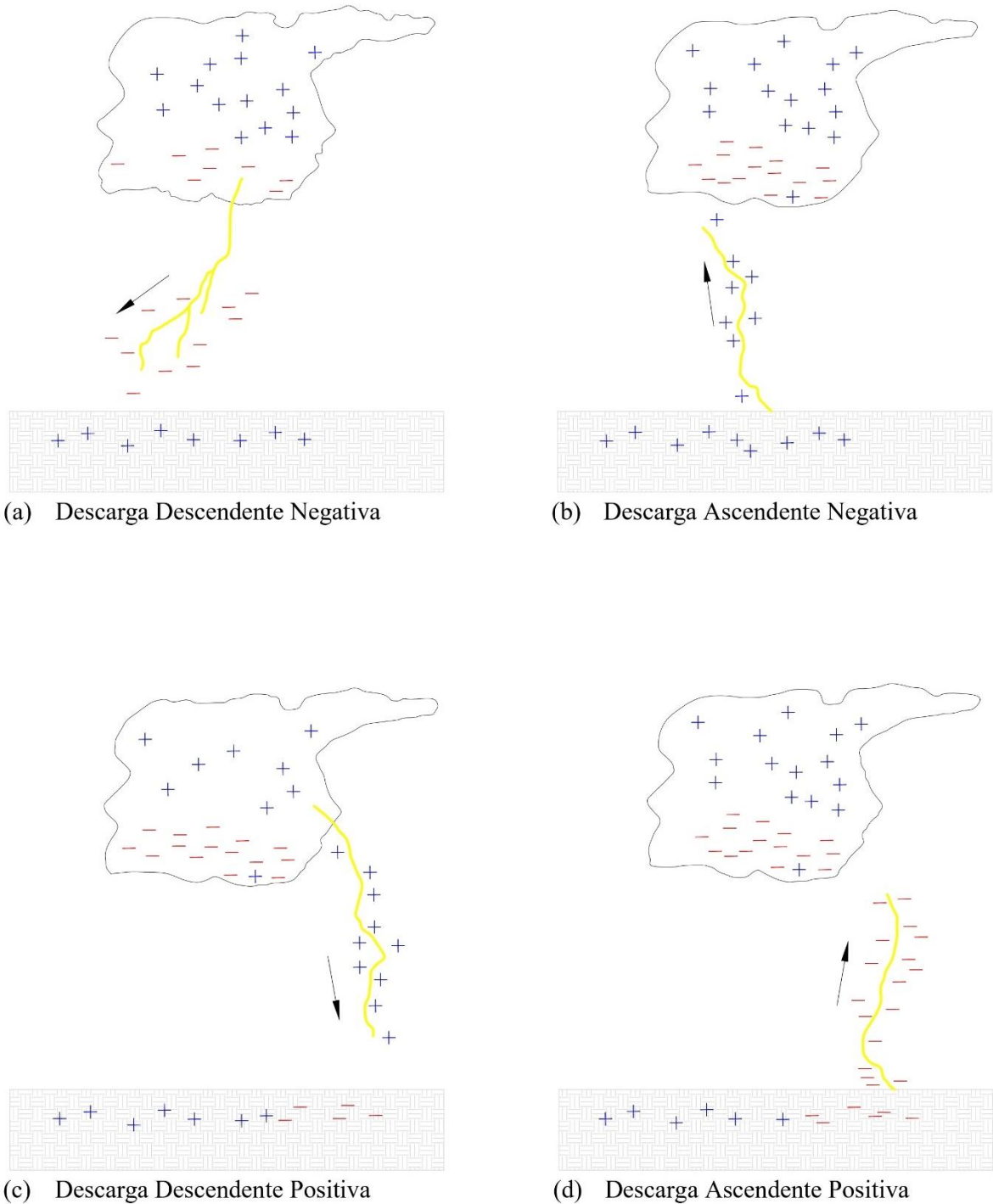
Figura 2.2 Ilustração do fenômeno de descarga atmosférica entre a base da nuvem e o solo. No caso de descargas descendentes, apenas a porção inferior do canal é representada. (a) Descarga descendente negativa, (b) Descarga ascendente negativa, (c) Descarga descendente positiva, (d) Descarga ascendente positiva.
