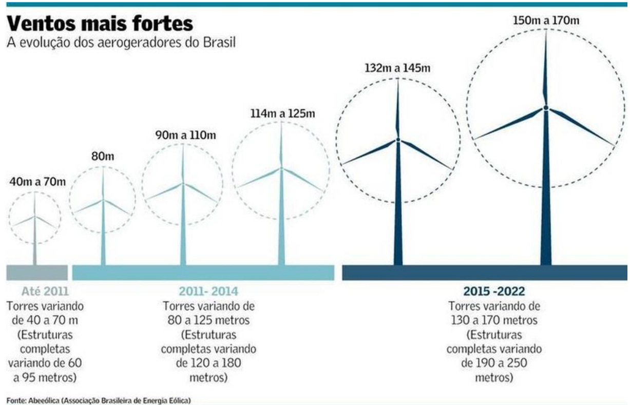
Figura 2.10 Evolução da altura das torres e da estrutura completa das turbinas eólicas ao longo dos últimos anos. Retirado de [37].
