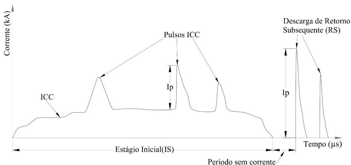
Figura 2.6 Representação estilizada da forma de onda de corrente associada com uma descarga ascendente – Adaptado de [11].
