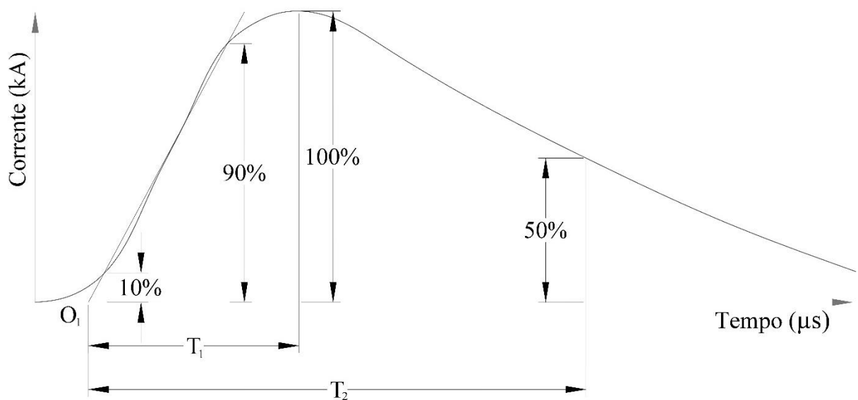
Figura 2.1 Parâmetros da corrente de descarga, considerando uma forma de onda estilizada.
