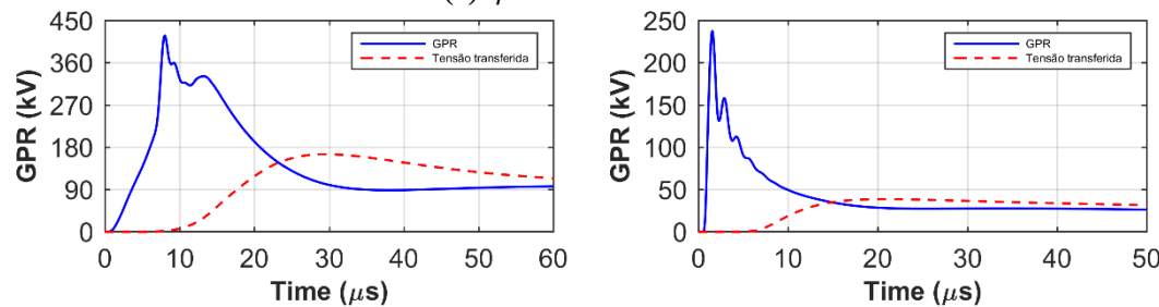
(c) \rho = 3.000 \Omega m e L = 240 m
