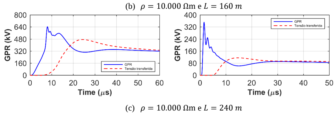
Figura 3.10 GPRs e tensão transferida, desenvolvidos em resposta a correntes representativas de primeiras descargas (curvas à esquerda) e descargas subsequentes (curvas à direita) descendentes negativas e ascendentes negativas, para solos de resistividade 10.000 \Omega m e comprimento do eletrodo de interligação (a) 80 m, (b) 160 m, (c) 240 m.
