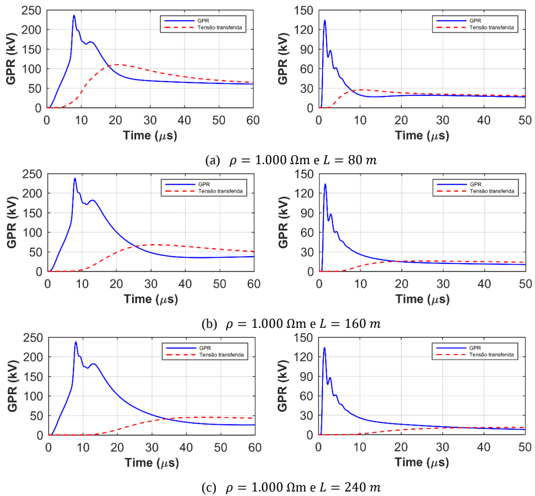
Figura 3.8 GPRs e tensão transferida, desenvolvidos em resposta a correntes representativas de primeiras descargas (curvas à esquerda) e descargas subsequentes (curvas à direita) descendentes negativas e ascendentes negativas, para solos de resistividade 1.000 \Omega m e comprimento do eletrodo de interligação (a) 80 m, (b) 160 m, (c) 240 m.
