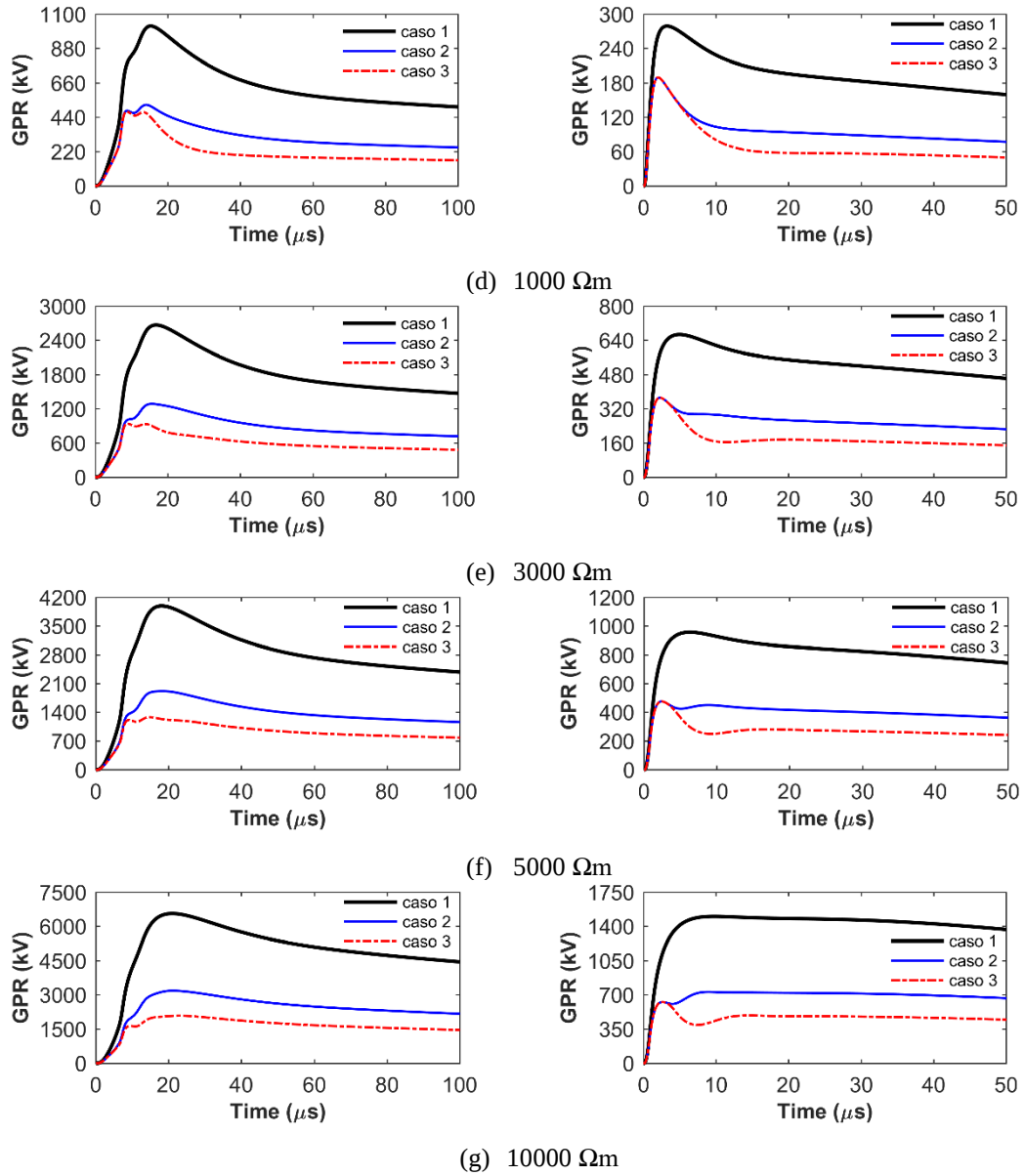
Figura 3.2 GPRs desenvolvidos em resposta a correntes representativas de primeiras descargas (curvas à esquerda) e descargas subsequentes descendentes negativas e correntes de retorno associadas às ascendentes (curvas à direita), para solos de resistividade (a) 50 \Omega\text{m} , (b) 300 \Omega\text{m} , (c) 1.000 \Omega\text{m} , (d) 3.000 \Omega\text{m} , (e) 10.000 \Omega\text{m} . Caso 1, aterramento da turbina eólica isolado; Caso 2, aterramento da turbina eólica conectado ao eletrodo de interligação de L=80 m (desconsiderando o aterramento da segunda turbina eólica); Caso 3, sistema completo (aterramentos de ambas as turbinas conectados via eletrodo de interligação de L=80 m).
