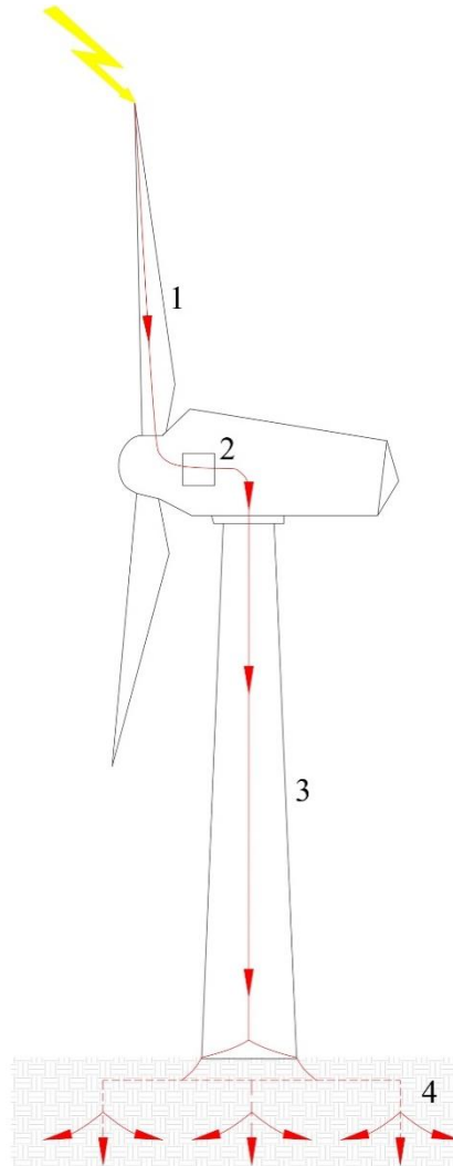
Figura 2.8 Caminho da corrente de descarga (1-condutor de descida na pá, 2-contato dinâmico, 3- corpo da torre, 4-sistema de aterramento).
