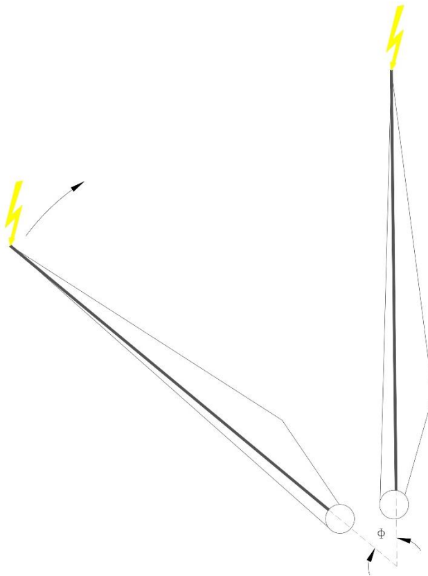
Figura 2.9 Condutor de descida nas pás de uma turbina eólica.
