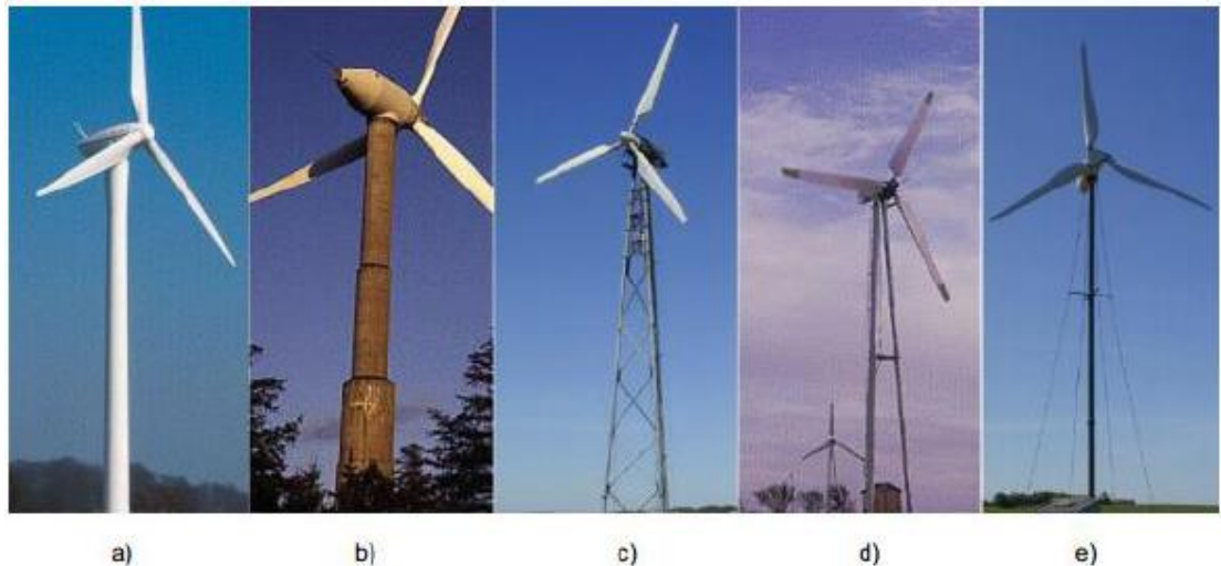
Figura 2.11 Diferentes tipos de torres: a) torre tubular em aço; b) torre em betão; c) torre treliçada; d) torre em tripé; e) torre estaiada. Retirado de [36].
