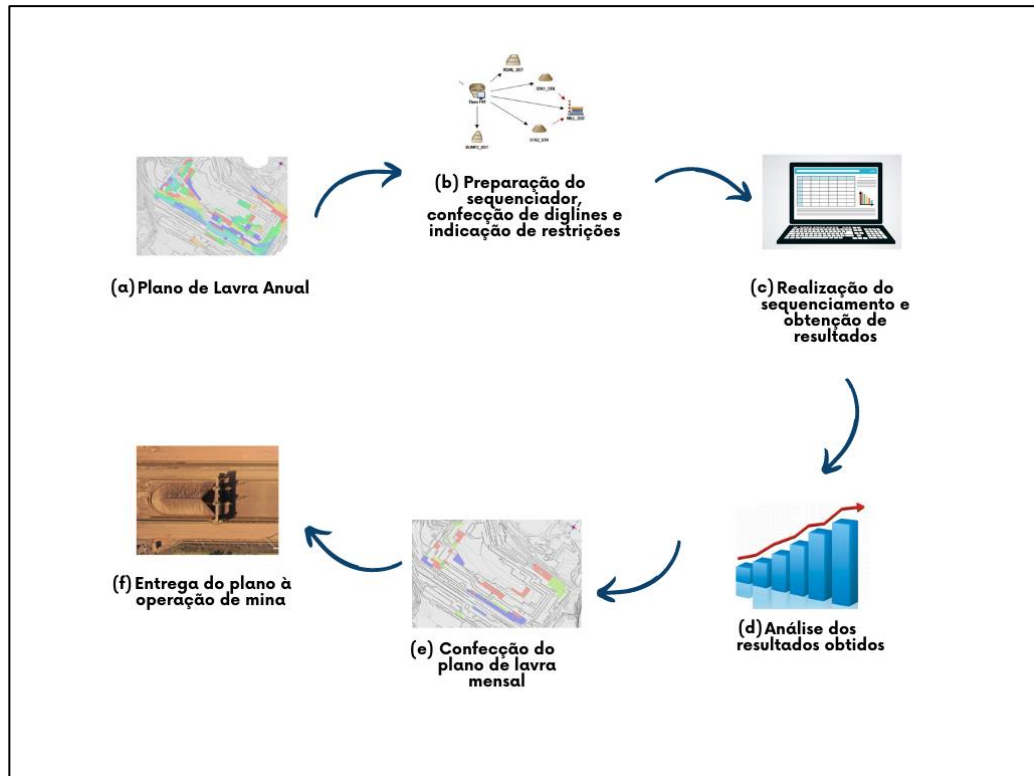
Figura 3.16 - Fluxograma esquemático da metodologia proposta para confecção de plano de lavra mensal subdividido em pilhas, utilizando sequenciador matemático
