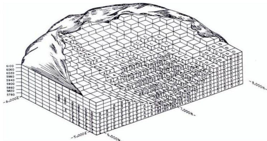
Figura 2.1- Modelo de blocos conceitual
