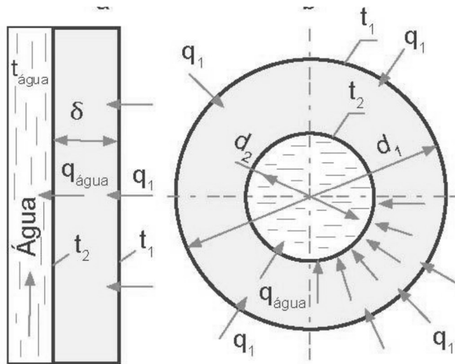
Figura 13 - Representação esquemática de um tubo de painel refrigerado
