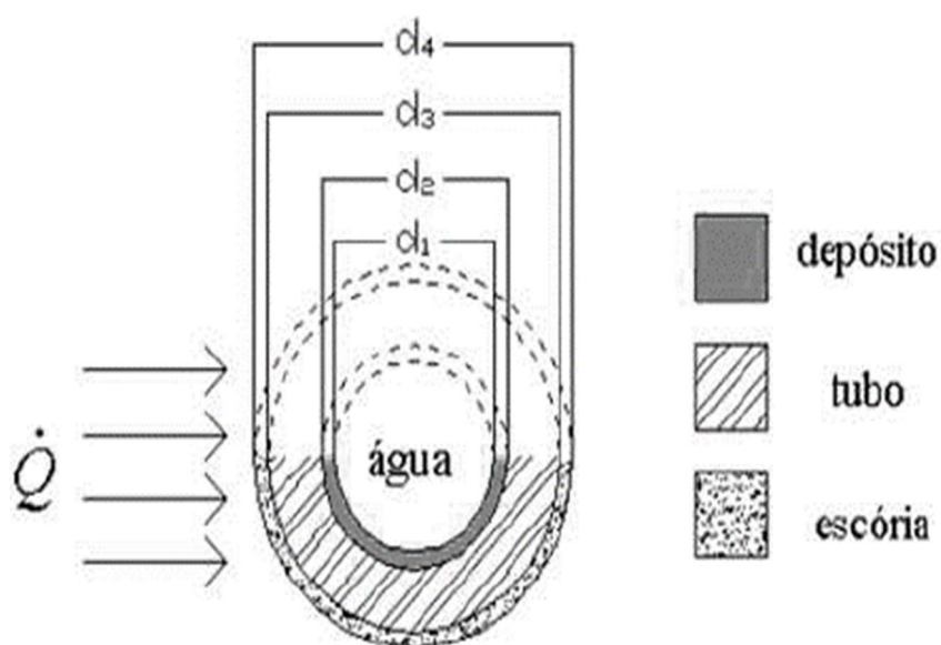
Figura 11 - Vista interna do tubo de refrigeração do painel refrigerado Fonte: Silva (2014)
