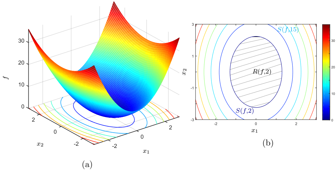
Figura 2.1: Gráfico e curvas de nível para o funcional de duas variáveis, f((x_1, x_2)) = 3x_1^2 + x_2^2 . Em (a), tem-se o gráfico em três dimensões de f , enquanto as curvas de nível de f são apresentadas no plano x_1 \times x_2 . Em (b), tem-se o plano x_1 \times x_2 , destacando-se as curvas de nível, em especial, S(f, 15) (—). Também em destaque, tem-se a região de subnível R(f, 2) ( \cdots ), limitada por S(f, 2) (—).
