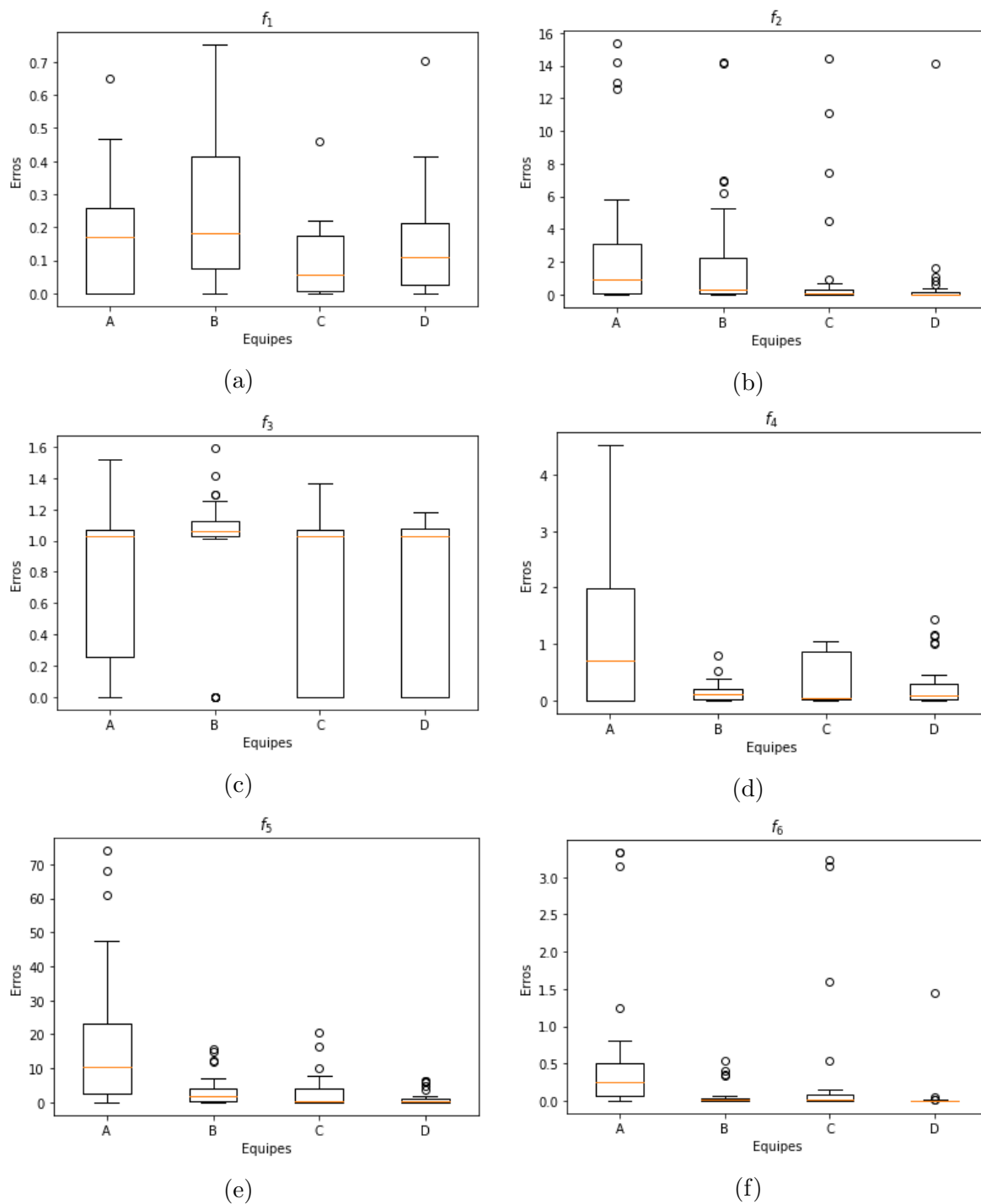
Figura 5.8: Boxplots das 30 execuções de cada um dos problemas f_1 ao f_6 considerando os erros dados nas matrizes \mathbf{E}_A , \mathbf{E}_B , \mathbf{E}_C e \mathbf{E}_D .
