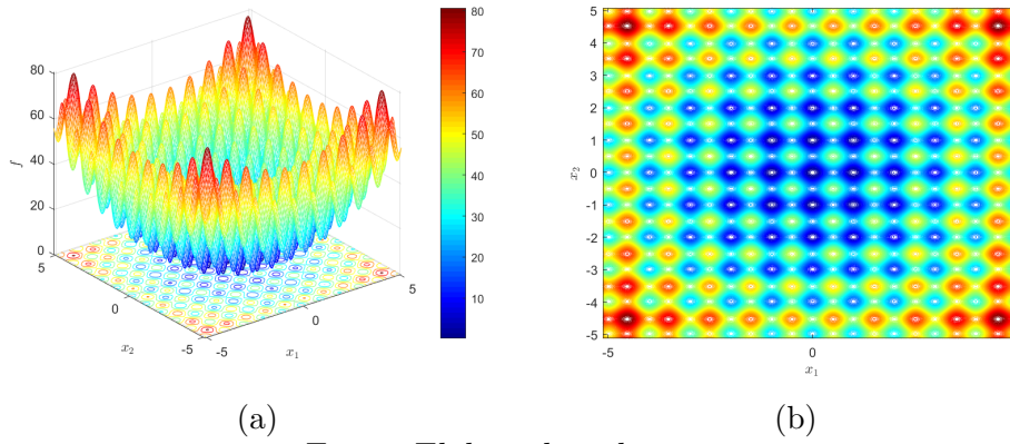
Figura 5.4: Função Rastrigin Bidimensional (5.5). Em (a), tem-se a representação de f(x_1, x_2) e em (b), tem-se o mapa de calor.
