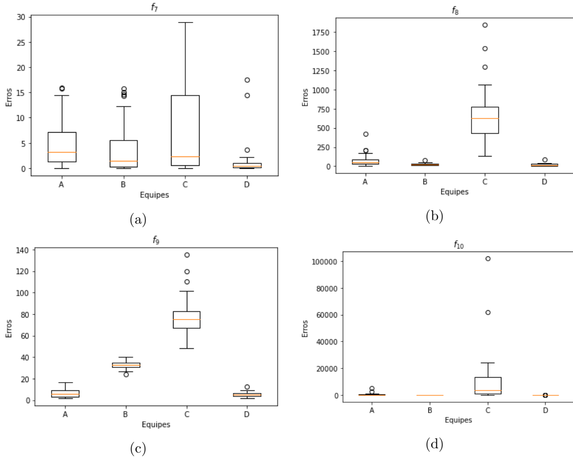
Figura 5.9: Boxplots das 30 execuções de cada um dos problemas f_7 ao f_{10} considerando os erros dados nas matrizes \mathbf{E}_A , \mathbf{E}_B , \mathbf{E}_C e \mathbf{E}_D .
