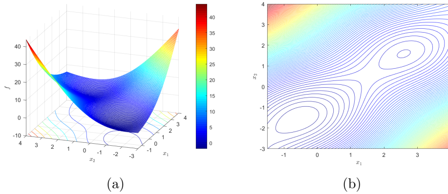
Figura 5.6: Função McCormick Bidimensional (5.7). Em (a), tem-se a representação de f(x_1, x_2) e em (b), tem-se as curvas de nível.
