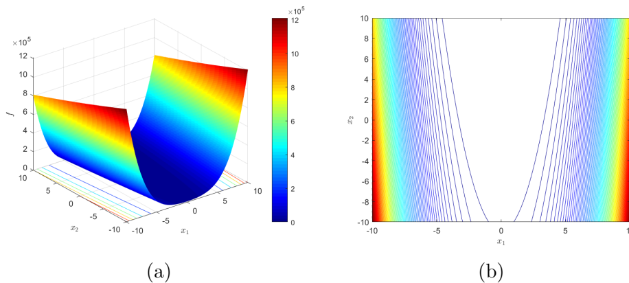
Figura 5.5: Função Rosenbrock Bidimensional (5.6). Em (a), tem-se a representação de f(x_1, x_2) e em (b), tem-se as curvas de nível.
