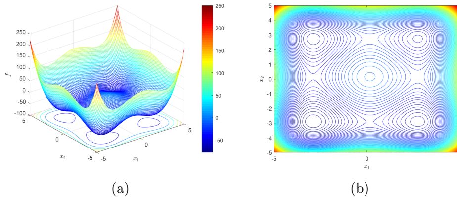
Figura 5.7: Função Styblinski–Tang Bidimensional (5.8). Em (a), tem-se a representação de f(x_1, x_2) e em (b), tem-se as curvas de nível.
