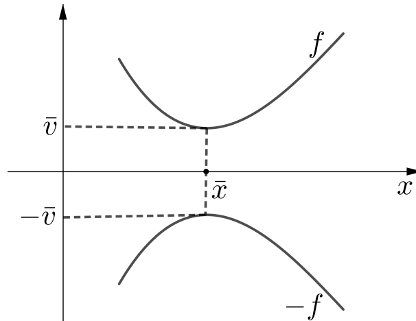
Figura 2.4: Na Figura, temos que o ponto \bar{x} que maximiza -f(x) é o mesmo que minimiza f(x) .
