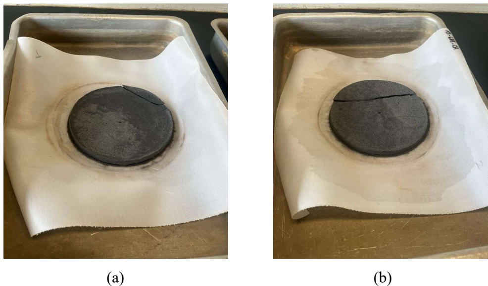
Figura 42: (a) Torta do teste 01, (b) torta do teste 02
