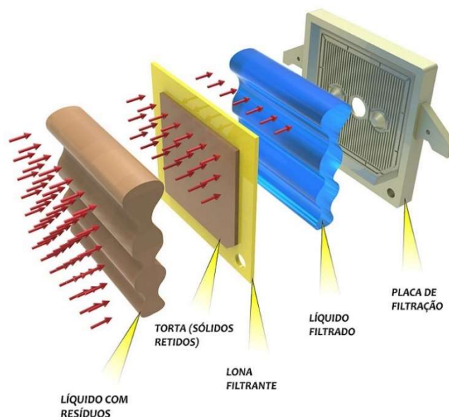
Figura 4 – Esquema de alimentação de polpa em placas de um filtro prensa.
