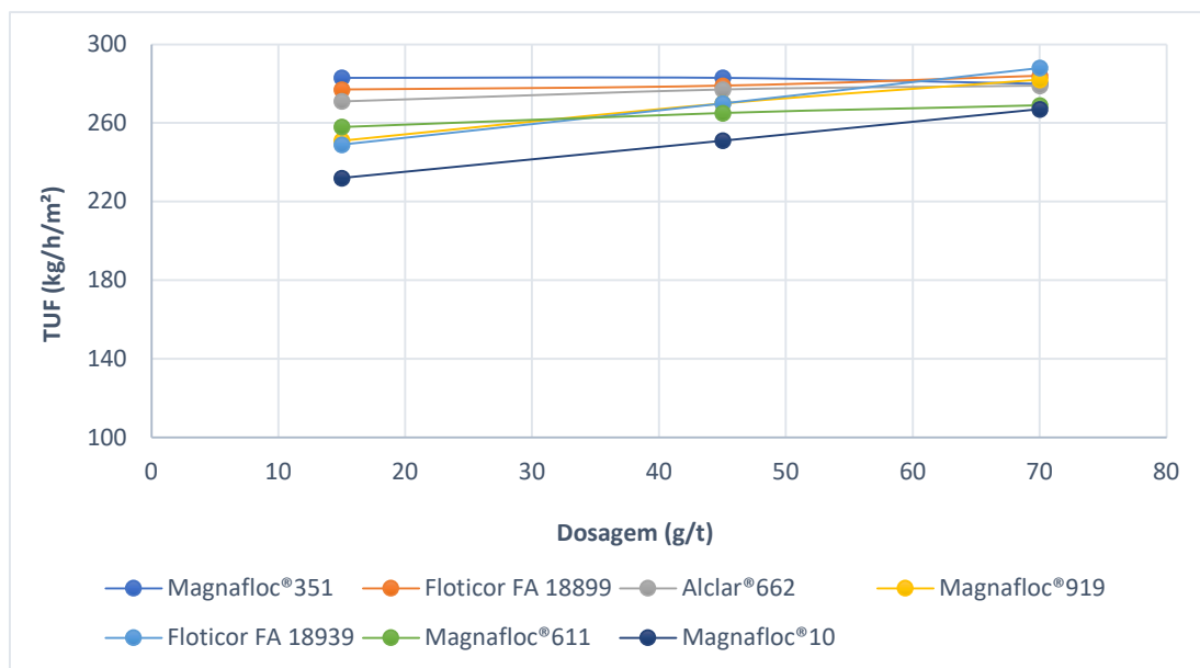
Figura 35 – Resultados de TUF em função da dosagem de reagente
