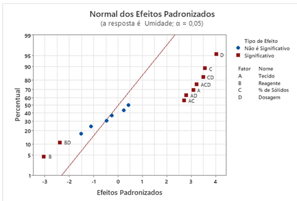
Figura 37 – Efeitos das interações para umidade
