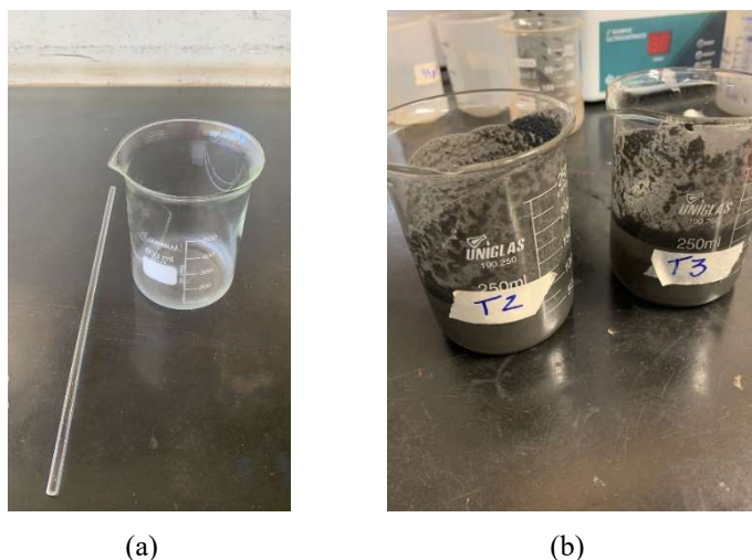
Figura 22 – (a) béquer e bastão de vidro, (b) béquer com polpa condicionada
