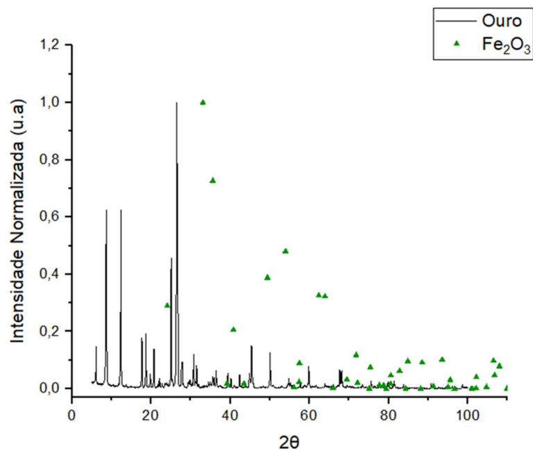
Figura 29 – Difratoograma de raios-X para \text{Fe}_2\text{O}_3
