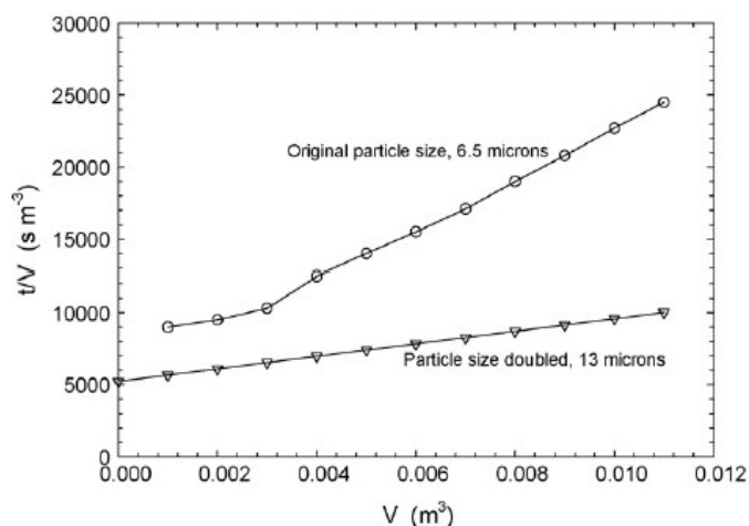
Figura 8 – O efeito na plotagem de t/V vs. V em relação aos tamanhos das partículas
