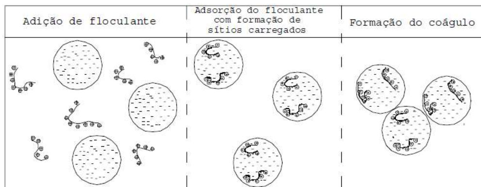
Figura 13 – Etapas envolvidas na formação do coágulo.
