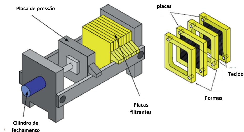
Figura 3 – Disposição geral de um filtro prensa indicando os elementos essenciais.
