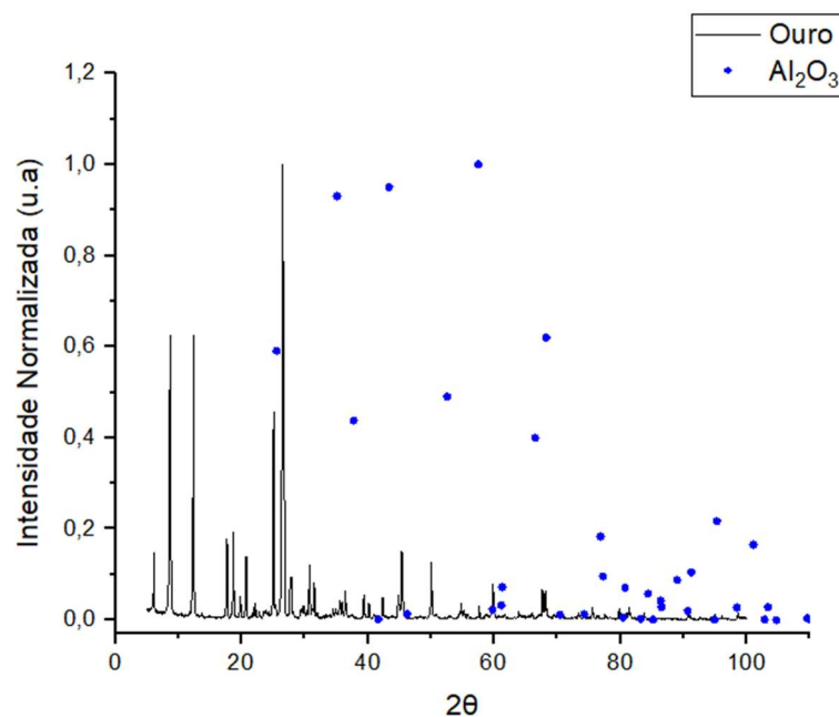
Figura 30 – Difratoograma de raios-X para \text{Al}_2\text{O}_3
