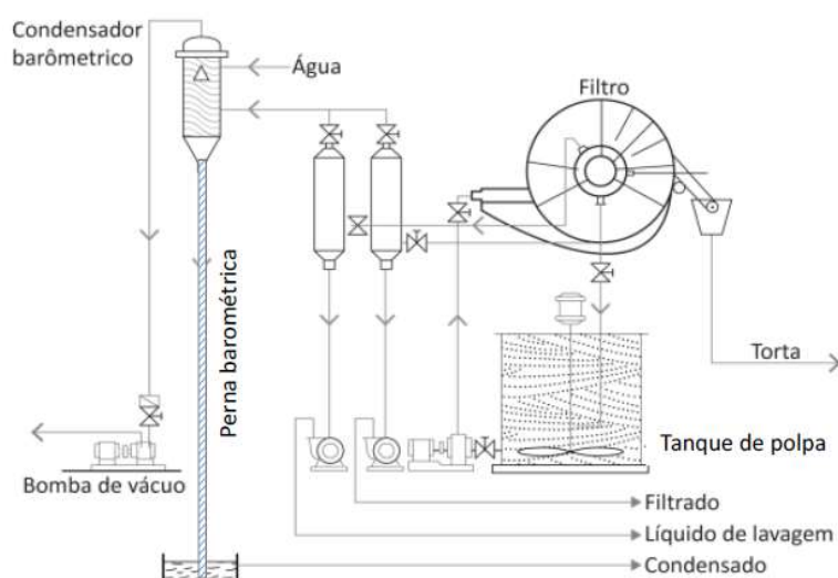
Figura 6 – Exemplo de um fluxograma de instalação industrial com filtro rotativo a vácuo
