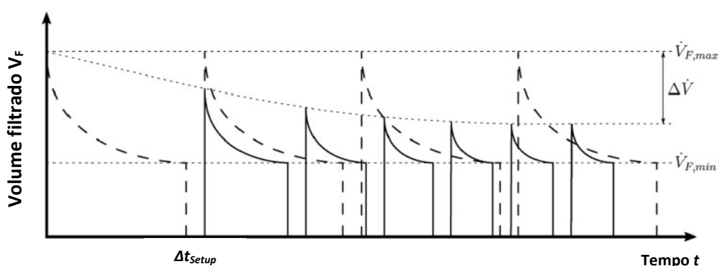
Figura 10 – Efeito da regeneração/limpeza inadequada no fluxo do filtrado
