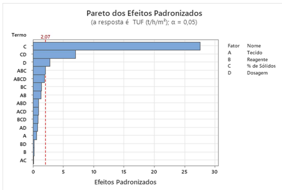
Figura 39 – Efeitos padronizados das interações em forma de Pareto
