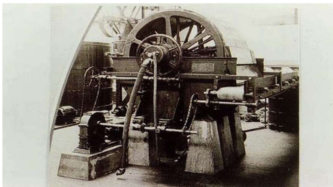
Figura 2 – Um dos primeiros filtros de tambor a vácuo rotativo de 1910 (FLSmidth GmbH).
