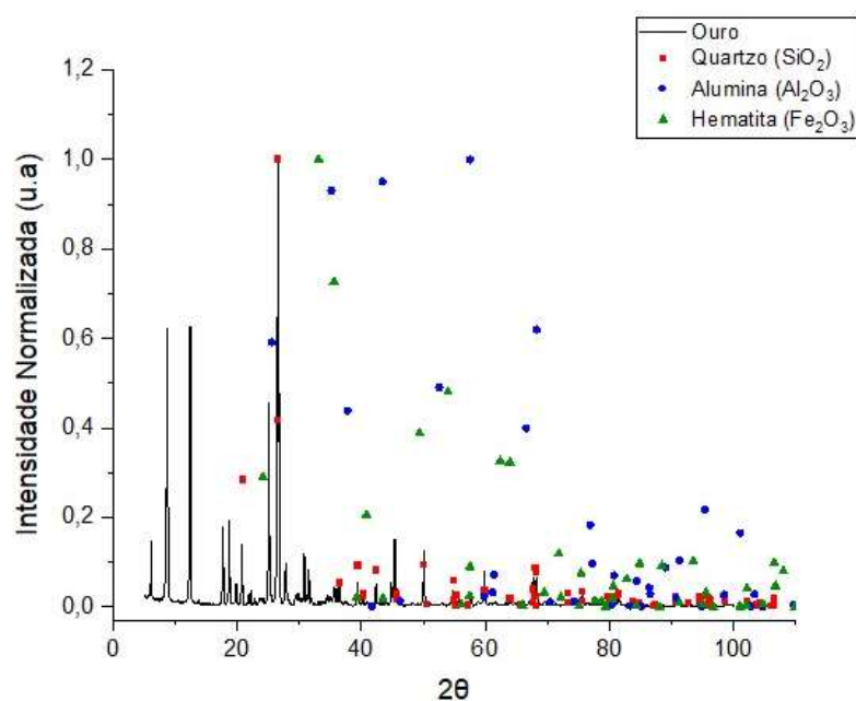
Figura 27 – Difratoograma de raios-X dos minerais agrupados
