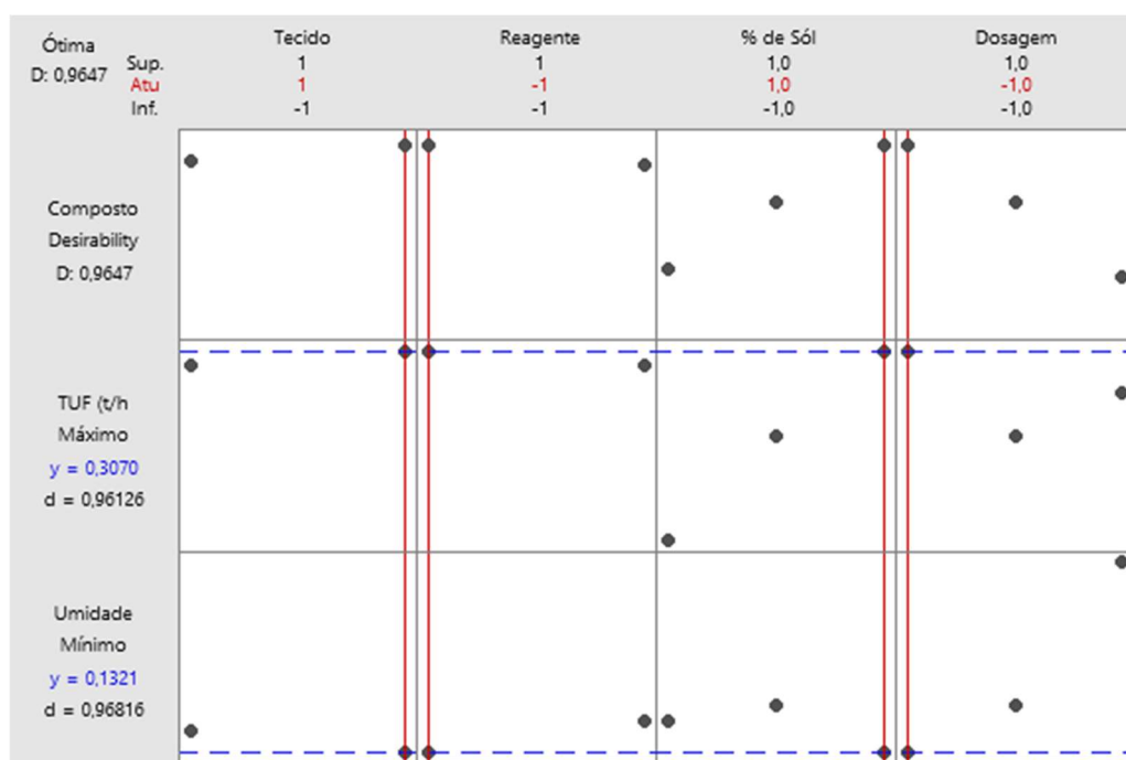
Figura 41 – Otimização da resposta: TUF (t/h/m 2 ) e Umidade
