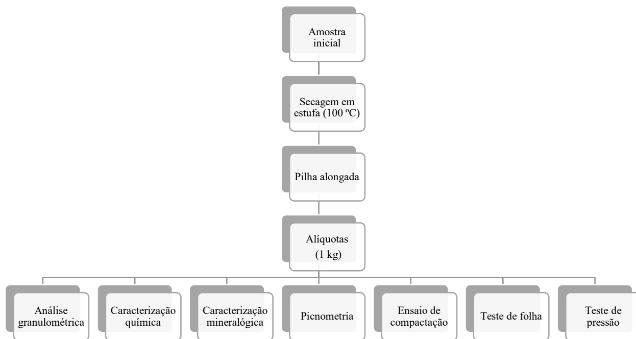
Figura 17 – Etapas de preparação de amostras
