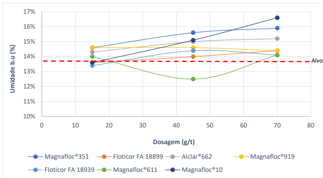
Figura 34 – Resultados de umidade média com utilização dos reagentes
