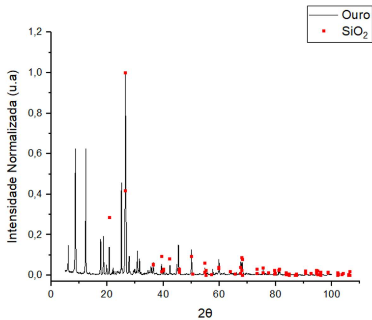
Figura 28 – Difratoograma de raios-X para \text{SiO}_2
