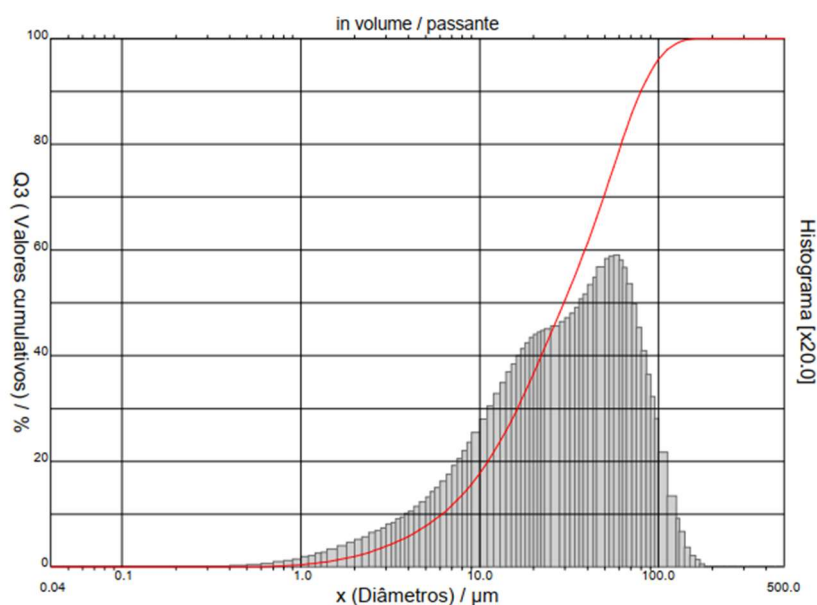
Figura 32 – Curva granulométrica via granulômetro (CILAS 1090)
