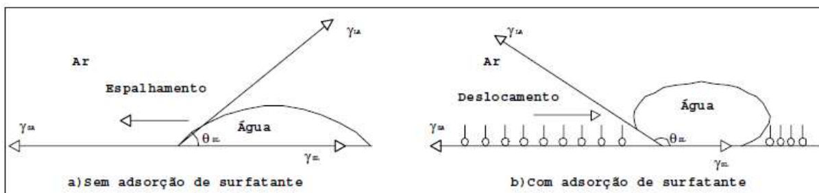
Figura 14 – Influência do surfatante no grau de hidrofobicidade na superfície da partícula.
