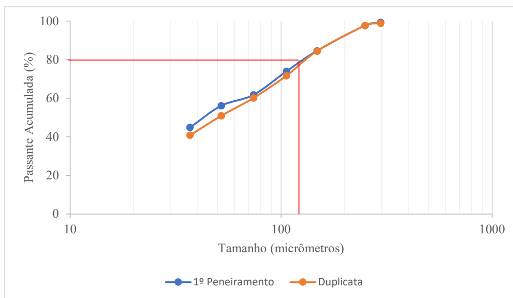
Figura 31 – Teste de granulometria
