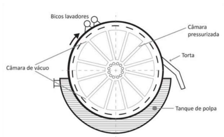
Figura 5 – Diagrama simplificado de um filtro rotativo à vácuo
