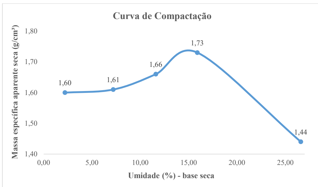
Figura 33 – Gráfico da curva de compactação
