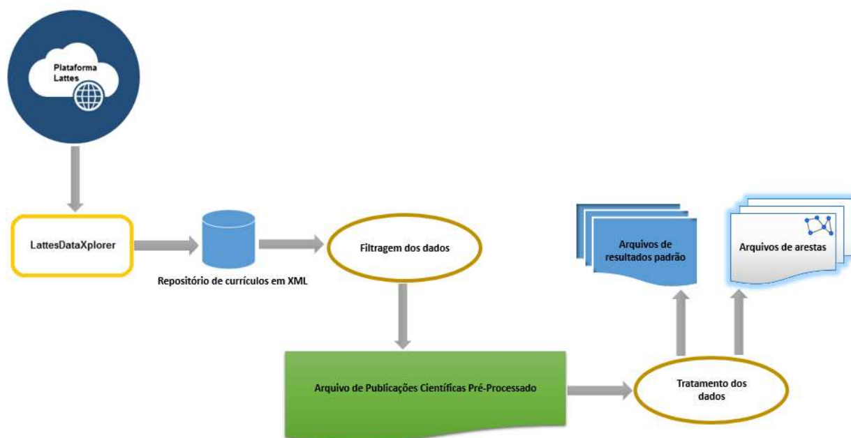
Figura 4.2 - Visão geral do arcabouço de componentes que suporta as análises de palavras-chave dos artigos.
