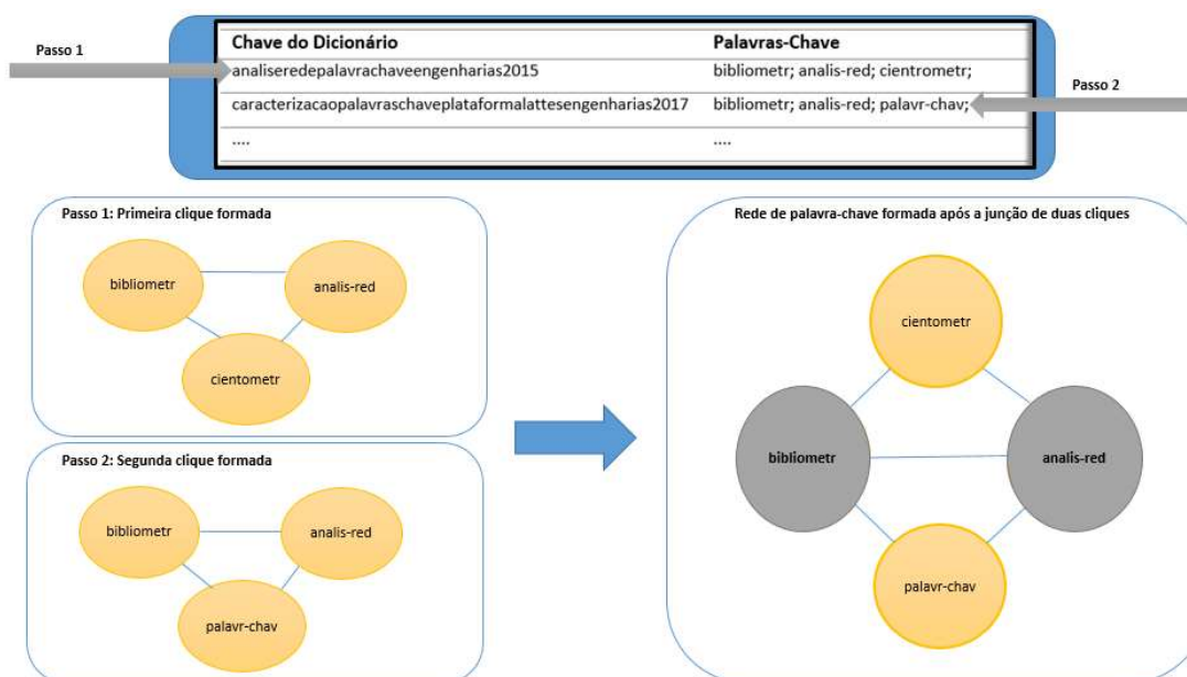
Figura 4.5 - Exemplo do processo de construção de redes de palavras-chave considerando dois artigos.
