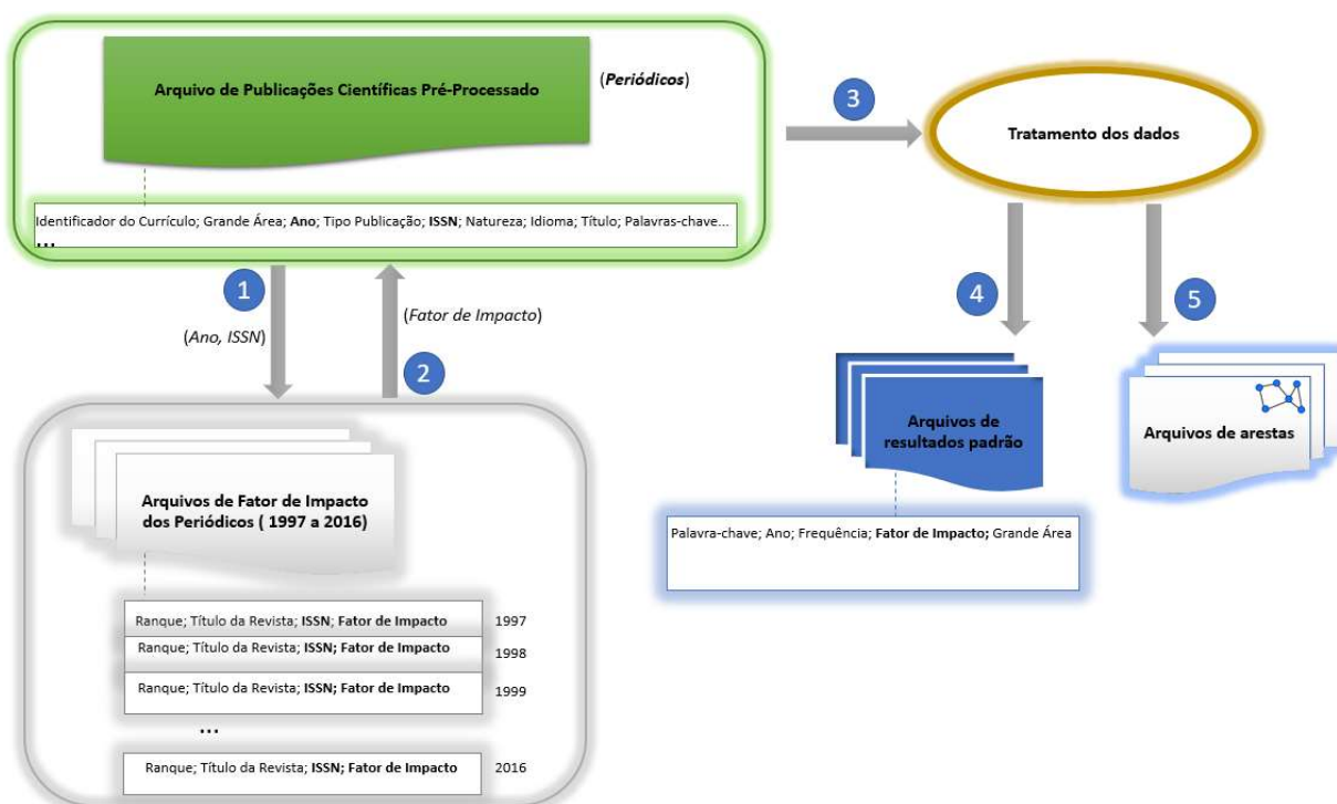
Figura 6.2 - Processo para adição de FI dos periódicos ao conjunto dos dados científicos dos doutores.
