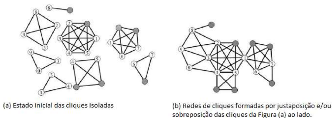
Figura 2.6 - Exemplo do estado inicial de cliques isoladas e uma configuração para redes de cliques. (FADIGAS e PEREIRA, 2013)
