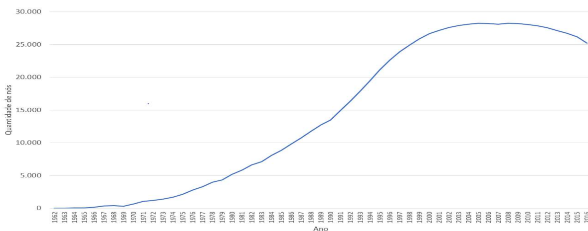
Figura 5.10 - Evolução temporal da quantidade de vértices.
