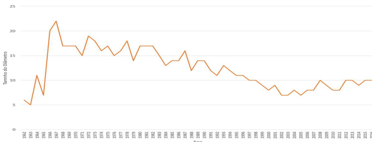
Figura 5.11 - Evolução do diâmetro da rede.
