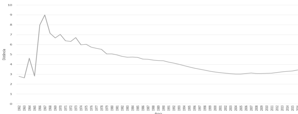
Figura 5.12 - Evolução do caminho mínimo médio.
