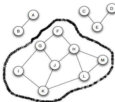
Figura 2.4 - Exemplo de um grafo G com três componentes. A componente em destaque representa a componente gigante. (Fonte: adaptado de EASLEY e KLEINBERG, 2010)
