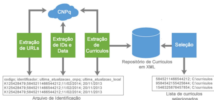
Figura 4.1 - Processo de extração de dados LattesDataXplorer (Fonte: Dias, 2016).
