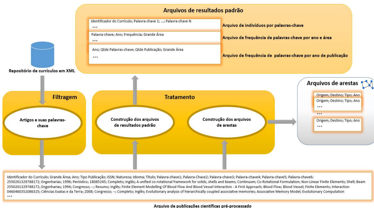
Figura 4.3 - Processo de filtragem e tratamento dos dados.
