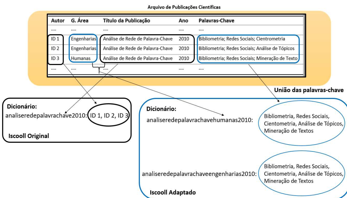
Figura 4.4 - Exemplo de processamento dos métodos ISCoolI original e adaptado.
