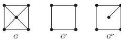
Figura 2.3 - Exemplo de um grafo G e seus subgrafos G' e G'' (Fonte: DIESTEL, 2010)
