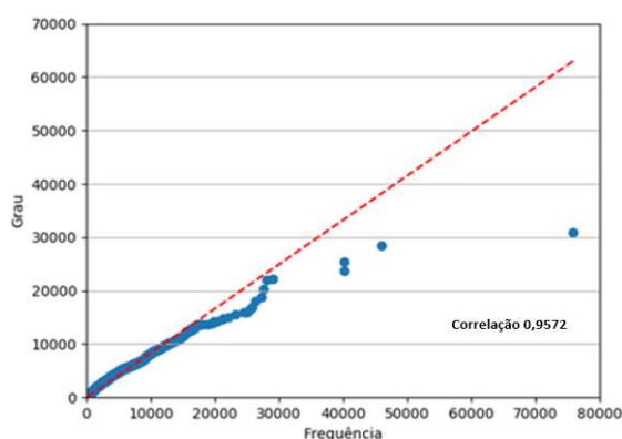
Figura 5.13 - Correlação entre as medidas de importância frequência e grau.
