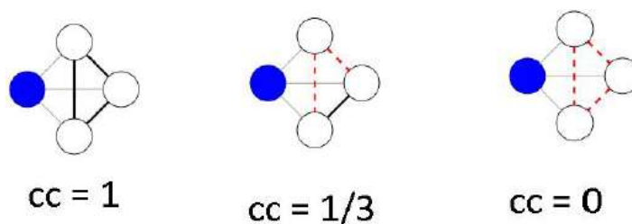
Figura 2.5 - Exemplo do cálculo do coeficiente de clusterização de um nodo em três cenários diferentes (BENEVENUTO, 2010)
