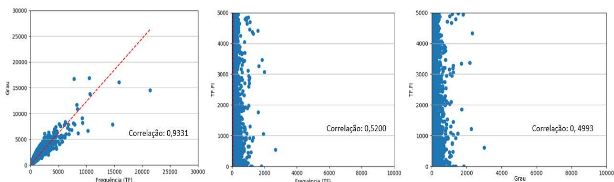
Figura 6.6 - Correlação entre as medidas de importância frequência e grau; e frequência e TF.FI.
