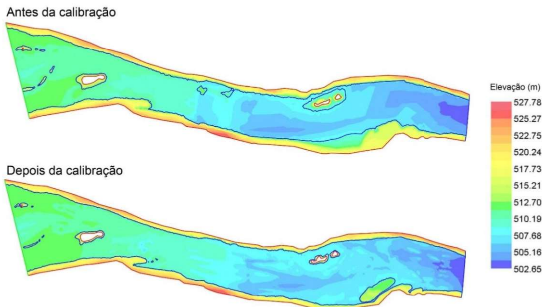
Figura 6 - Batimetria do trecho do rio antes e após calibração. O contorno em azul escuro representa o nível d'água. Após a calibração a superfície d'água se tornou mais parecida com as imagens de satélite observadas.
