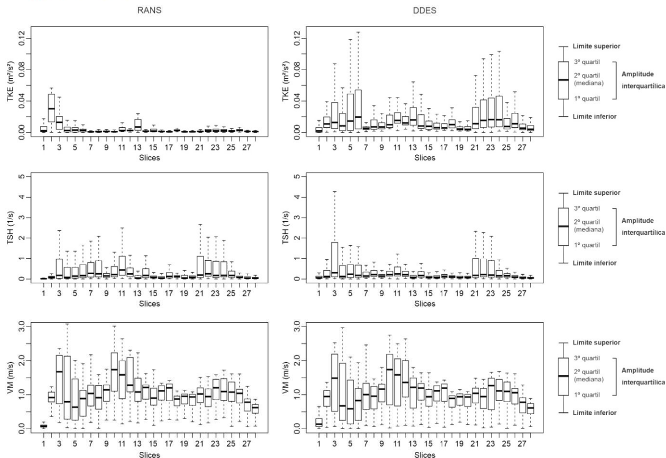
Figura 42 - Boxplots da energia cinética turbulenta, da deformação hidráulica e da magnitude da velocidade de acordo com as seções transversais no modelo RANS e no modelo DDES
