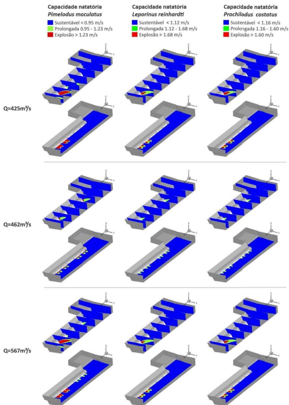
Figura 32 - Corredores de natação para as espécies P. maculatus , P. costatus e L. reinhardti no canal de fuga em diferentes vazões
