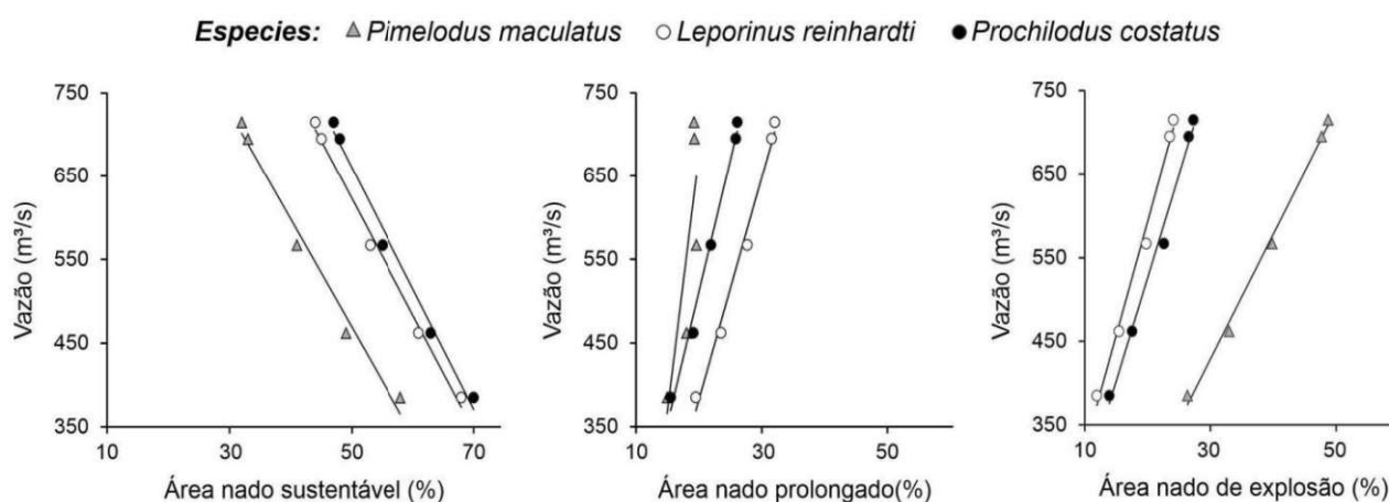
Figura 34 - Relação entre vazão e área do modo de natação para P. maculatus , P. costatus , e L. reinhardti no trecho do rio
