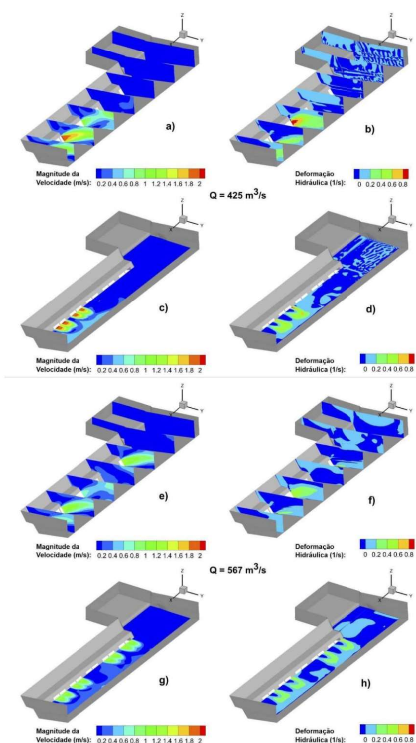
Figura 27 – Perfil de magnitude da velocidade para a vazão 425 m 3 /s (a, c) e para a vazão 567 m 3 /s (e, g); perfil de deformação hidráulica para a vazão 425 m 3 /s (b, d) e para a vazão de 567 m 3 /s (f, h) no modelo 3D
