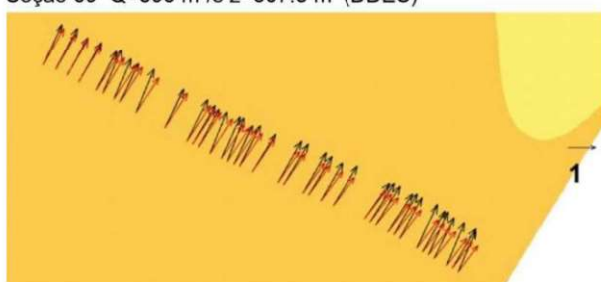
Seção 69 Q=596 \text{ m}^3/\text{s} z=507.3 \text{ m} (DDES)
