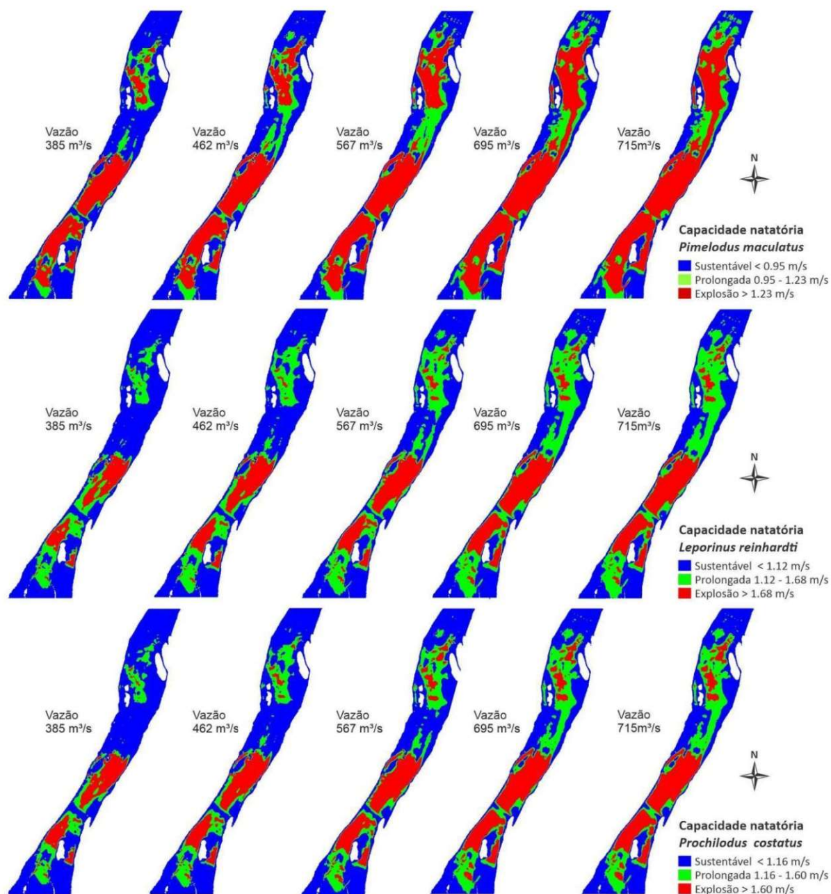
Figura 33 - Corredores de natação para as espécies P. maculatus , P. costatus e L. reinhardti no trecho do rio em diferentes vazões
