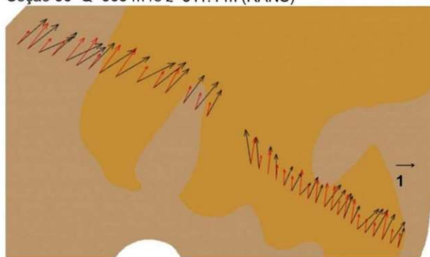
Seção 69 Q=596 \text{ m}^3/\text{s} z=507.3 \text{ m} (RANS)
