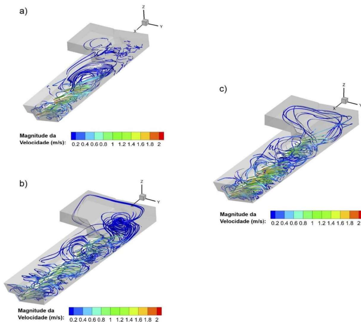
Figura 26 - Linhas de corrente com indicação da magnitude de velocidade para vazões de 425 m 3 /s (a), 462 m 3 /s (b) e 567 m 3 /s (c) no modelo 3D do canal de fuga
