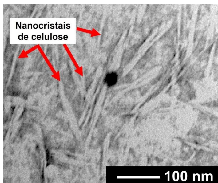
Figura 26 - Micrografia dos nanocristais de celulose após o processo de hidrólise ácida, diálise e centrifugação. Usando MET para uma concentração de 0,001%
