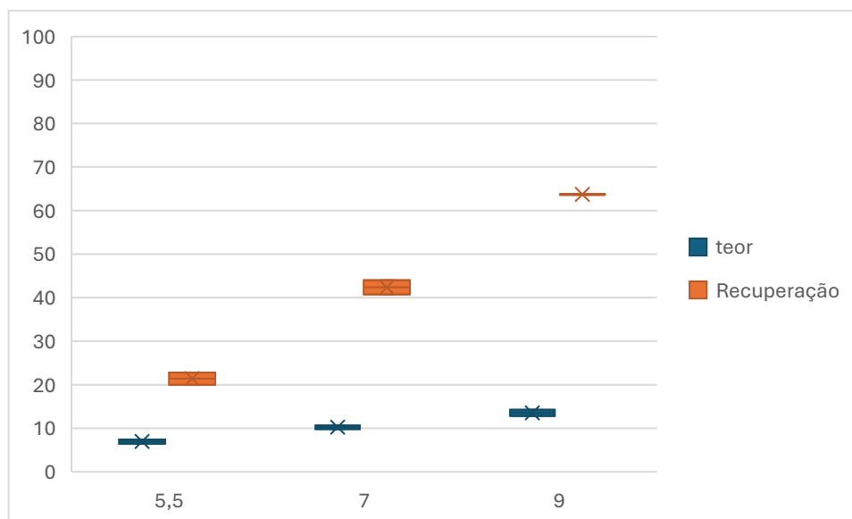
Figura 36 - Flotação direta em função do pH, dosagem de coletor 250g/t e depressor nanoamido 475g/t
