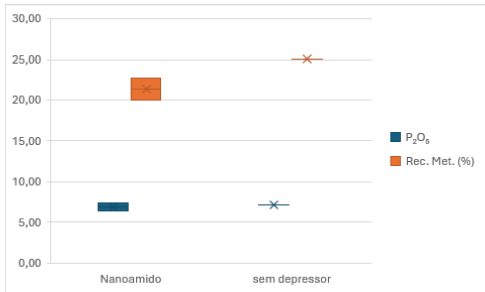
Figura 38 - Resultados de flotação direta com pH 5,5, dosagem de coletor 250g/t e depressor 475g/t
