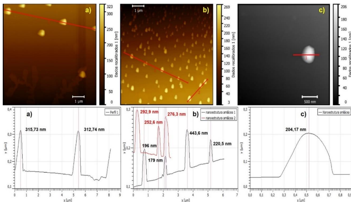
Figura 30 - Micrografias de MFA no modo topografia com área de medição de 14\ \mu\text{m}^2 , de PRAB. a) imagem topográfica em escala de 1\ \mu\text{m} com mensuração de diâmetros de duas nanoestruturas amiláceas, b) imagem topográfica em escala de 1\ \mu\text{m} com mensuração de diâmetros de três nanoestruturas amiláceas na cor vermelha e mais três, na cor preta e c) imagem topográfica em escala de 500\text{nm} com mensuração de diâmetro de apenas 1 nanoestrutura amilácea. Os gráficos abaixo representam as medidas em escala nanométrica dos diâmetros das nanoestruturas das mesmas letras mostradas nos gráficos
