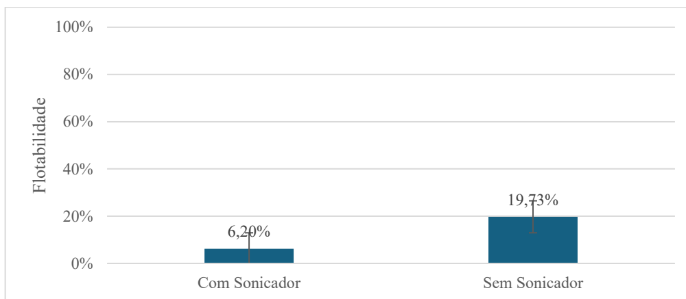
Figura 31 – Comparativo da flotabilidade de apatita na presença de nanocelulose de Eucalipto (0,5% m/m)
