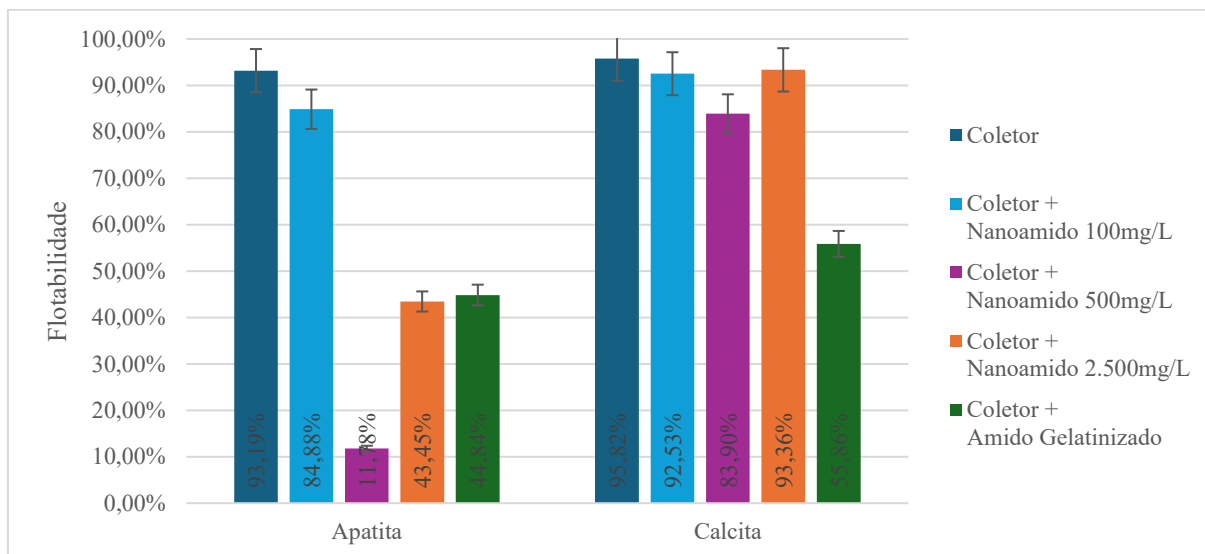
Figura 34 – Resultados da microflotação dos minerais na presença e ausência de polímeros.
