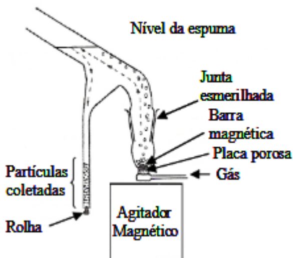
Figura 3 - Tubo de Hallimond
