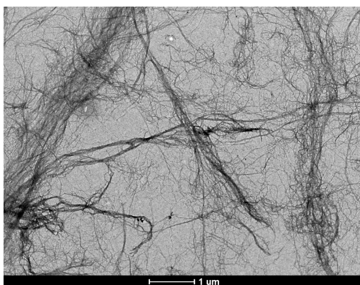
Figura 15 - Micrografias das nanofibrilas celulósicas de Pinus sp. após processo mecânico de desconfiguração da parede celular
