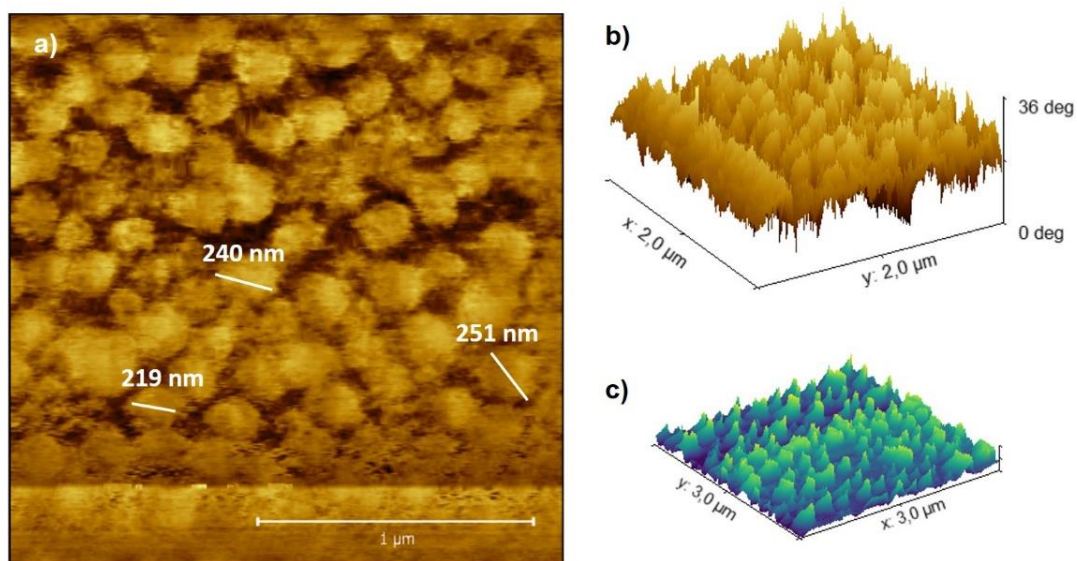
Figura 29 - Micrografias de MFA no modo a) topografia com área de medição de 64\mu\text{m}^2 , b) 4\mu\text{m}^2 e c) 9\mu\text{m}^2 , de suspensões de nanoestruturas amiláceas de PRAB
