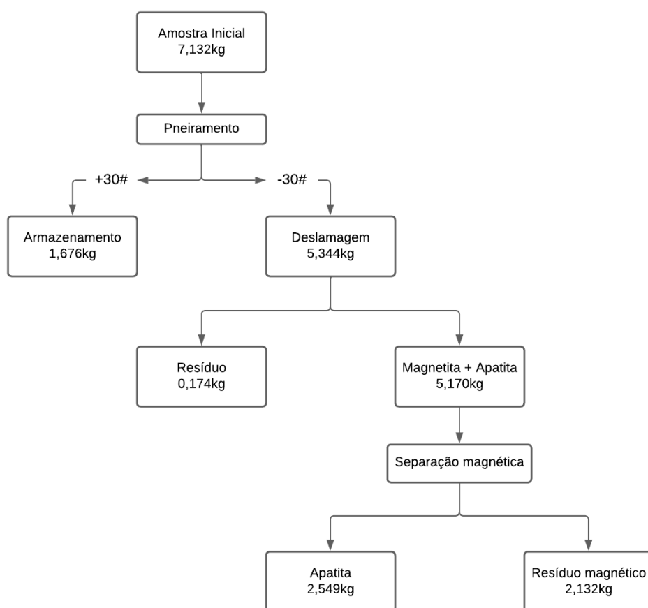
Figura 10 - Esquema da preparação das amostras de apatita
