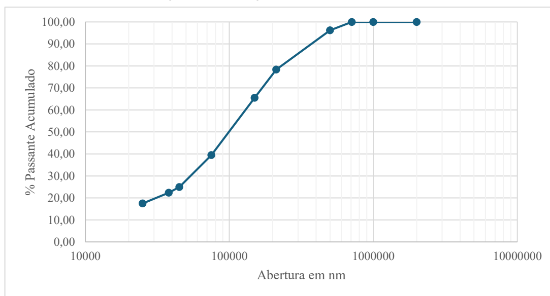
Figura 25 - Análise granulométrica da alimentação
