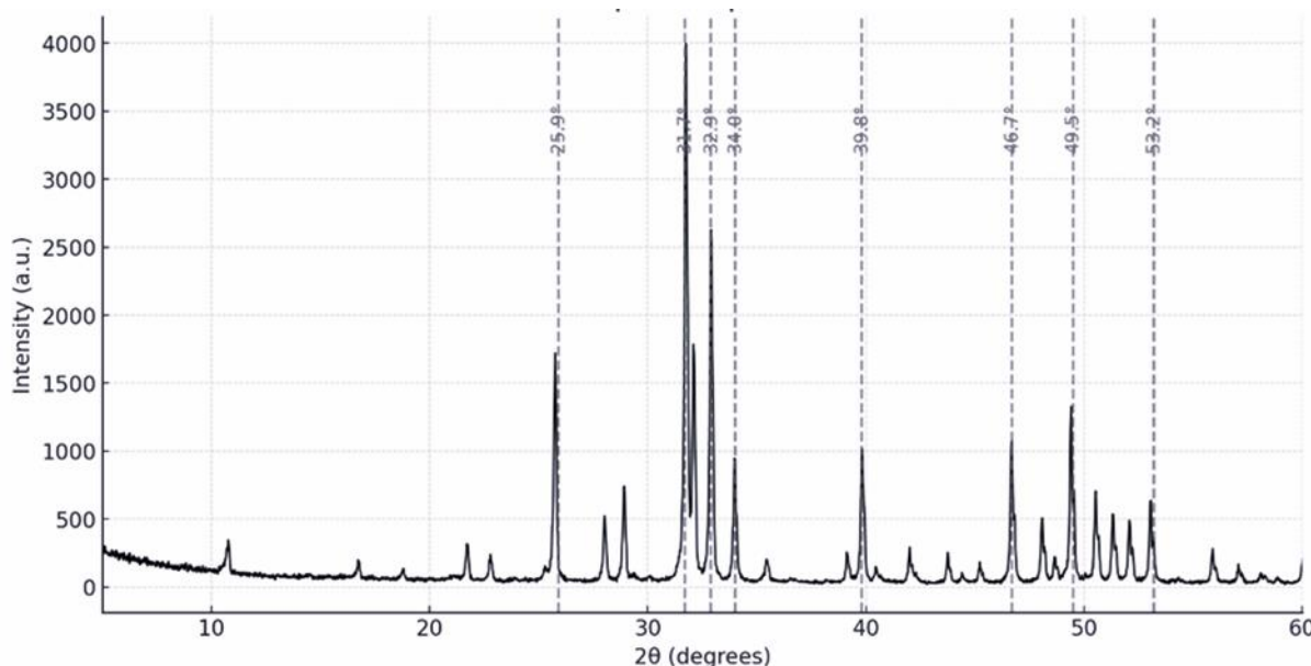
Figura 23 - DRX da apatita
