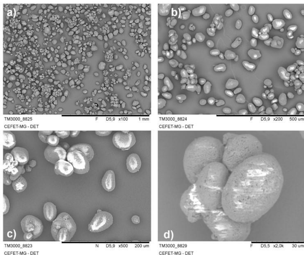
Figura 28 - Microscopia eletrônica de varredura dos grânulos de polpa residual de amido de batata. Micrografias com vários valores de barras de escala. a) 1mm; b) 500µm; c) 200µm e d) 50µm
