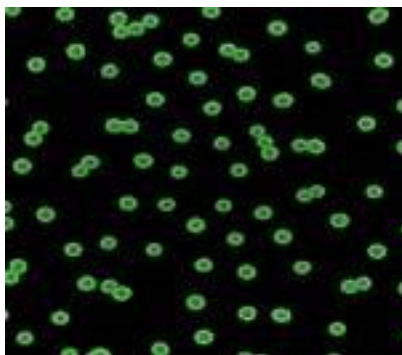
Figura 7 - Nanoshells
