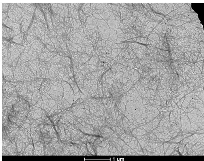
Figura 14 - Micrografias das nanofibrilas celulósicas de Eucalyptus sp. após processo mecânico de desconfiguração da parede celular
