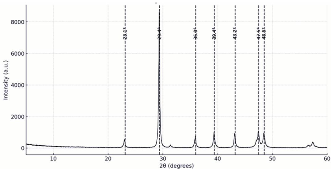
Figura 24 - DRX da calcita
