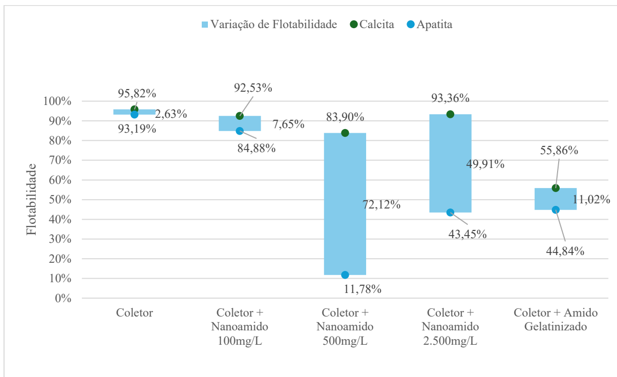
Figura 35 – Diferença entre a flotabilidade da apatita e calcita (janela de flotabilidade)
