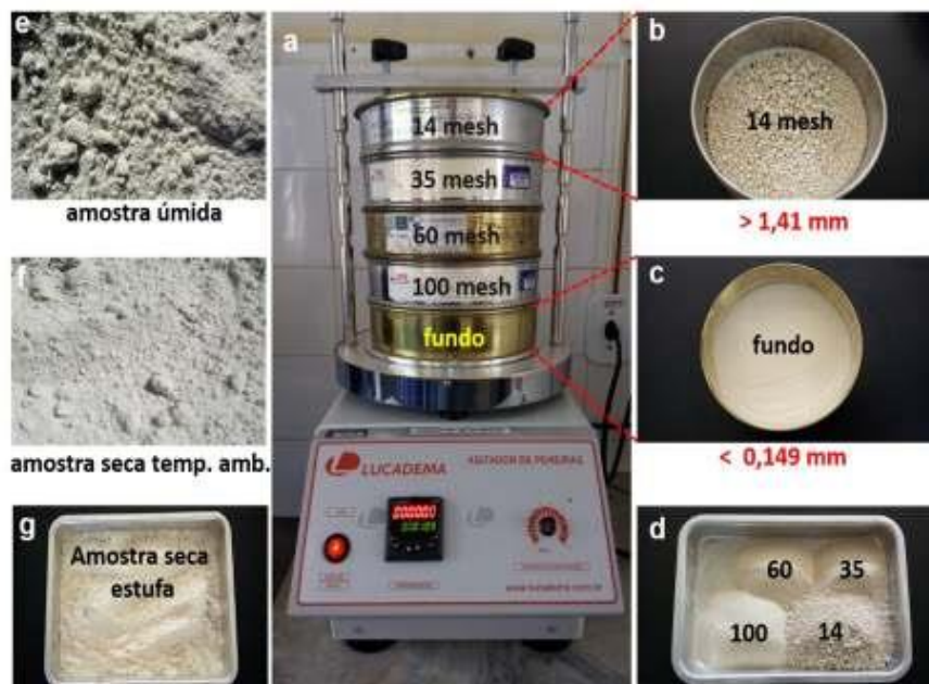
Figura 17 - Etapas de preparação das amostras de PRAB a) aparelho vibratório com quatro peneiras; b) peneira de classificação granulométrica com abertura de 1,41mm; c) peneira de classificação granulométrica com abertura de 0,59mm; d) amostra de PRAB após passagem
