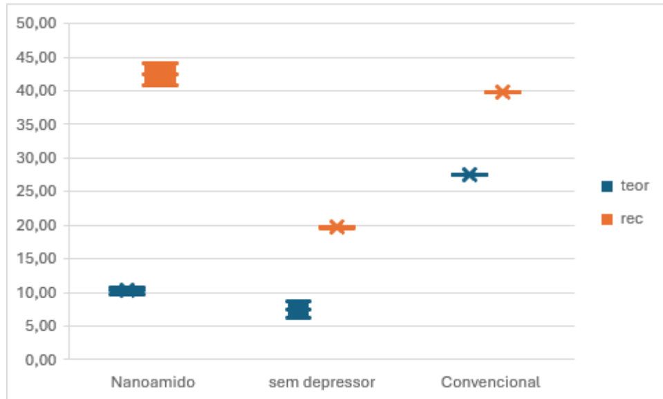
Figura 37 - Resultados de flotação com pH 9, dosagem de coletor 250g/t e depressor 475g/t
