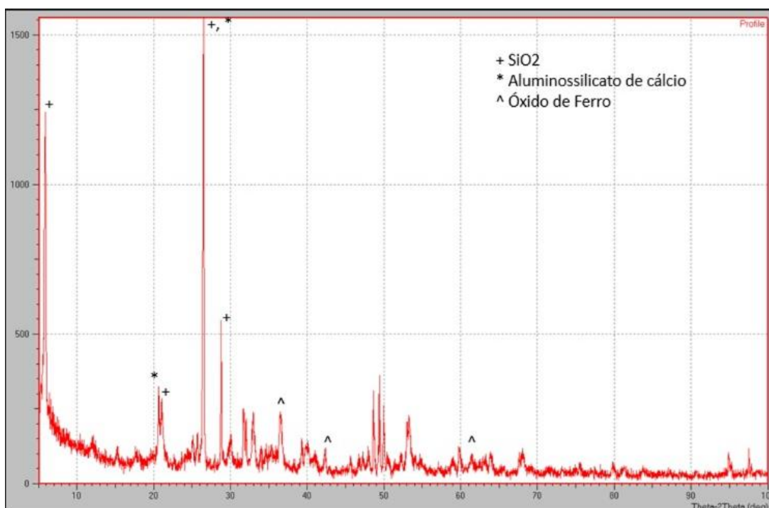
Figura 22: Espectro obtido por DRX para o precursor rejeito do minério concentração do minério fosfático em Araxá.
