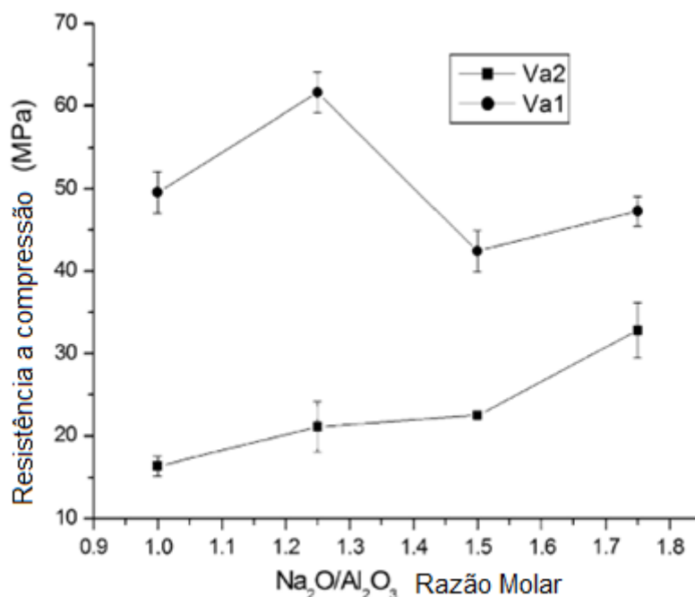
Figura 9: Resultados de resistências à compressão das cinzas ativadas por álcalis.
