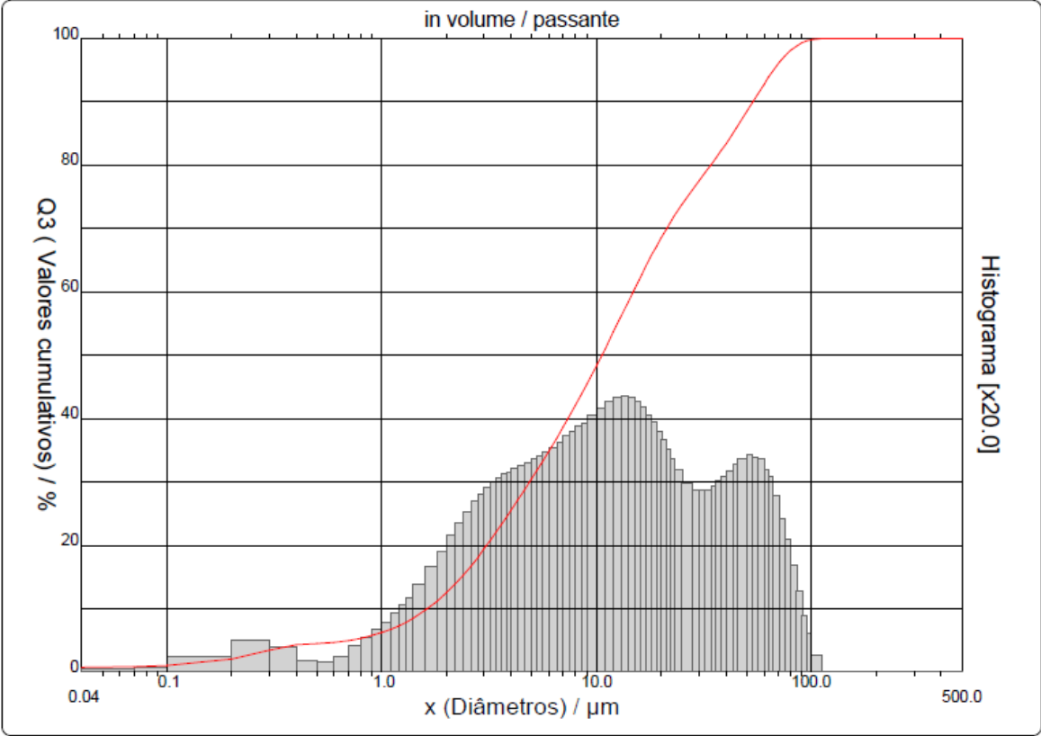
Figura 21: Distribuição granulométrica do rejeito do minério fosfático produzido em Araxá (MG).
