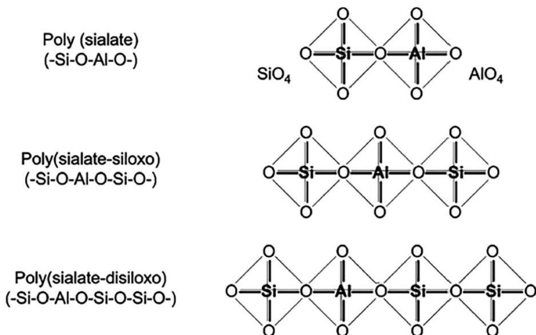
Figura 7: modelo de unidade estrutural de geopolímeros com diferentes proporções de Si/Al, Davidovits et. al., J. Therm. Anal, 2008, 2.
