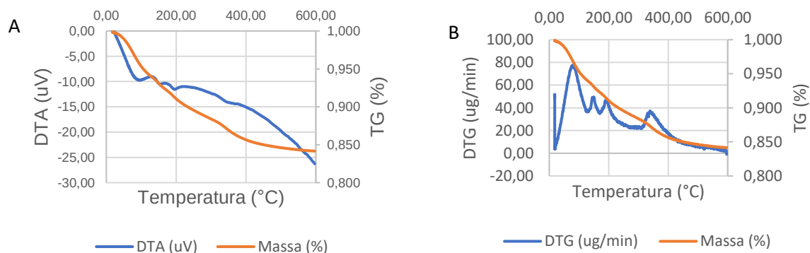
Figura 32: Curvas – A: DTA e TG e B: DTG e TG.
