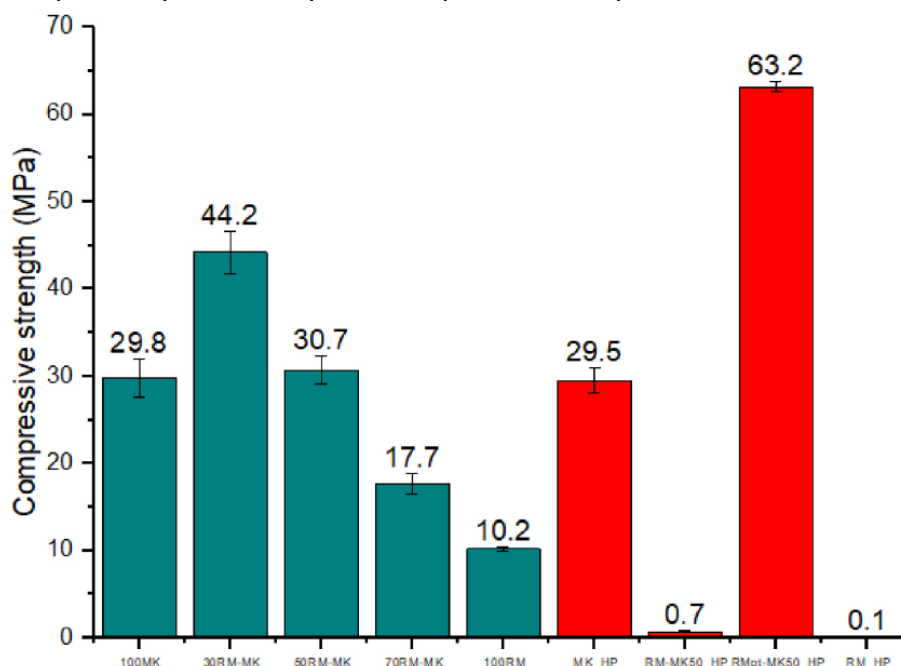
Figura 29: Valores de resistência à compressão em MPa para amostras de geopolímero cúbico alcalino (em azul) e ativado por ácido (em vermelho).
