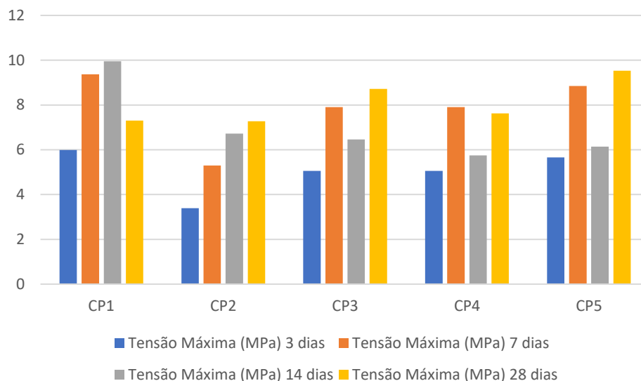
Figura 27: Tensão máxima em diferentes períodos de cura.
