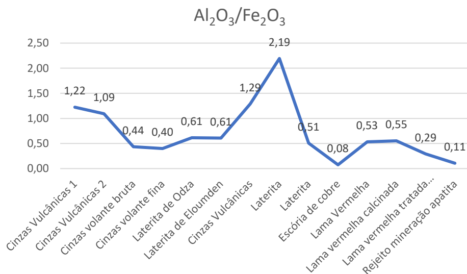
Figura 18: Relação entre a razão \text{Al}_2\text{O}_3/\text{Fe}_2\text{O}_3 e ativadores usados.
