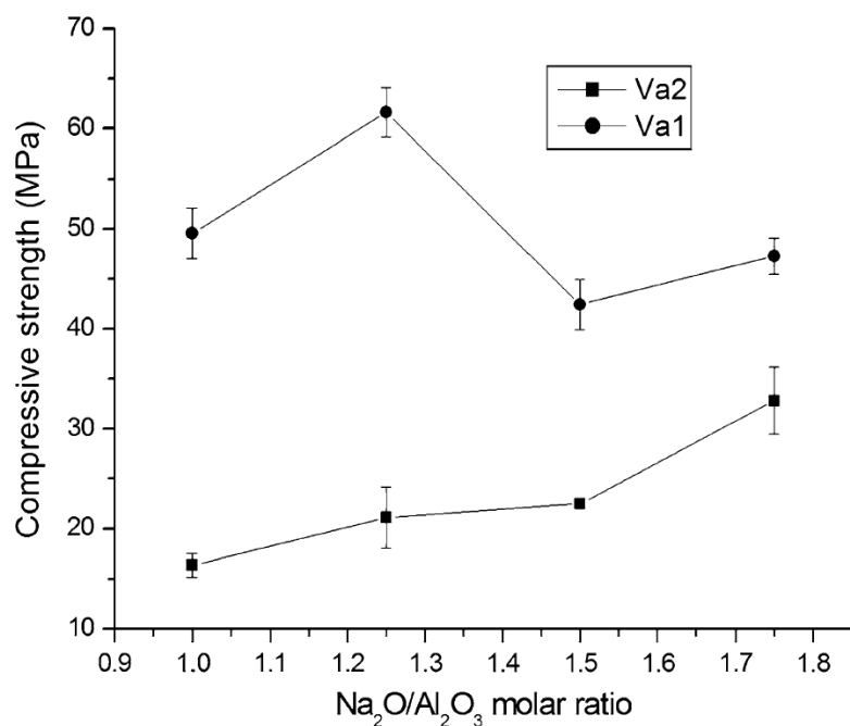
Figura 28: Efeito da composição molar nas resistências à compressão das cinzas ativadas por álcalis.
