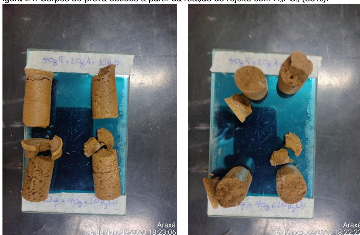
Figura 24: Corpos de prova obtidos a partir da reação do rejeito com \text{H}_3\text{PO}_4 (85%).
