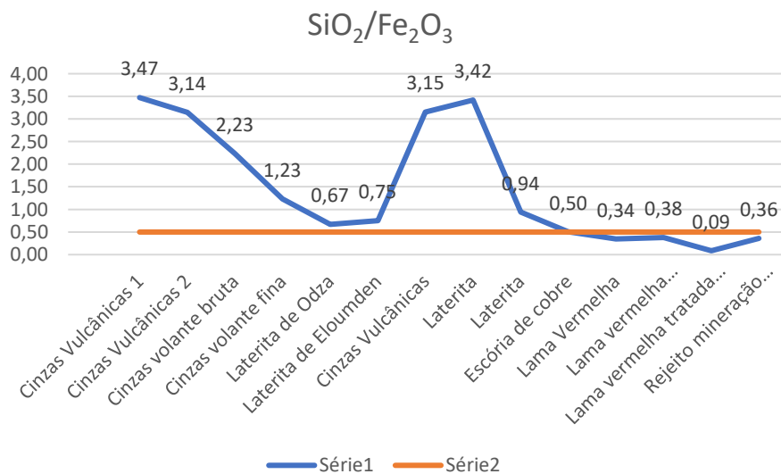
Figura 19: Relação entre a razão \text{SiO}_2/\text{Fe}_2\text{O}_3 e ativadores usados.
