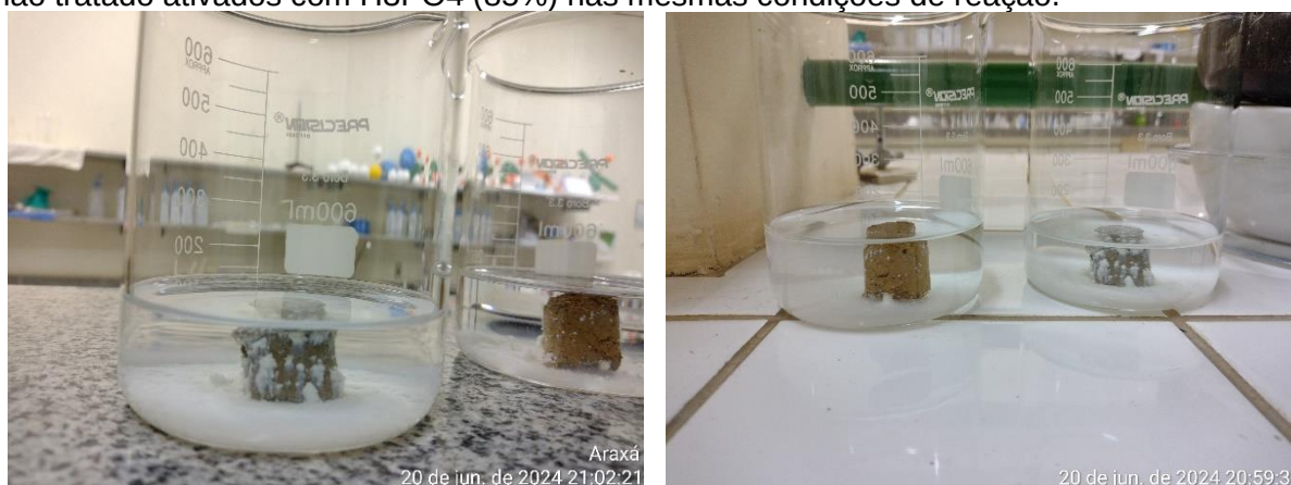
Figura 26: Teste de absorção de água com corpos de prova moldados com rejeito tratado e não tratado ativados com H 3 PO 4 (85%) nas mesmas condições de reação.
