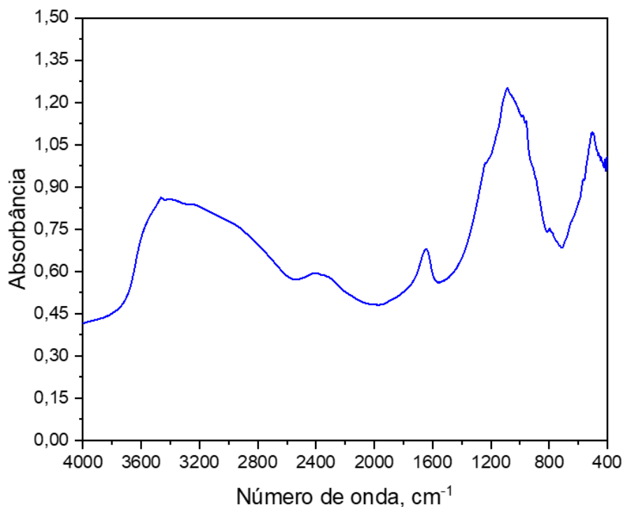
Figura 33: Espectro de FTIR para amostra de geopolímero.
