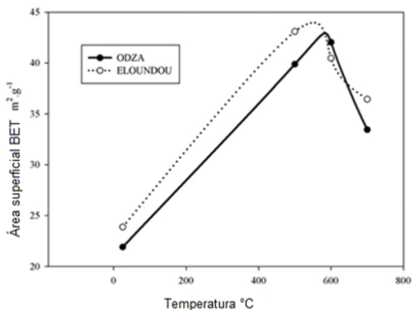
Figura 10: Efeito do aquecimento na área de superfície de amostras de lateritas de Odza e Elounden.
