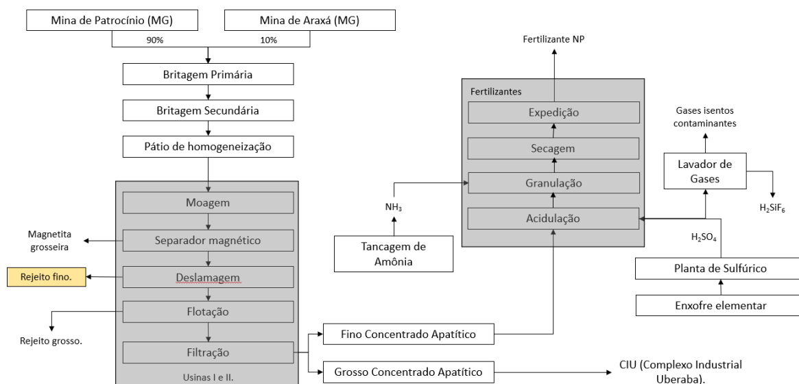
Figura 11: Fluxograma de processo.
