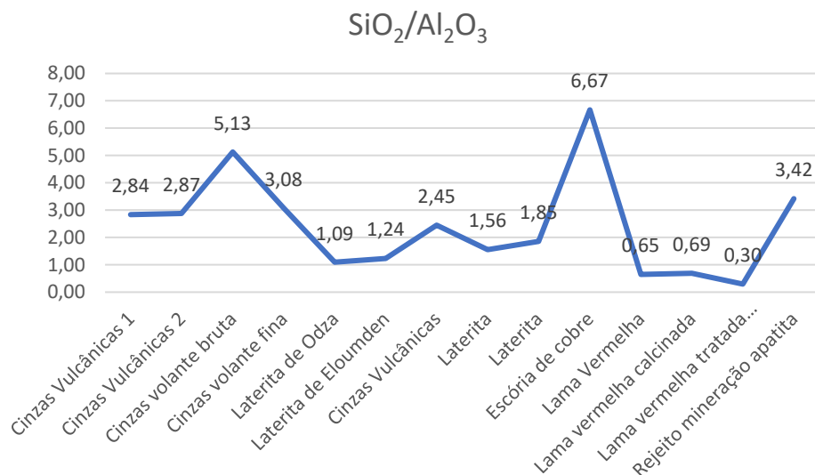
Figura 17: Relação entre a razão \text{SiO}_2/\text{Al}_2\text{O}_3 e ativadores usados.
