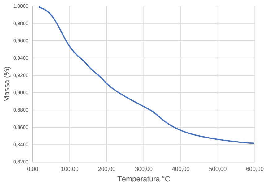
Figura 31: Análise termogravimétrica geopolímero 7 dias cura a temperatura ambiente.
