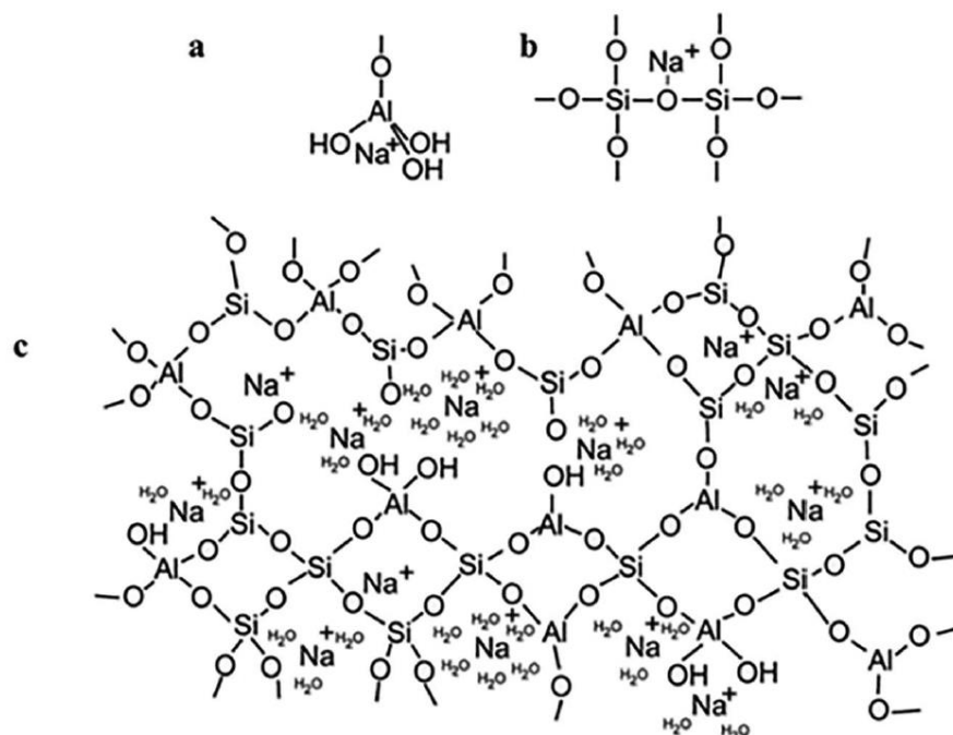
Figura 8: (a) Modelo proposto para a localização do cátion \text{Na}^+ de balanceamento de carga que assume a forma de uma espécie de aluminato de Na semi-anexado; (b) modelo proposto para a localização do cátion \text{Na}^+ de balanceamento de carga que assume a forma de uma rede de ponte modificada; (c) modelo esquemático proposto para estrutura de geopolímero ativado por álcali com base em um modelo original.
