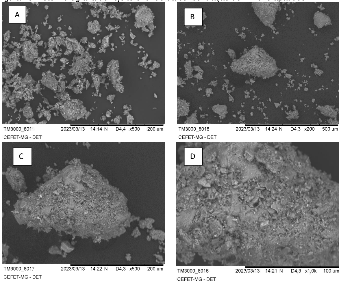
Figura 23: Fotomicrografia do rejeito oriundo da concentração do minério apatítico.
