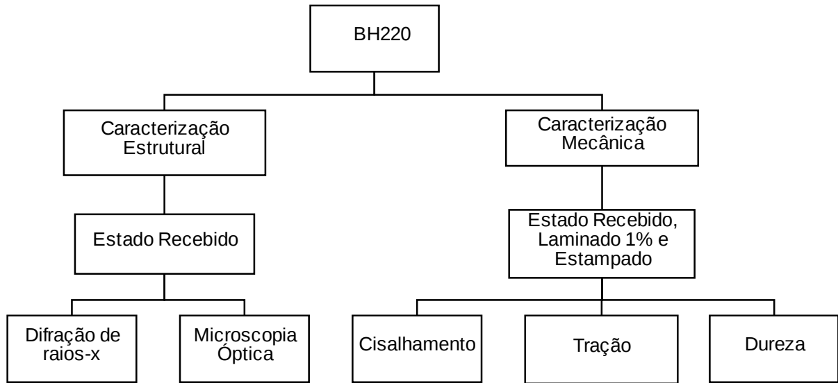
Figura 37 - Fluxograma caracterização aço BH220
