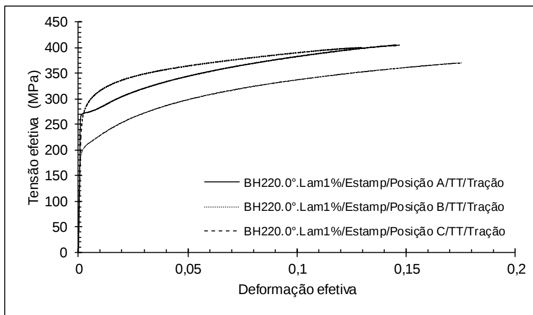
Figura 65 - Curva tensão x deformação em tração aço BH220 a 0° para diferentes posições do produto estampado/tratado termicamente
