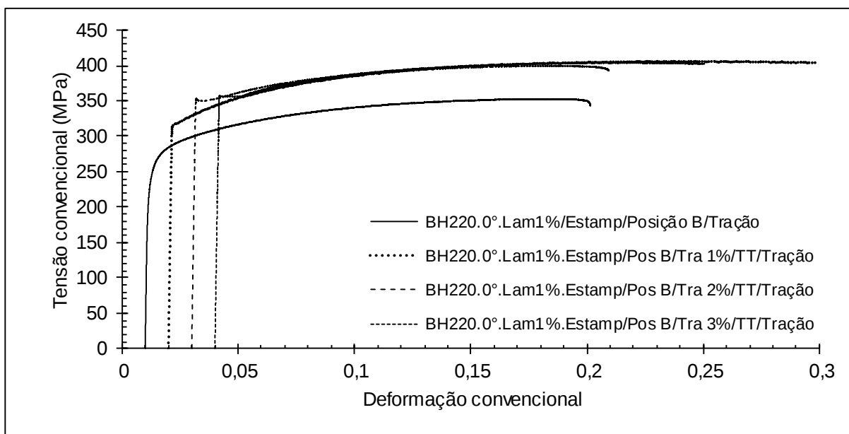
Figura 73 - Curvas de fluxo aço BH220 0° para diversos valores de pré-deformação em tração no produto estampado - região B
