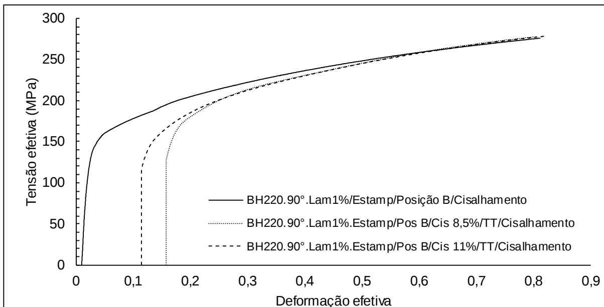
Figura 81 - Curvas de fluxo aço BH220 90° para diversos valores de pré-deformação em cisalhamento no produto estampado - região B
