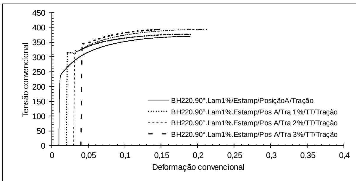
Figura 75 - Curvas de fluxo aço BH220 90° para diversos valores de pré-deformação em tração no produto estampado - região A
