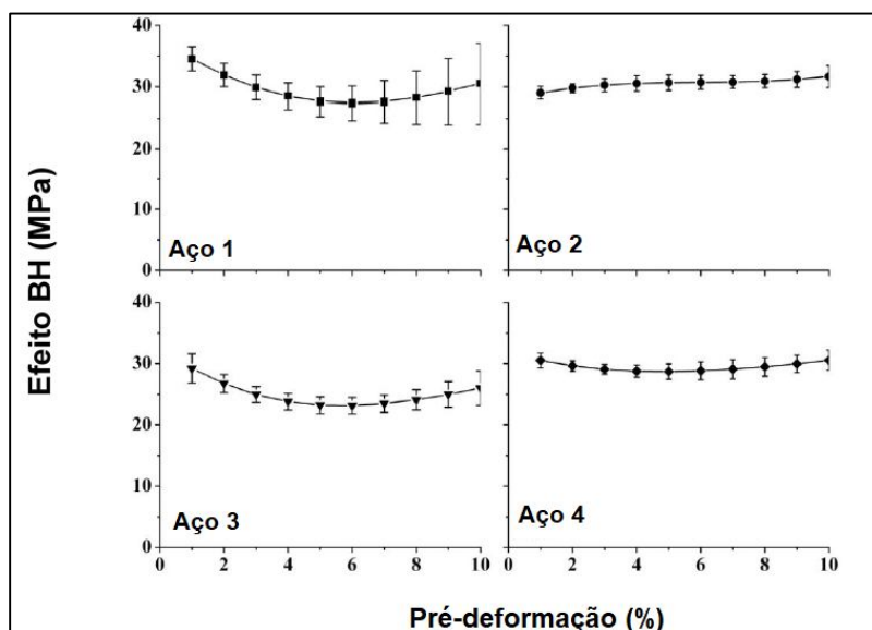
Figura 11 - Efeito calculado da pré-deformação no efeito BH de diferentes aços
